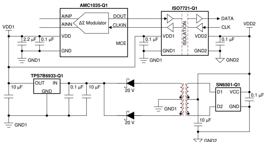
图 49. Galvanic Isolation of the AMC1035-Q1
