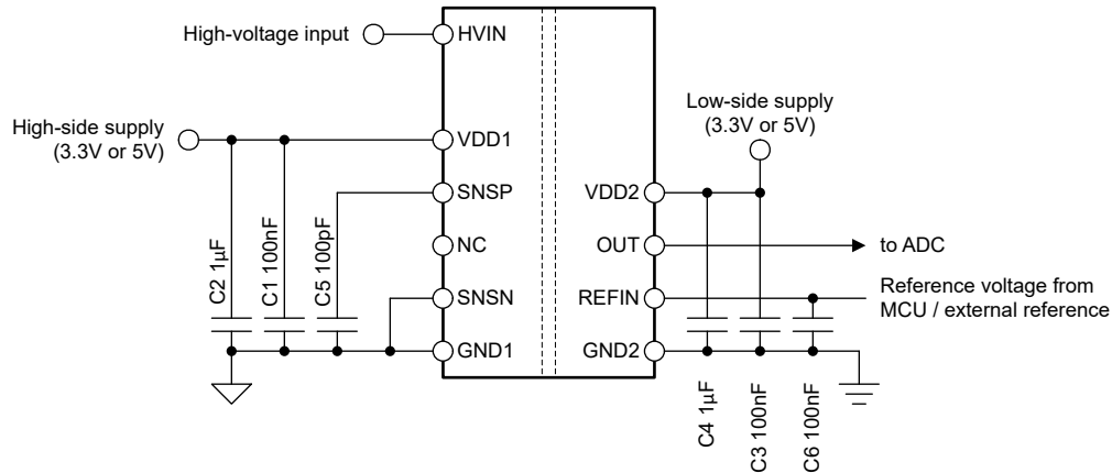
图 8-5. AMC0381R-Q1 去耦
