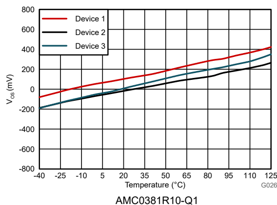
图 6-15. 输入失调电压与温度间的关系
