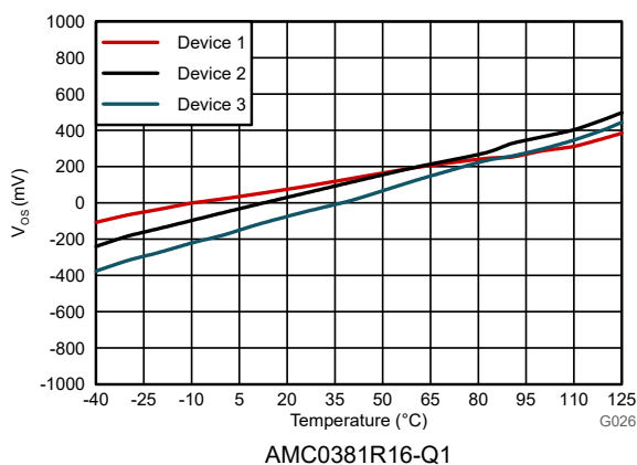
图 6-16. 输入失调电压与温度间的关系
