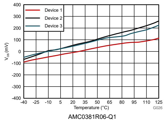
图 6-14. 输入失调电压与温度间的关系
