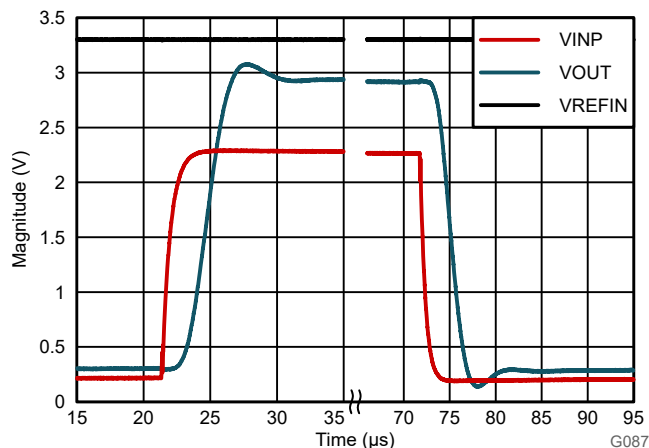
图 8-4. AMC0381R 的阶跃响应
