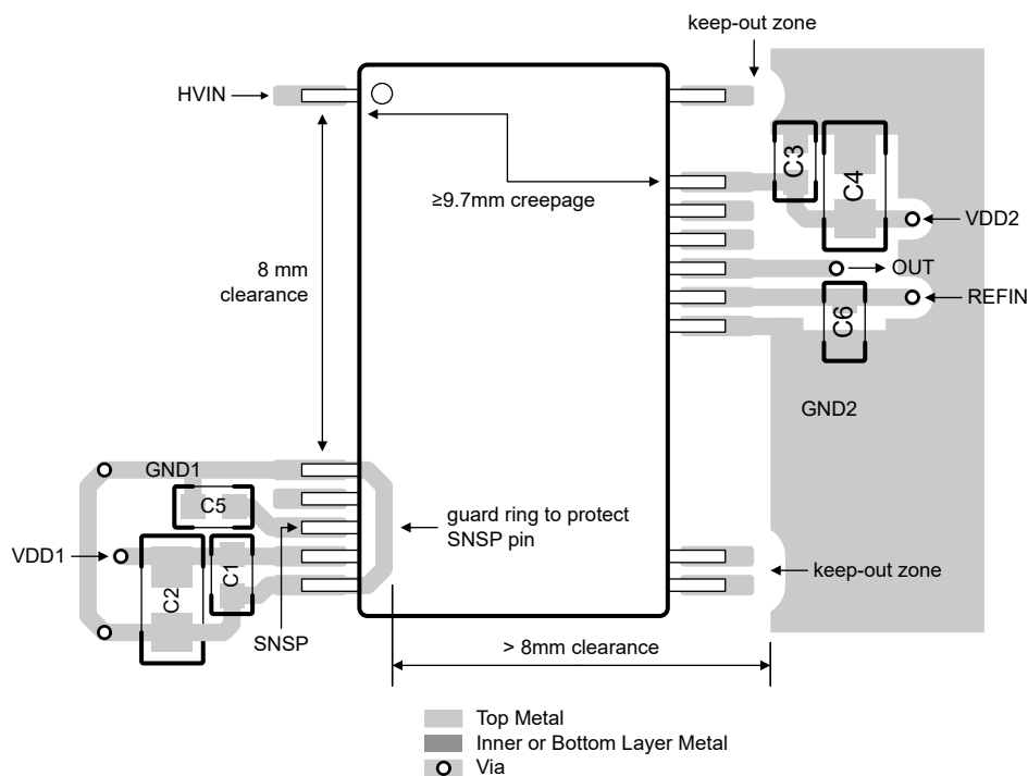
图 8-6. AMC0381R 的建议布局
