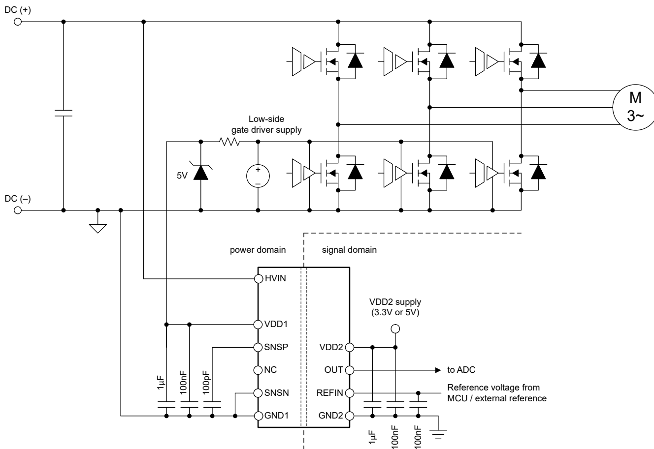
图 8-1. 在典型应用中使用 AMC0381R
