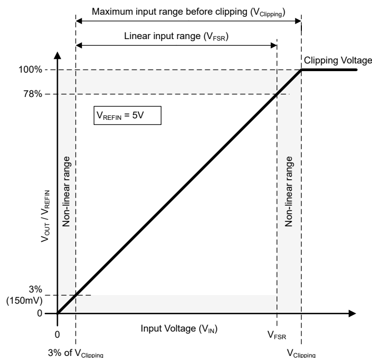
图 7-2. AMC0381R 的输入到输出传送曲线
