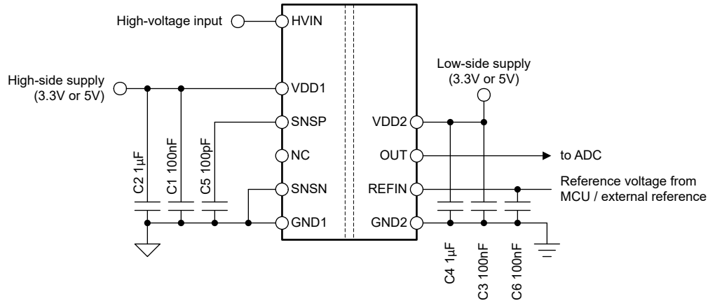
图 8-5. AMC0381R 去耦
