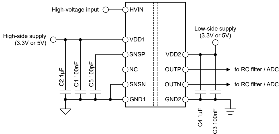
图 8-5. AMC0381D-Q1 去耦
