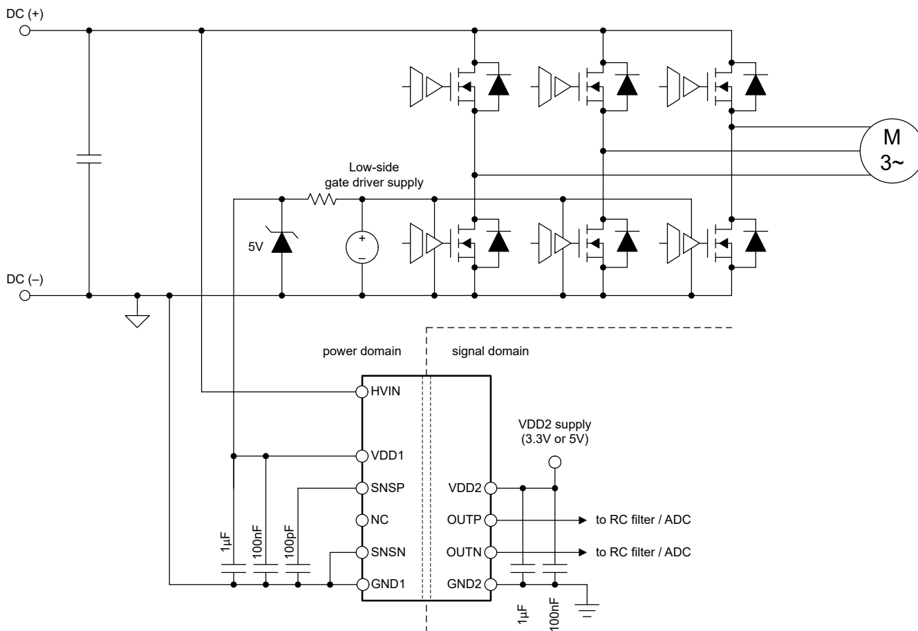
图 8-1. 在典型应用中使用 AMC0381D-Q1
