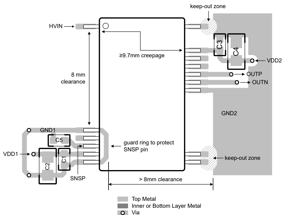
图 8-6. AMC0381D-Q1 的建议布局
