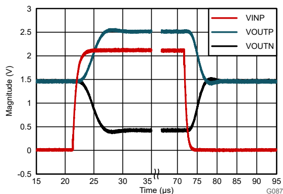
图 8-4. AMC0381D-Q1 的阶跃响应
