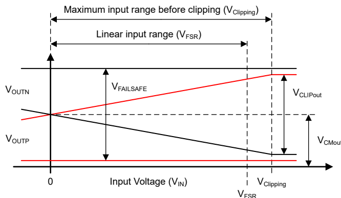
图 7-2. AMC0381D-Q1 的输入到输出传递曲线
