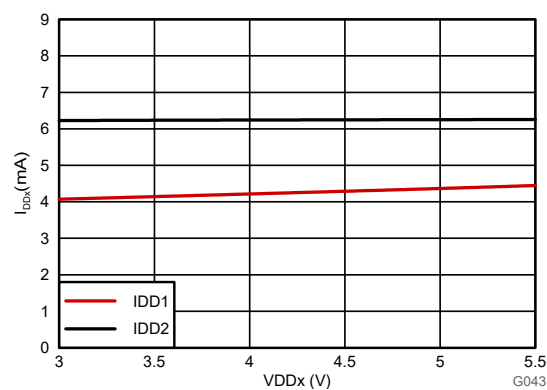
图 6-18. 电源电流与电源电压间的关系
