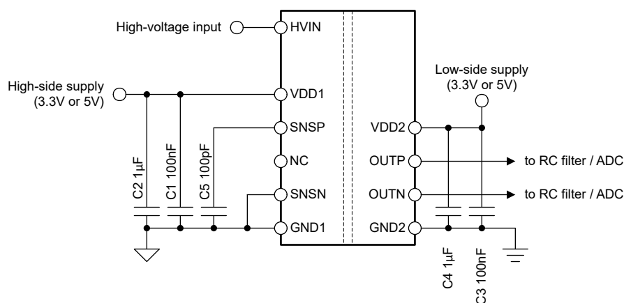
图 8-5. AMC0380D 去耦
