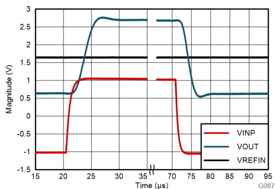
图 8-4. AMC0x30S 的阶跃响应
