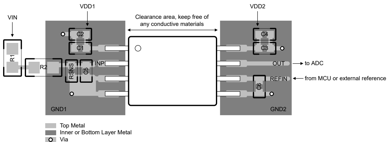
图 8-6. AMC0x30S 的建议布局
