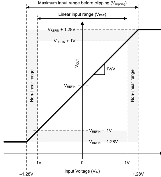
图 7-2. AMC0x30S 的输入到输出传送曲线
