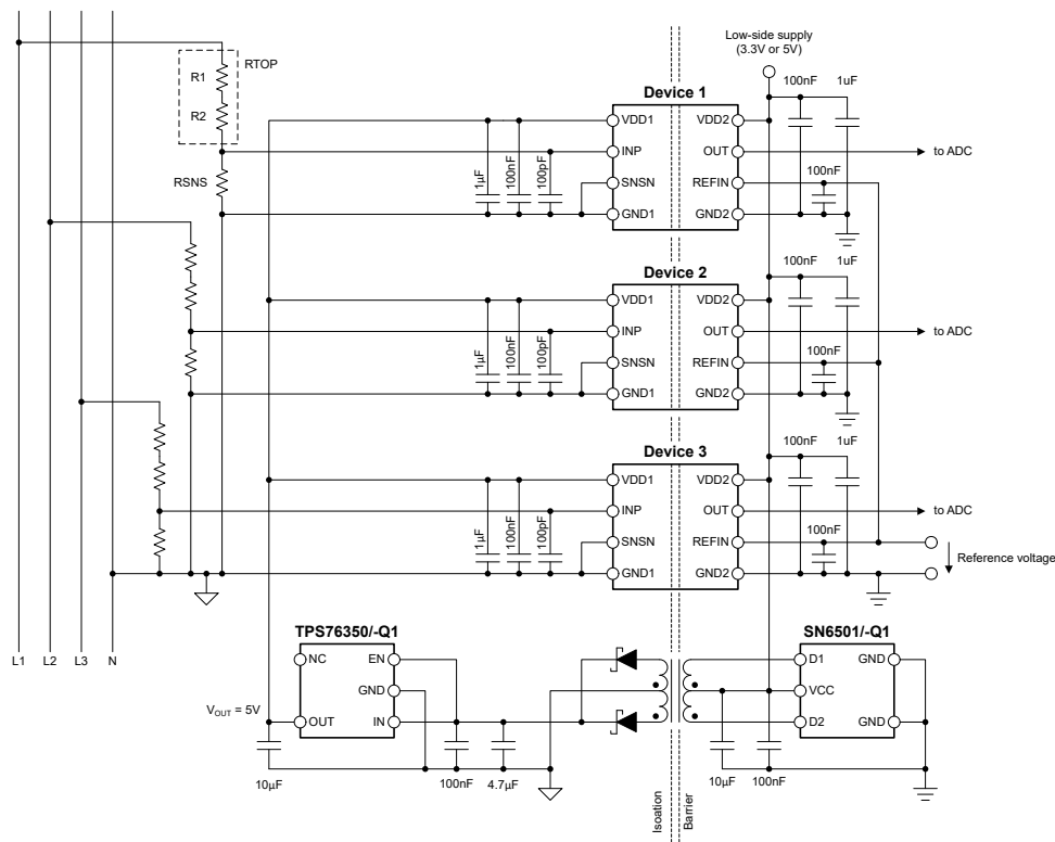
图 8-1. 在典型应用中使用 AMC0x30R-Q1
