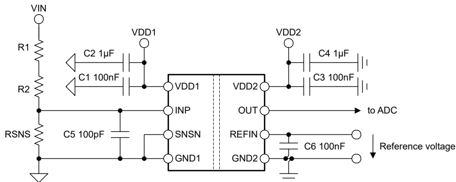
图 8-5. AMC0x30R-Q1 去耦
