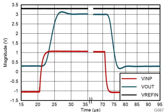
图 8-4. AMC0x30R-Q1 的阶跃响应
