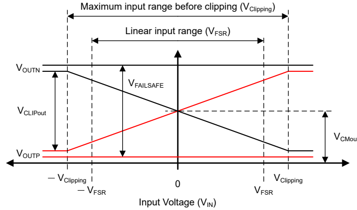
图 7-2. AMC0x30D 的输入到输出传递曲线
