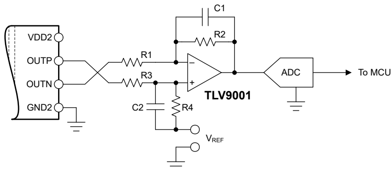
图 8-3. 将 AMC0x30D 输出连接到单端输入 ADC
