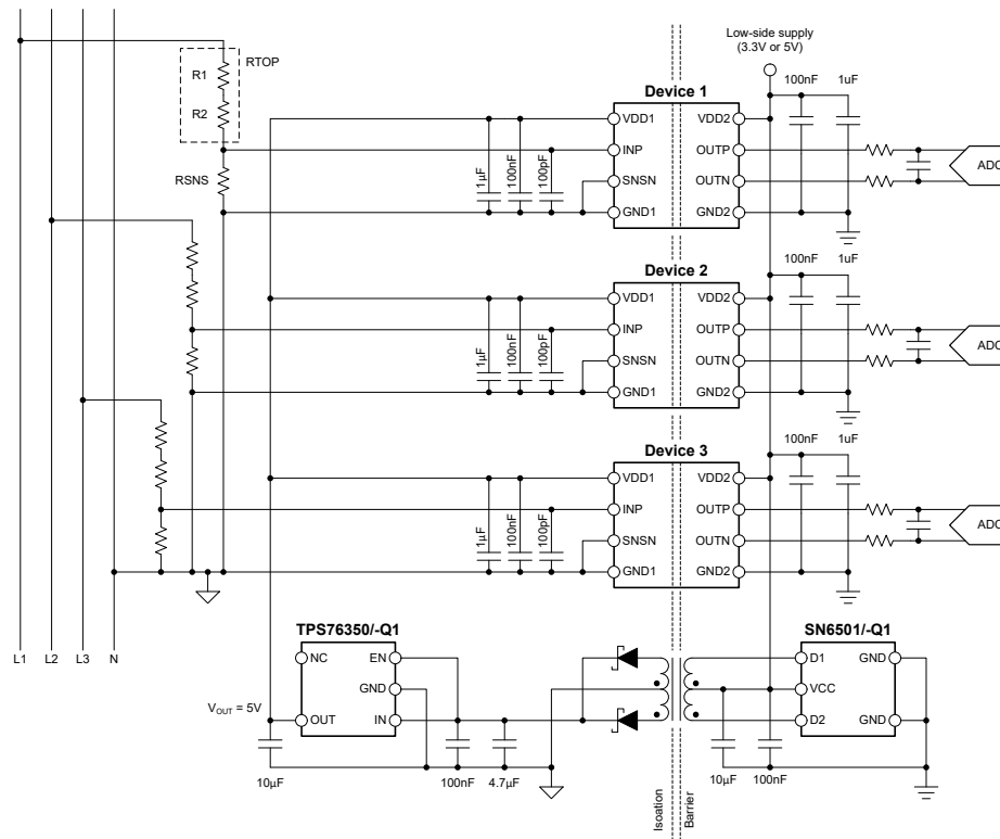
图 8-1. 在典型应用中使用 AMC0x30D
