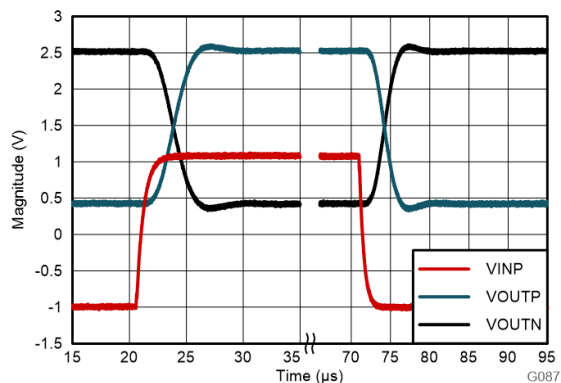
图 8-4. AMC0x30D 的阶跃响应
