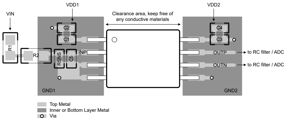
图 8-6. AMC0x30D 的建议布局
