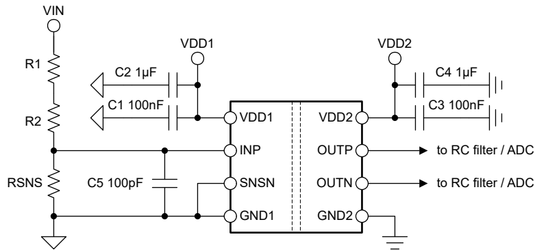
图 8-5. AMC0x30D 去耦
