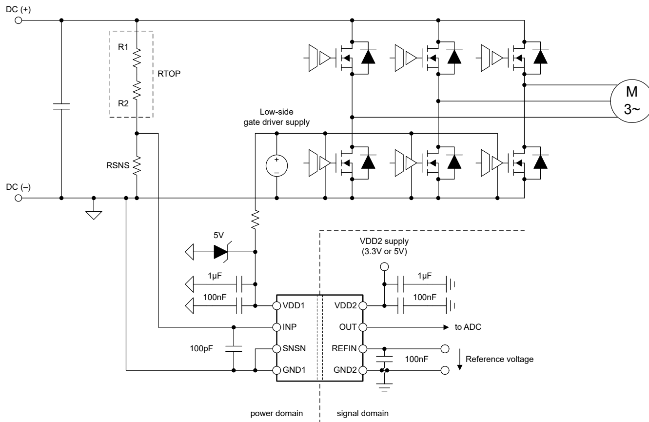
图 8-1. 在典型应用中使用 AMC0x11S
