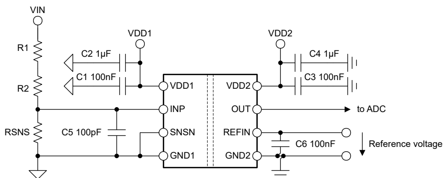
图 8-5. AMC0x11S 去耦
