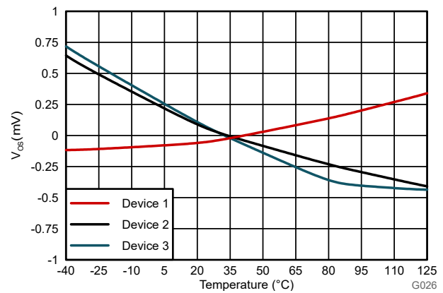
图 6-6. 输入失调电压与温度间的关系
