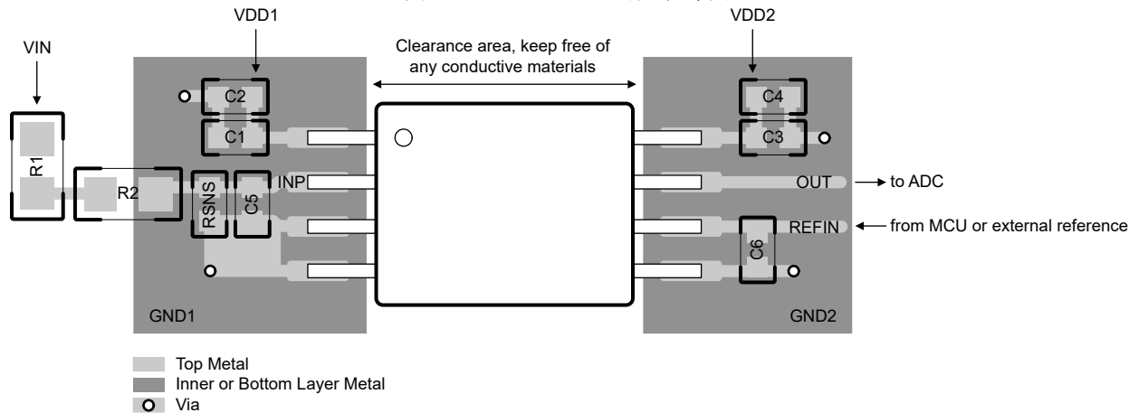
图 8-6. AMC0x11S 的建议布局
