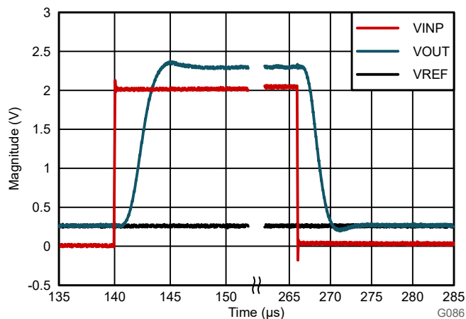
图 8-4. AMC0x11S 的阶跃响应
