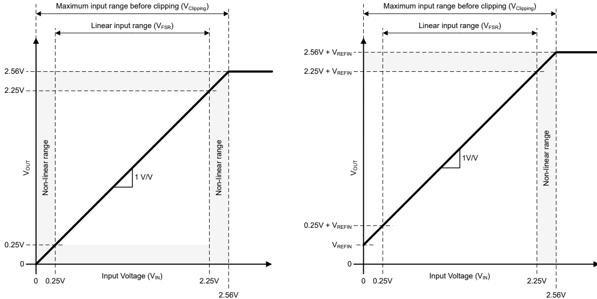
图 7-2. AMC0x11S 的输入到输出传递曲线 左：REFIN 短接至 GND2。右： V_{\text{REFIN}} = 250\text{mV}
