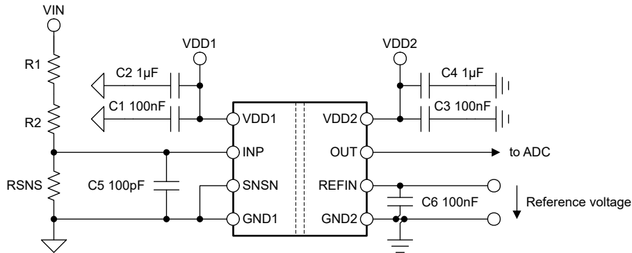
图 8-5. AMC0x11R-Q1 去耦
