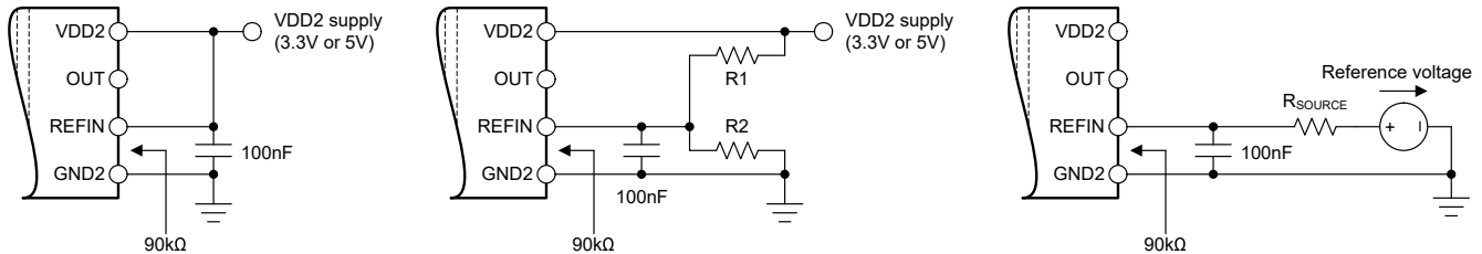
图 8-3. 连接 REFIN 引脚
