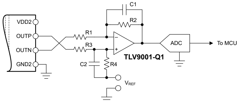
图 8-3. 将 AMC0x11D-Q1 输出连接到单端输入 ADC
