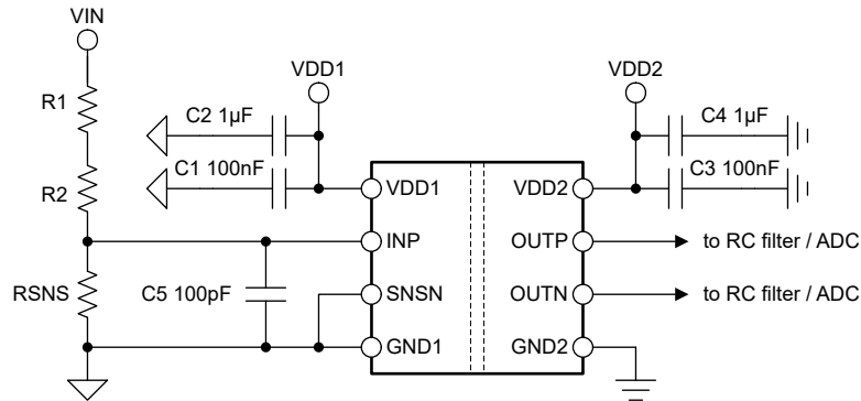
图 8-5. AMC0x11D-Q1 去耦
