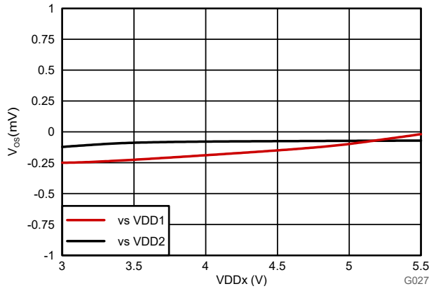
图 6-5. 输入失调电压与电源电压间的关系
