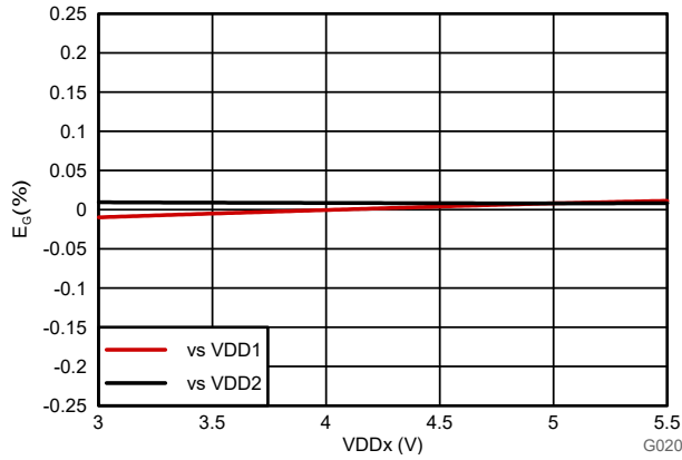
图 6-7. 增益误差与电源电压间的关系
