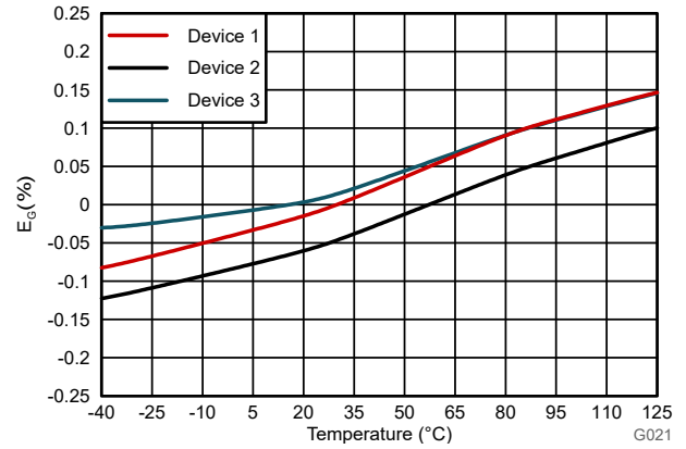
图 6-8. 增益误差与温度间的关系
