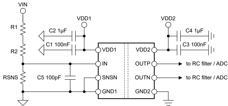
图 8-5. AMC0x11D 去耦
