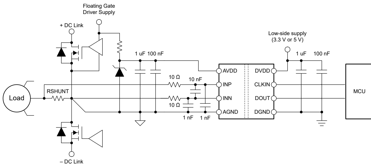
图 8-1. 在典型应用中使用 AMC0x06M25 进行电流检测
