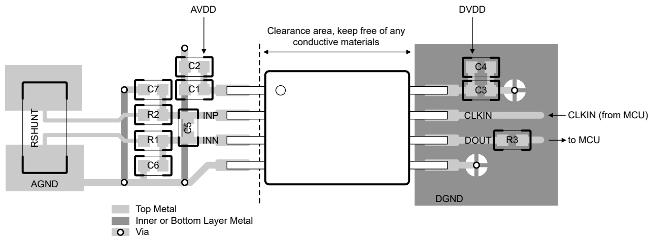
图 8-5. AMC0x06M25 的建议布局
