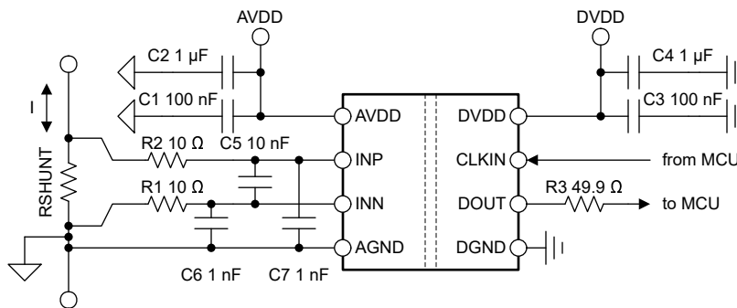
图 8-4. AMC0x06M25 去耦
