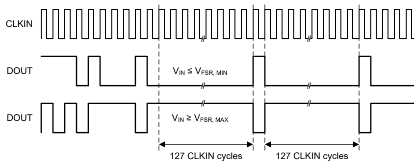
图 7-6. AMC0x06M25 的满量程输出
