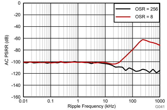
图 6-20. 电源抑制比与纹波频率间的关系
