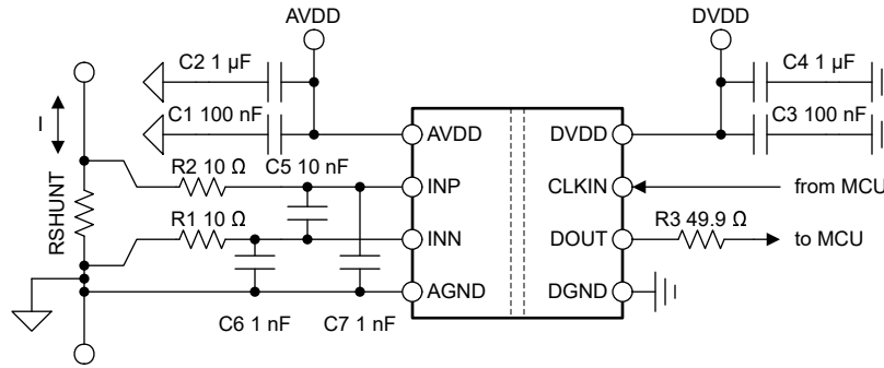
图 8-4. AMC0x06M05-Q1 去耦
