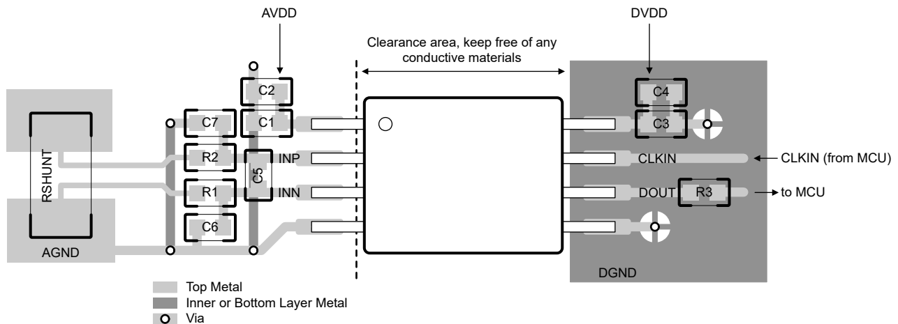
图 8-5. AMC0x06M05-Q1 的建议布局
