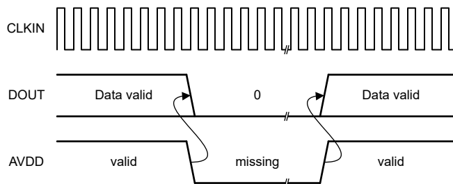
图 7-7. 高侧电源缺失情况下 AMC0x06M05-Q1 的输出
