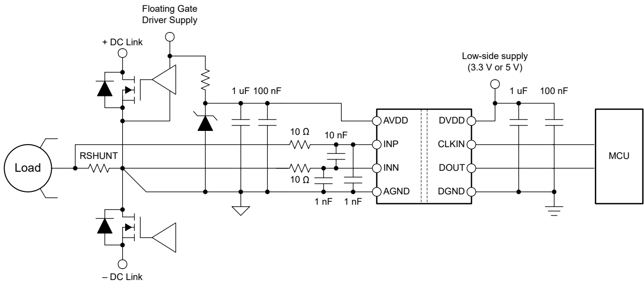
图 8-1. 在典型应用中使用 AMC0x06M05-Q1 进行电流检测
