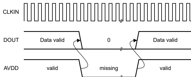
图 7-7. 高侧电源缺失情况下 AMC0x06M05 的输出
