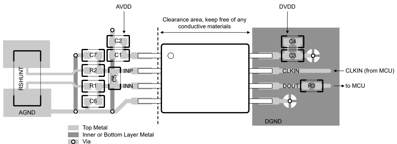
图 8-5. AMC0x06M05 的建议布局
