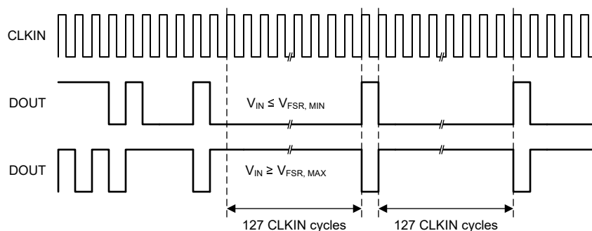
图 7-6. AMC0x06M05 的满量程输出
