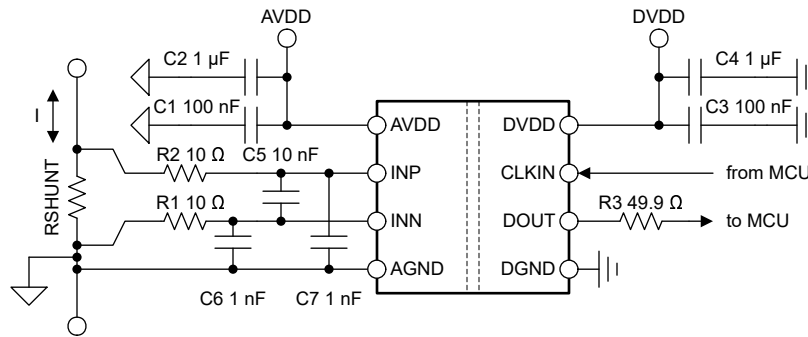
图 8-4. AMC0x06M05 去耦
