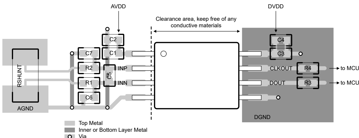
图 8-5. AMC0x03M2510 的建议布局
