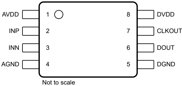
图 5-1. DWV 和 D 封装，8 引脚 SOIC（顶视图）
