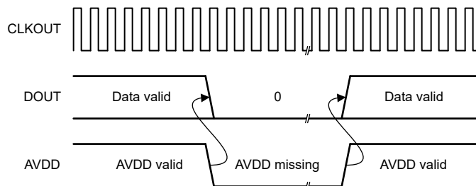
图 7-7. 高侧电源缺失情况下 AMC0x03M2510 的输出
