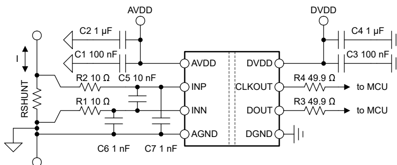
图 8-4. AMC0x03M2510 去耦
