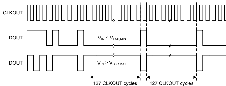
图 7-6. AMC0x03M2510 的满量程输出
