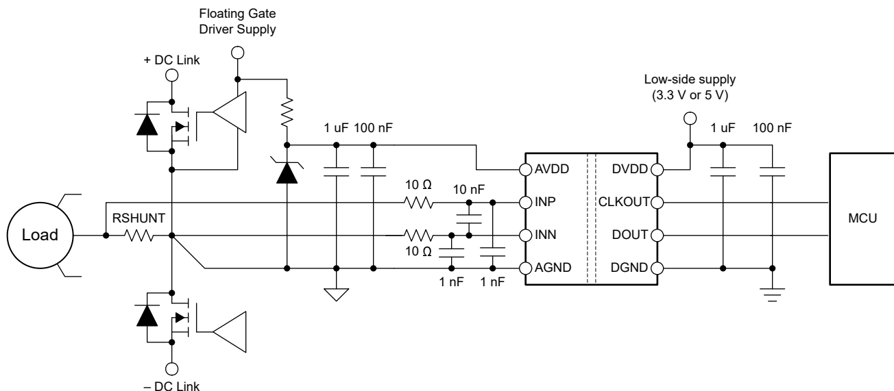
图 8-1. 在典型应用中使用 AMC0x03M2510 进行电流检测
