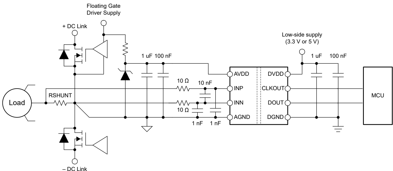
图 8-1. 在典型应用中使用 AMC0x03M0510 进行电流检测
