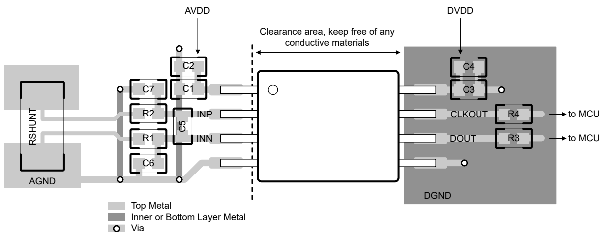
图 8-5. AMC0x03M0510 的建议布局
