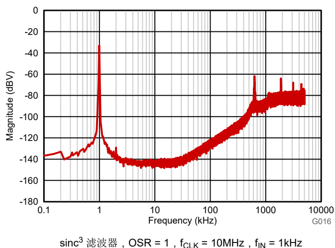
图 7-3. 量化噪声整形
