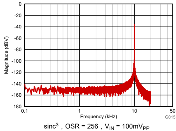
图 6-25. 10kHz 输入信号时的频谱
