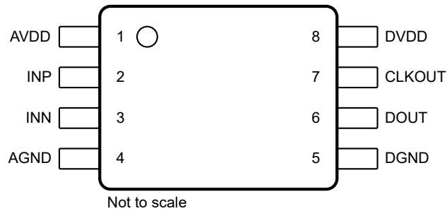
图 5-1. DWV 和 D 封装，8 引脚 SOIC（顶视图）
