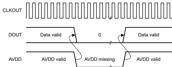
图 7-7. 高侧电源缺失情况下 AMC0x03M0510 的输出
