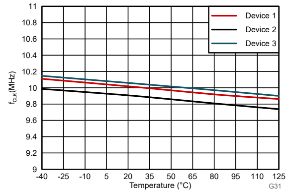
图 6-26. 内部时钟频率与温度间的关系
