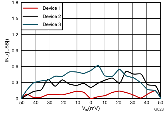
图 6-14. 积分非线性与输入电压间的关系
