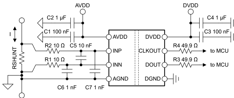
图 8-4. AMC0x03M0510 去耦
