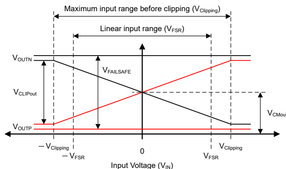
图 7-2. AMC0x00D-Q1 的输入到输出传递曲线
