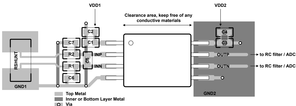
图 8-6. AMC0x00D-Q1 的建议布局
