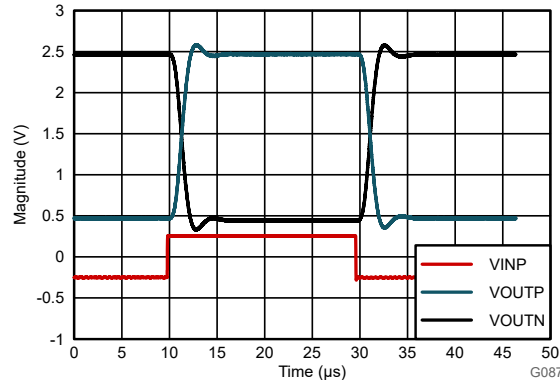
图 8-4. AMC0x00D-Q1 的阶跃响应
