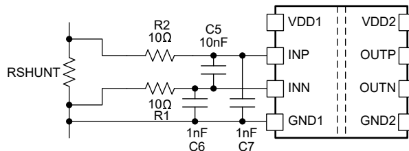
图 8-2. 输入滤波器
