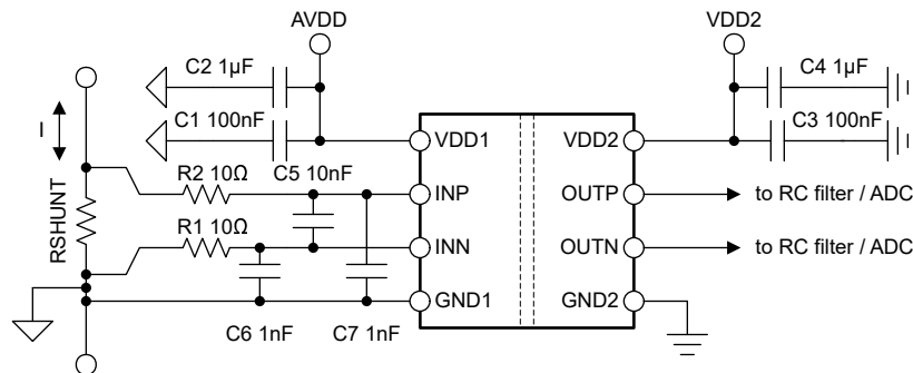
图 8-5. AMC0x00D-Q1 去耦
