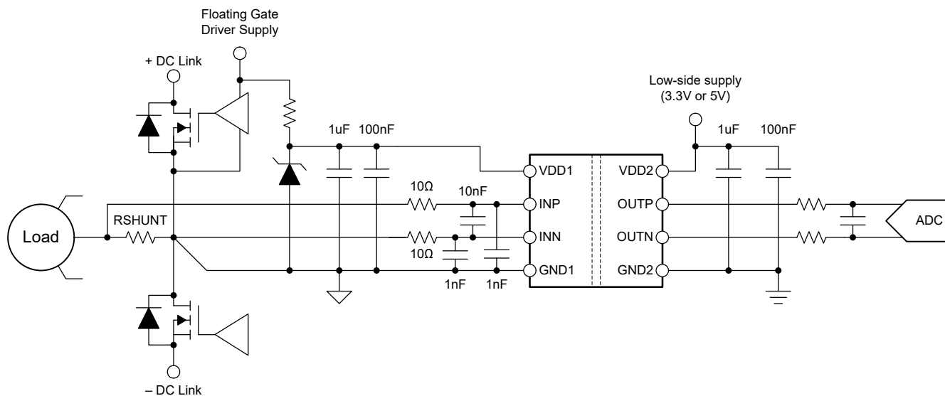
图 8-1. 在典型应用中使用 AMC0x00D-Q1 进行电流检测
