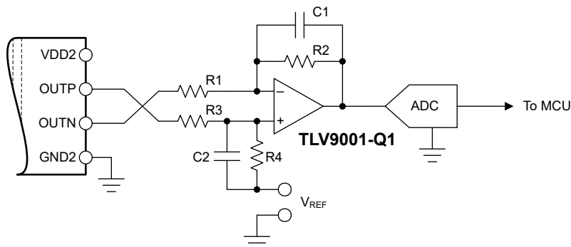
图 8-3. 将 AMC0x00D-Q1 输出连接到单端输入 ADC
