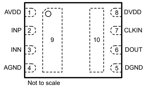
图 4-1. DEN 封装，8 引脚 VSON（顶视图）
