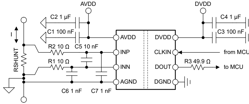
图 7-3. AMC0106M25 去耦
