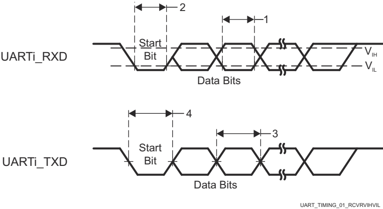
图 6-115. UART 时序
