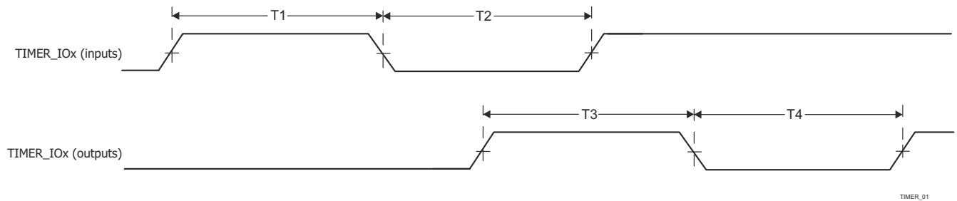
图 6-114. 计时器时序
