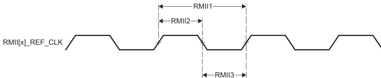
图 6-36. CPSW2G RMII[x]_REFCLK 时序要求 - RMII 模式
