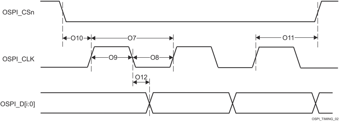
图 6-102. OSPI0/1 开关特性 - PHY SDR 数据训练
