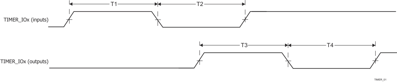
图 6-111. 计时器时序
