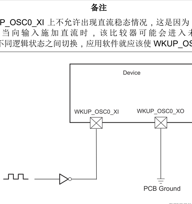
图 6-27. 1.8V LVCMOS 兼容时钟输入
