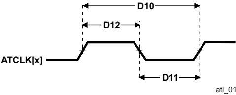
图 6-34. ATCLK[x] 时序
