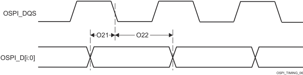
图 6-103. OSPI 时序要求 - SDR，外部环回时钟
