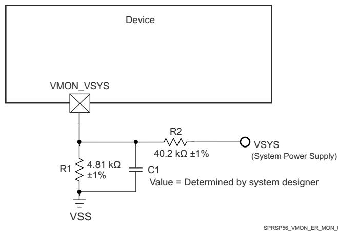
图 8-5. 系统电源监测分压器电路
