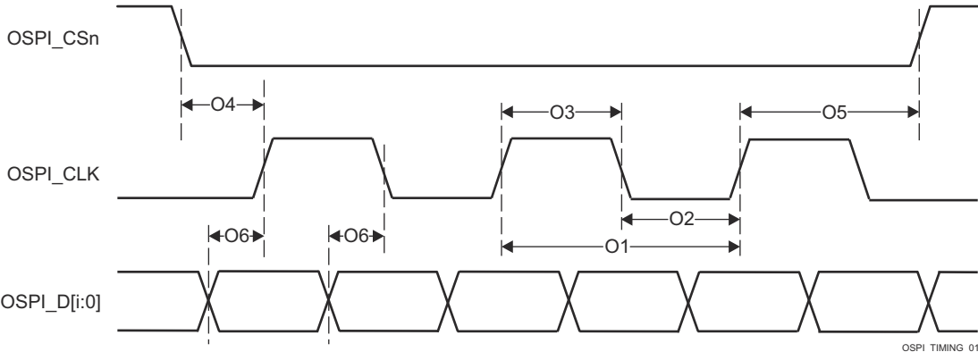
图 6-113. OSPI0/1 开关特性 - Tap DDR，无环回
