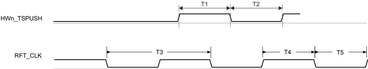
图 6-100. CPTS 时序要求
