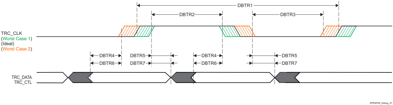
图 6-113. 布线开关特性
