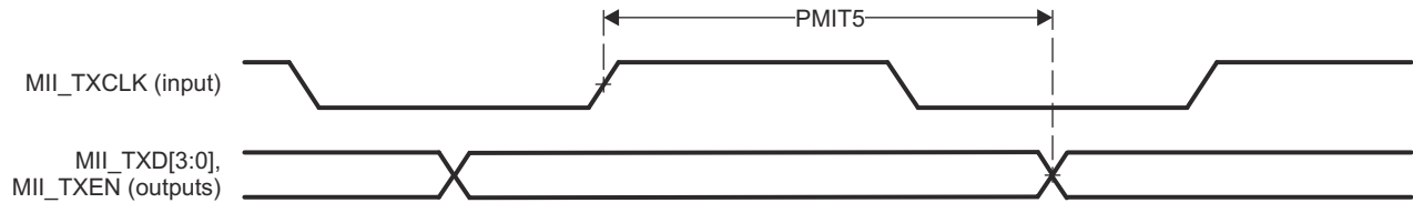
图 6-121. PRU_ICSSG MII_TXD[3:0], MII_TXEN Timing
