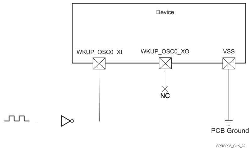
图 6-17. 1.8-V LVC MOS-Compatible Clock Input
