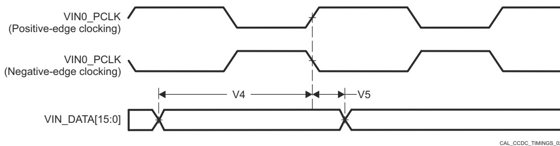
图 6-31. LVDSRX Input Timings
