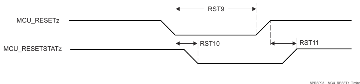
图 6-8. MCU_RESETz and MCU_RESETSTATz Timing
