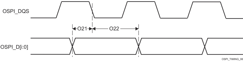
图 7-98. OSPI0 时序要求 - 具有外部电路板环回的 PHY SDR
