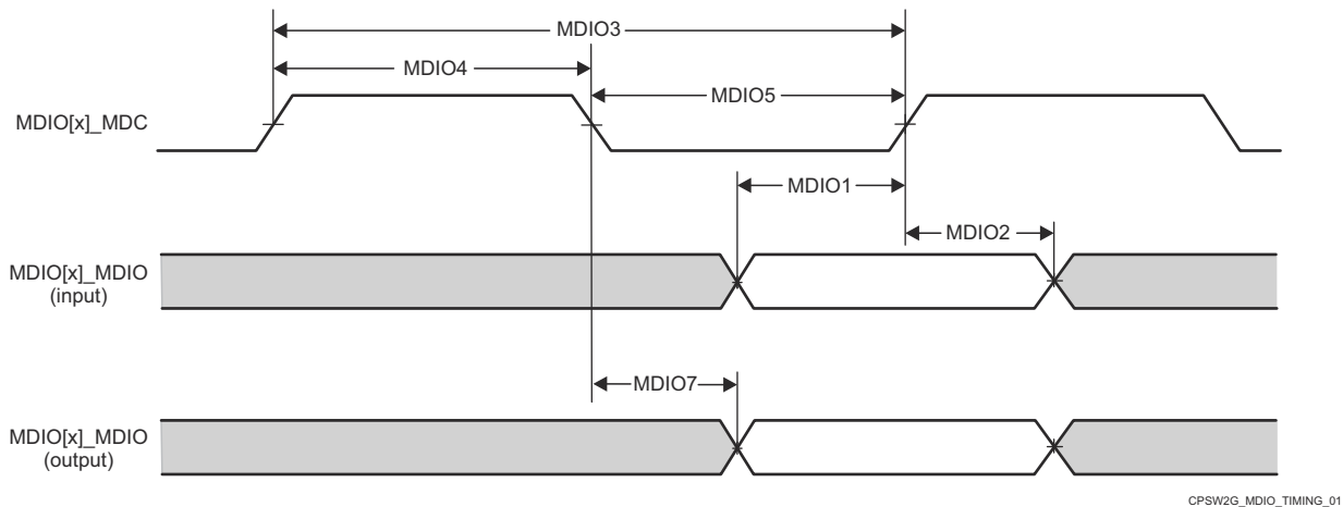
图 7-26. CPSW3G MDIO 时序要求和开关特性
