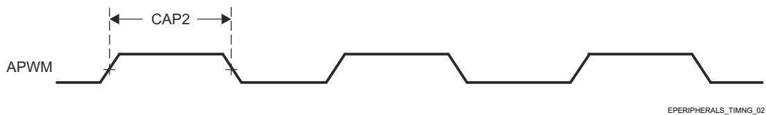
图 7-38. ECAP 开关特性
