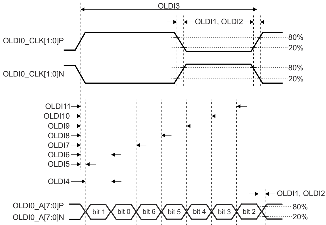
图 7-94. OLDI0 开关特性
