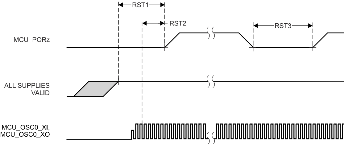
图 7-7. MCU_PORz 时序要求
