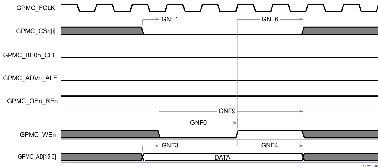
图 7-60. GPMC 和 NAND 闪存 - 数据写入周期
