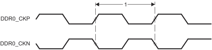
图 7-34. DDRSS 开关特性
