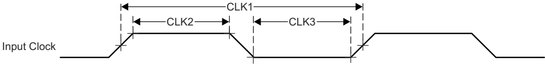
图 7-14. 时钟时序要求
