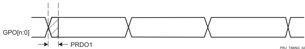
图 7-106. PRUSS PRU 直接输出时序
