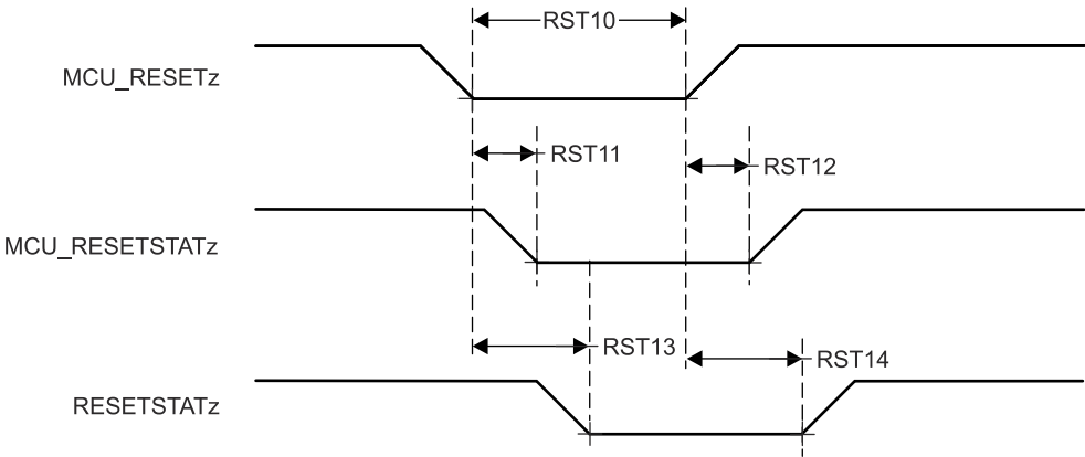
图 7-9. MCU_RESETz、MCU_RESETSTATz 和 RESETSTATz 时序要求和开关特性
