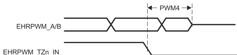
图 7-44. EHRPWM_TZn_IN 至 EHRPWM_A/B 高阻态开关特性
