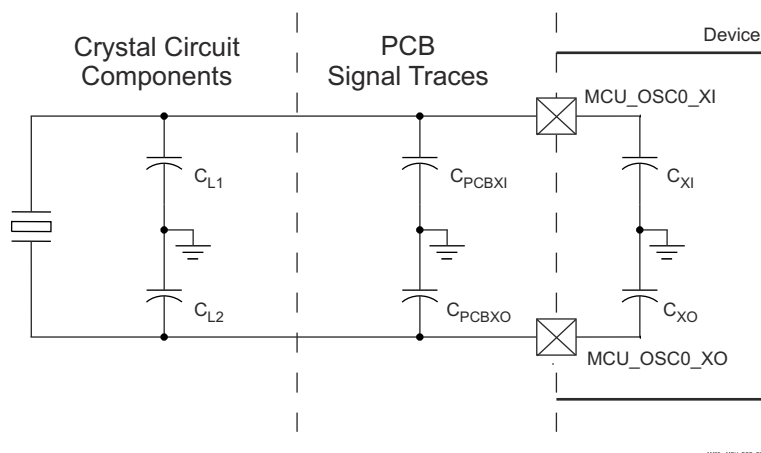
图 7-18. 负载电容
