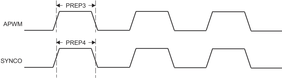
图 7-114. PRUSS ECAP 开关特性
