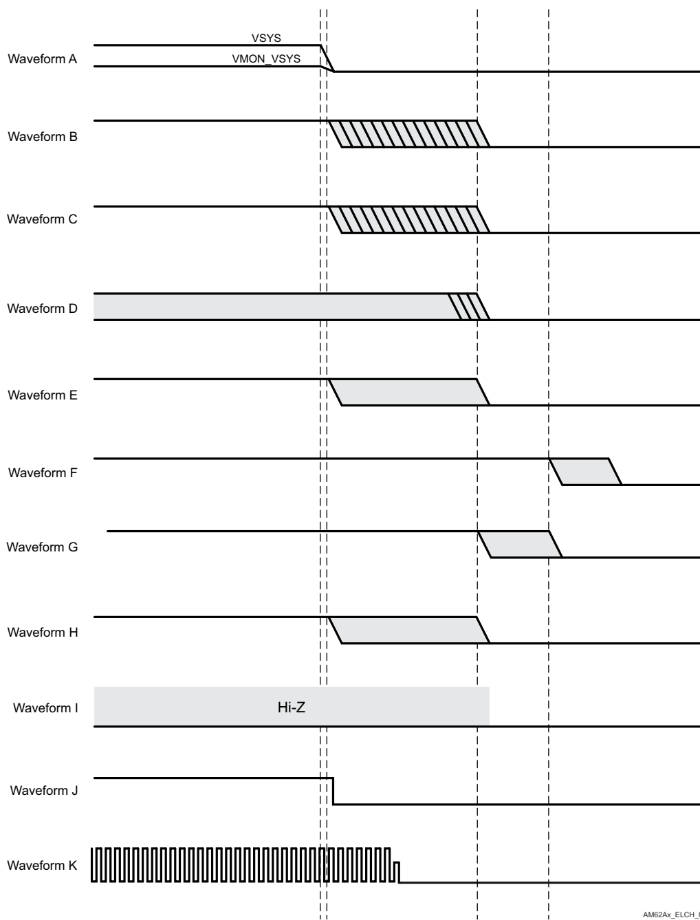
图 7-6. 下电时序
