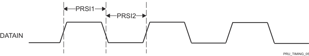
图 7-109. PRUSS PRU 移入时序
