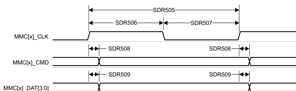
图 7-80. MMC0 - UHS-I SDR50 - 发送模式
