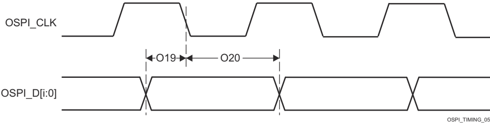
图 7-97. OSPI0 时序要求 - 具有内部 PHY 环回的 PHY SDR
