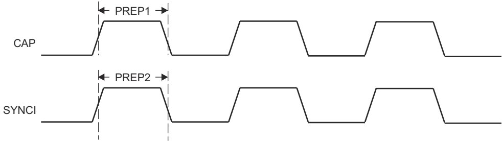
图 7-113. PRUSS ECAP 时序
