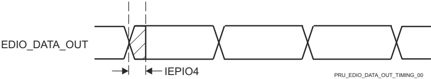
图 7-111. PRUSS IEP 数字 IO 时序要求
