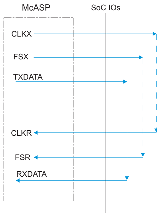
图 7-43. McASP1-8 COIFIO – ASYNC Mode
