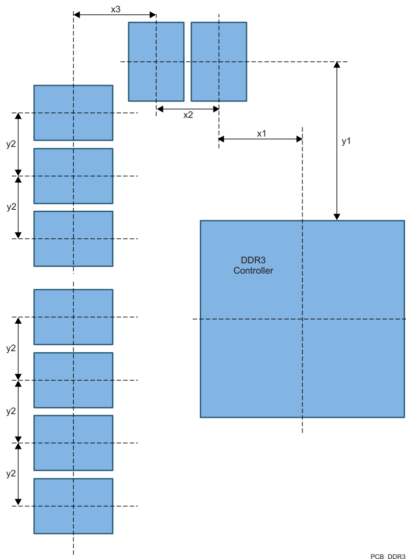
图 8-4. Placement Specifications
