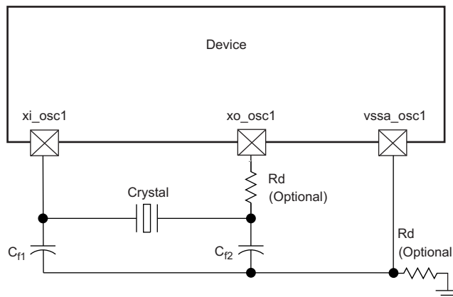
图 6-6. Crystal Implementation
