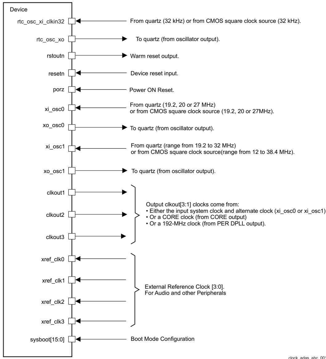
图 6-1. Clock Interface
