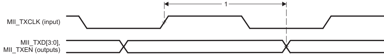
图 7-107. PRU-ICSS MII_TXD[3:0], MII_TXEN Timing
