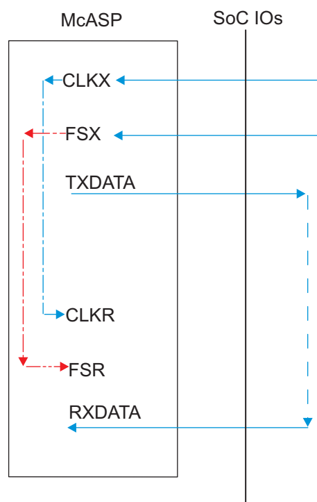
图 7-49. McASP1-8 CI-FI- – SYNC Mode
