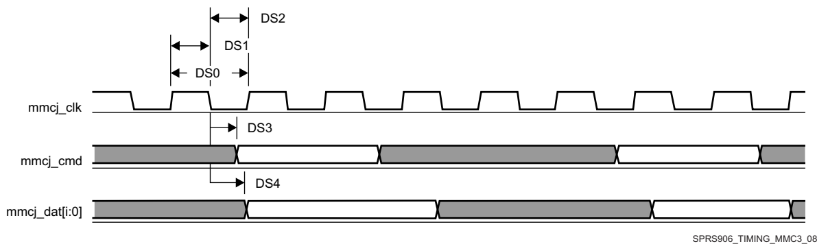
图 7-82. MMC/SD/SDIOj in - Default Speed - Transmitter Mode
