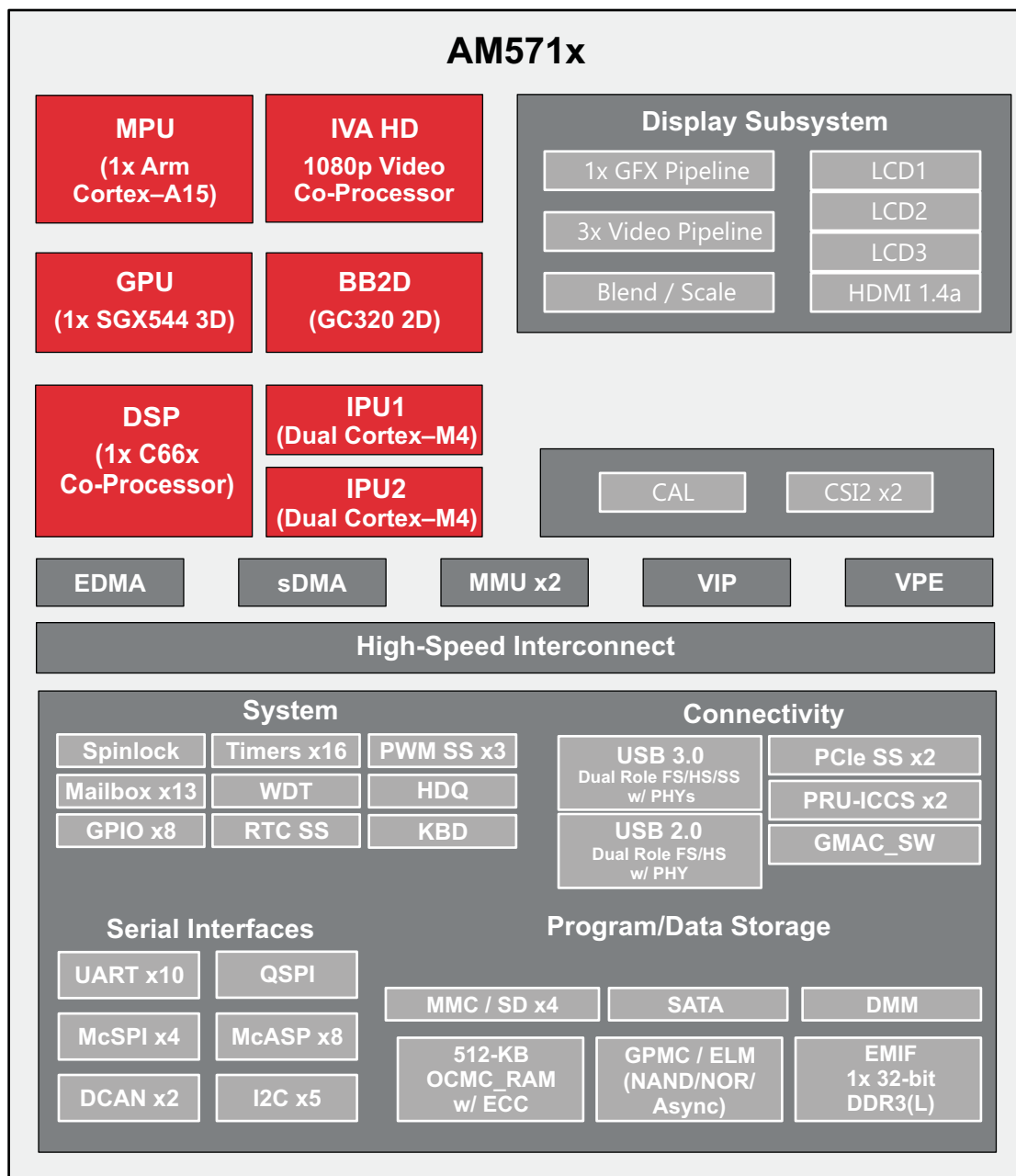
图 1-1. AM571x 框图
