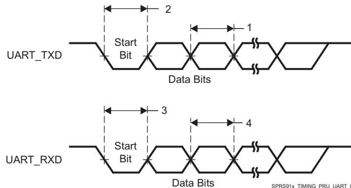
图 7-111. PRU-ICSS UART Timing
