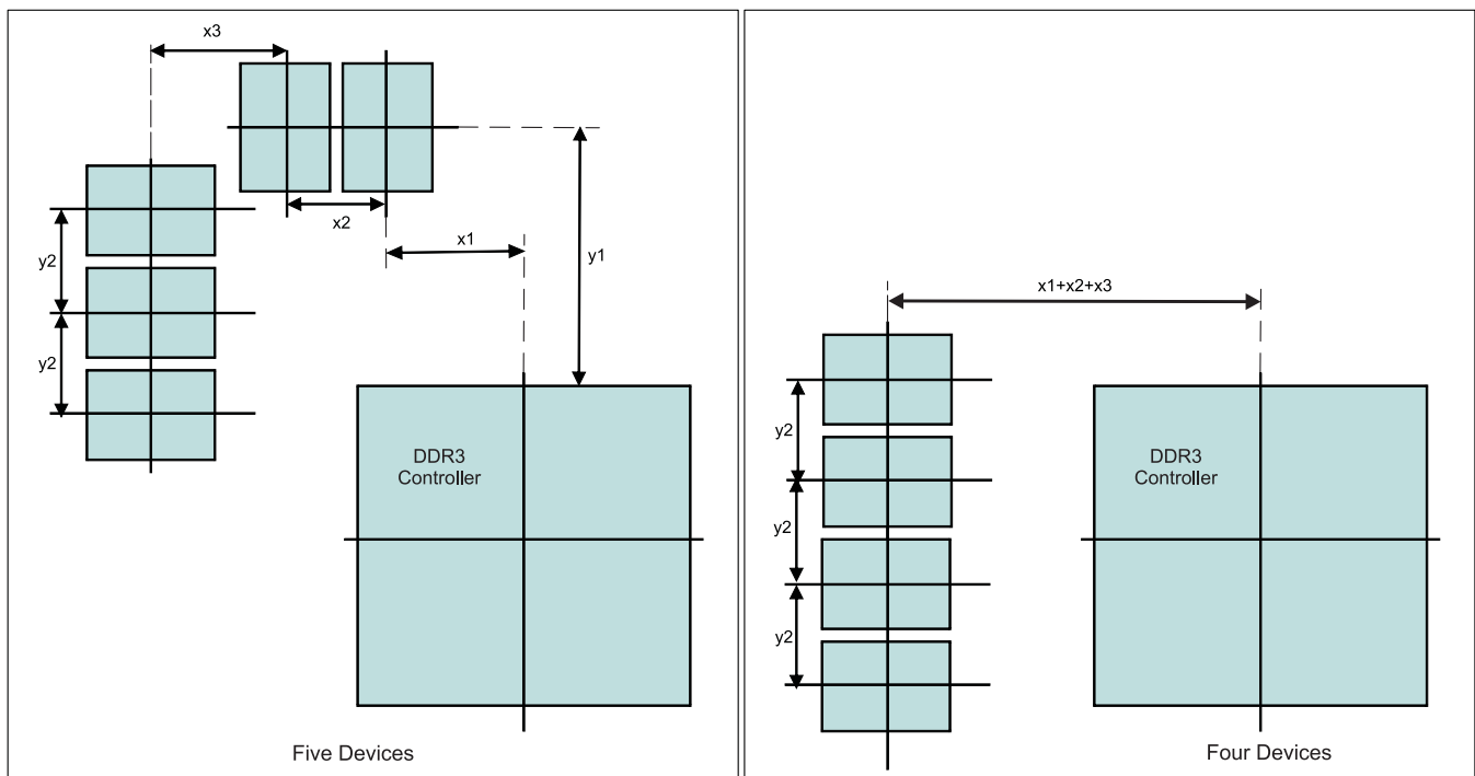
图 7-4. Placement Specifications
