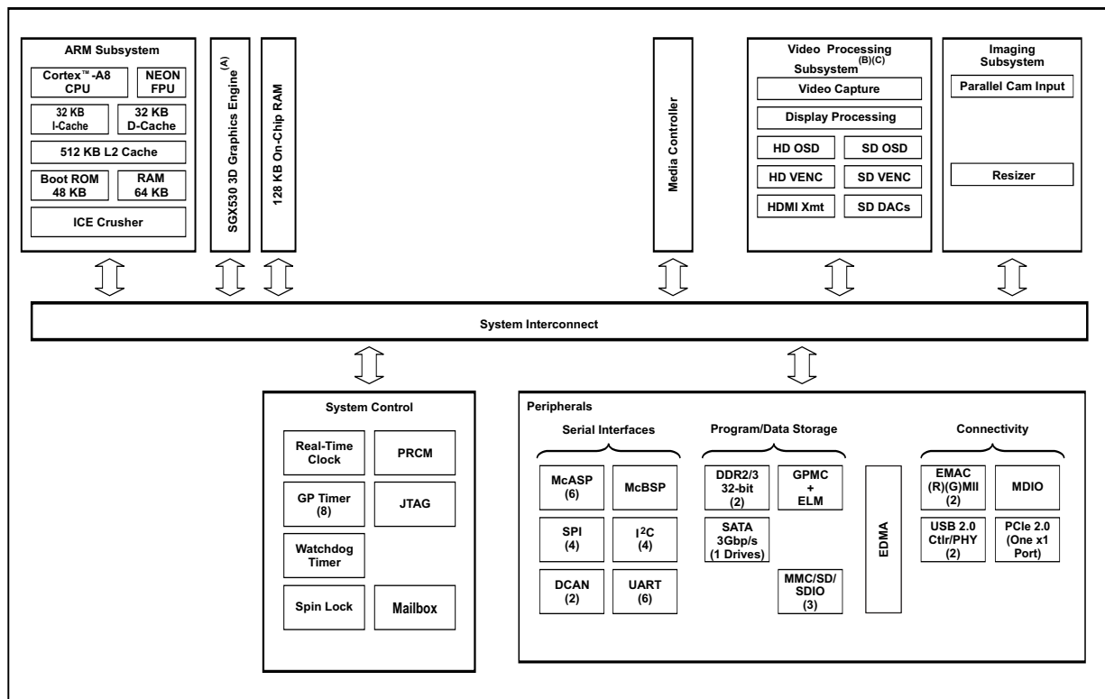
图 1-1. AM387x Sitara™ ARM 处理器功能方框图
