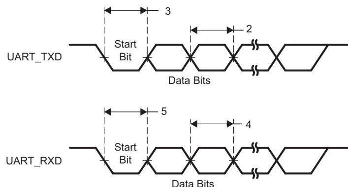
图 7-109. PRU-ICSS UART Timing
