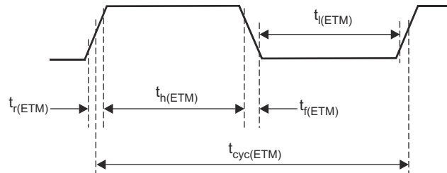
图 6-24. ETMTRACECLKOUT Timing
