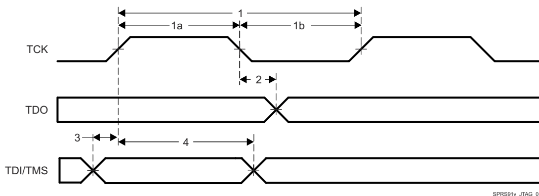
图 6-23. JTAG Timing
