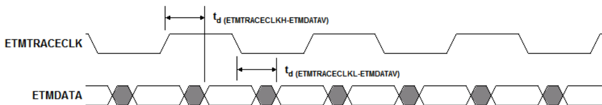
图 6-25. ETMDATA Timing
