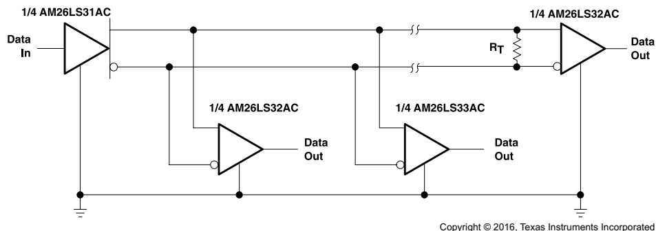
图 9-1. Application Diagram
