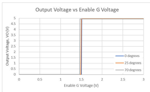
图 6-5. Output Voltage vs Enable G Voltage
