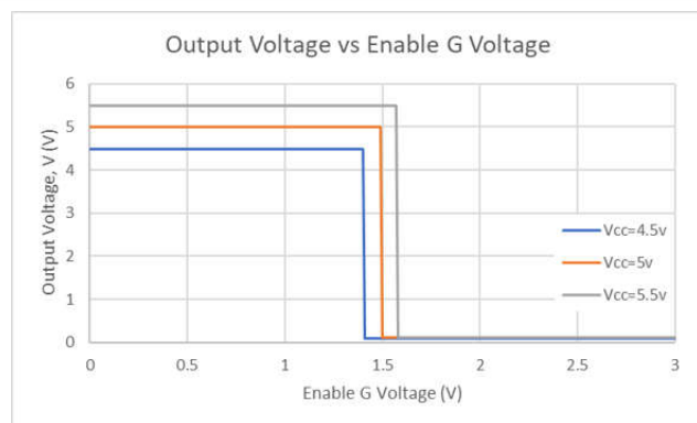
图 6-6. Output Voltage vs Enable G Voltage
