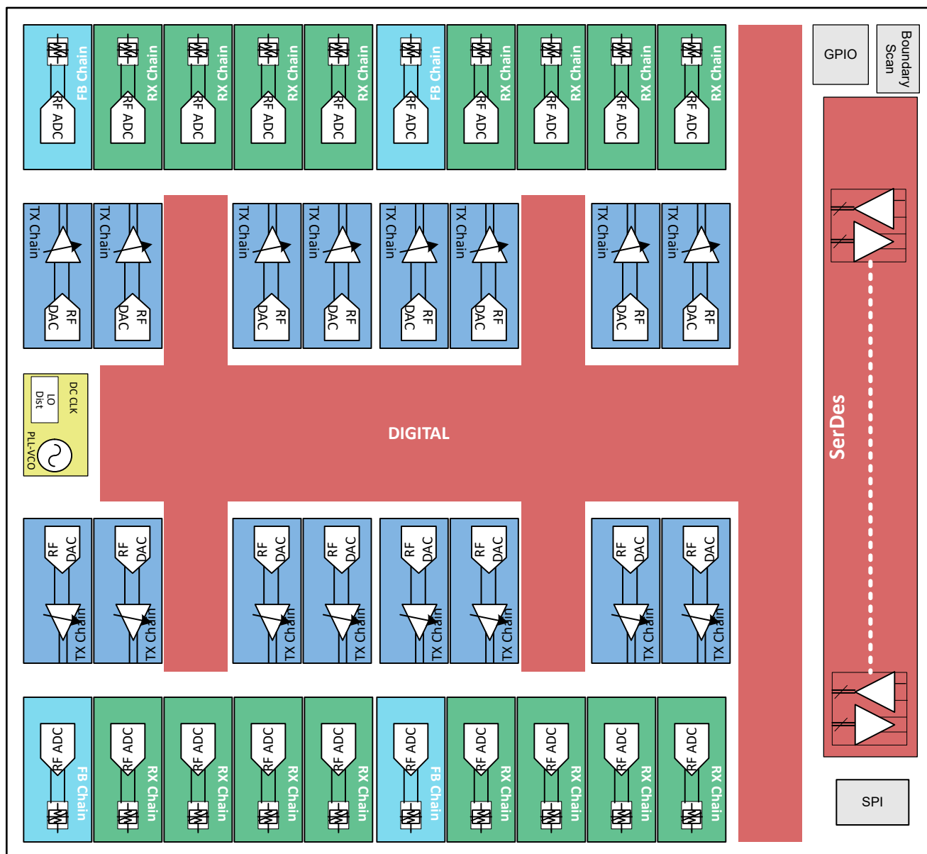
功能方框图
