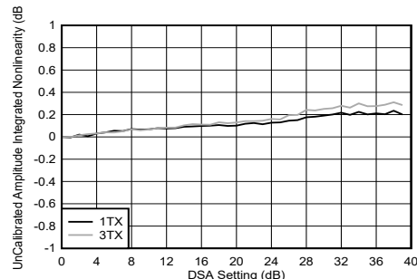
图 4-191. 8.1GHz 条件下 TX DSA 未校准振幅积分非线性
