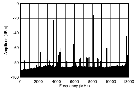
图 4-209. 8.11GHz 条件下 TX 双音输出频谱
