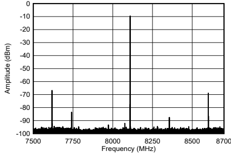
图 4-206. 8.11GHz 条件下 TX 单音输出频谱
