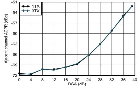
图 4-71. 1.8GHz 条件下 TX 20MHz LTE ACPR 与 DSA 间的关系
