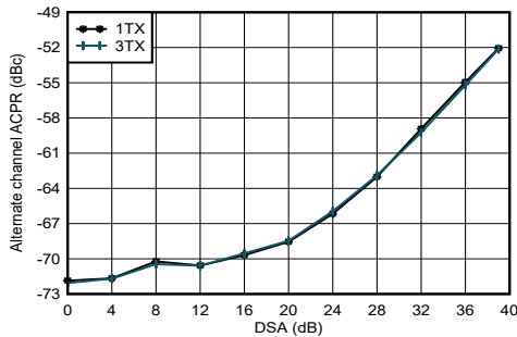
图 4-70. 1.8425GHz 条件下 TX 20MHz LTE alt-ACPR 与数字电平间的关系
