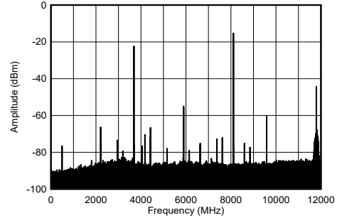
图 4-207. 8.11GHz 条件下 TX 单音输出频谱
