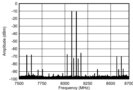
图 4-208. 8.11GHz 条件下 TX 单音输出频谱
