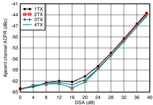
图 7-175. 4.9GHz 条件下 TX 20MHz LTE ACPR 与数字电平间的关系
