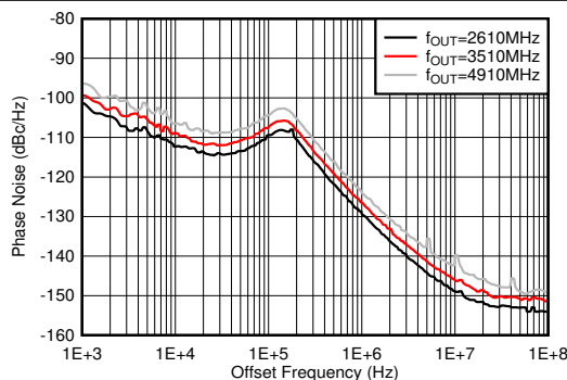
图 7-498. 25°C 条件下 9GHz VCO 相位噪声与偏移频率和 f_{OUT} 间的关系
