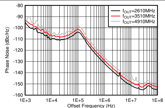
图 7-475. 25°C 条件下 12GHz VCO 相位噪声与偏移频率和 f_{\text{OUT}} 间的关系
