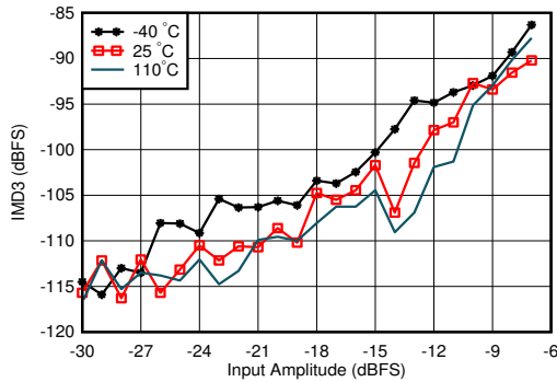
图 7-296. 0.8GHz 条件下 RX IMD3 与输入电平和温度间的关系
