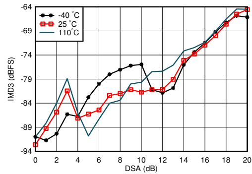
图 7-401. 4.9GHz 条件下 RX IMD3 与 DSA 设置和温度间的关系
