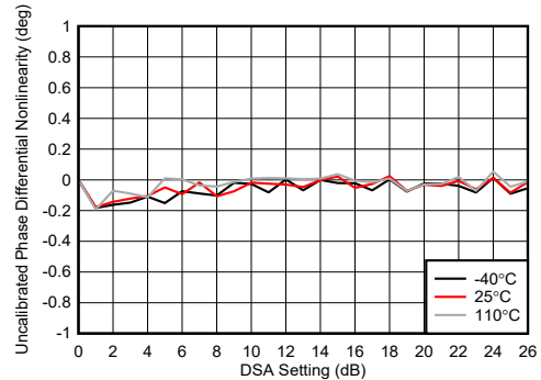
图 7-242. TX DSA 未校准相位微分非线性
