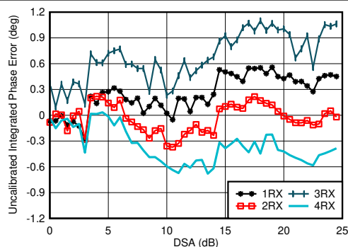
图 7-285. 0.8GHz 条件下 RX 未校准差分相位误差与 DSA 设置间的关系
