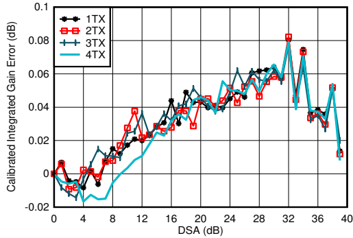
图 7-5. 0.85GHz 条件下 TX 校准差分增益误差与 DSA 设置和通道间的关系
