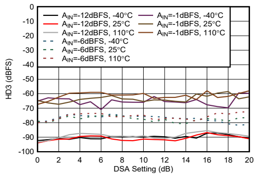
图 7-460. 9.6 GHz 条件下 RX HD3 与 DSA 设置间的关系
