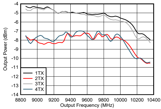
图 7-229. 9.61GHz 条件下 TX 输出功率与频率间的关系
