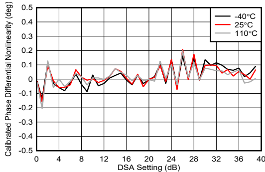
图 7-198. 8.1GHz 条件下 TX DSA 校准相位微分非线性
