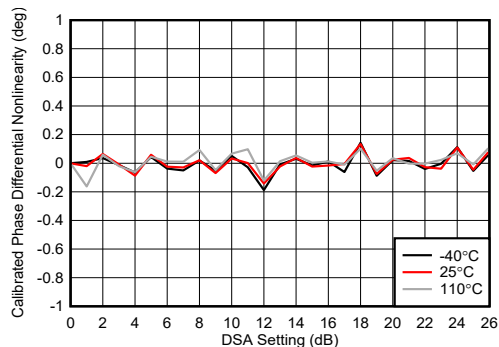
图 7-243. TX DSA 校准相位微分非线性
