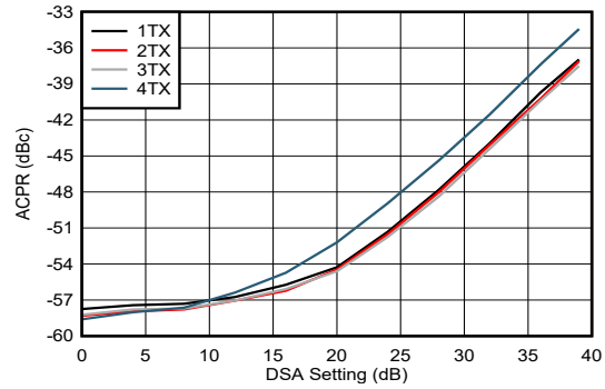
图 7-223. 8.11GHz 条件下 TX NR100MHz alt-ACPR 与 DSA 设置间的关系
