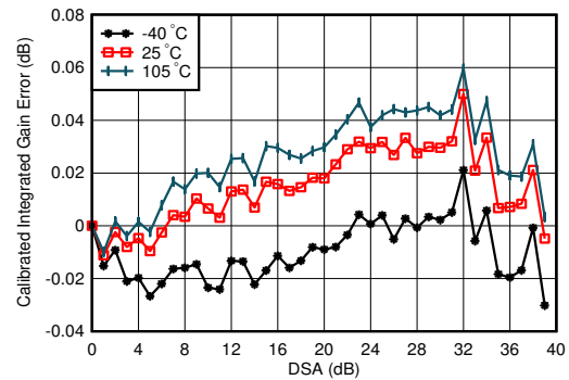
图 7-85. 2.6GHz 条件下 TX 校准差分增益误差与 \text{DSa} 设置和温度间的关系
