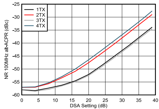
图 7-274. 9.61GHz 条件下 TX NR100MHz alt-ACPR 与 DSA 设置间的关系
