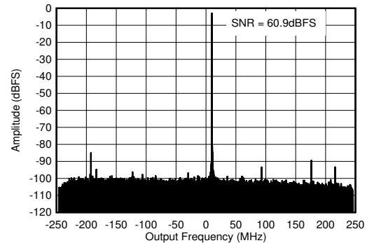
图 7-320. 1.75GHz 条件下的 RX 输出 FFT
