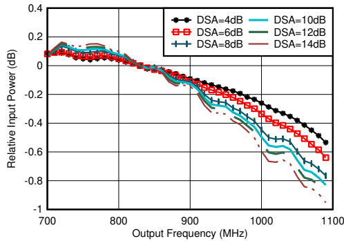
图 7-278. 通道 1RX 的 RX 带内增益平坦度， f_{\text{IN}} = 830\text{MHz}
