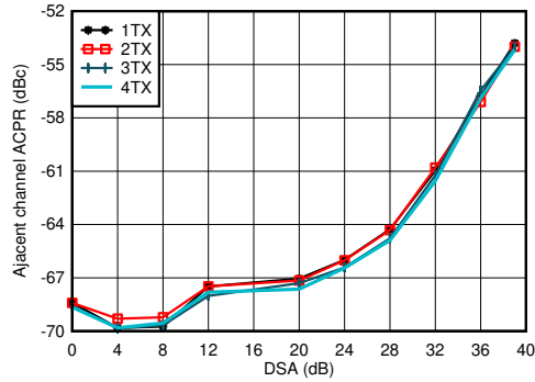
图 7-35. 0.85GHz 条件下 TX 20MHz LTE ACPR 与 DSA 间的关系
