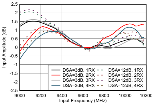
标准化为 9.6GHz，9.6GHz 条件下 RX 输入振幅与频率间的关系 图 7-444. RX 输入振幅与频率间的关系
