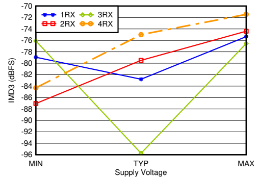
图 7-413. 4.9GHz 条件下 RX IMD3 与电源和通道间的关系
