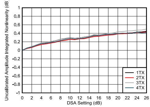
图 7-236. TX DSA 未校准振幅积分非线性
