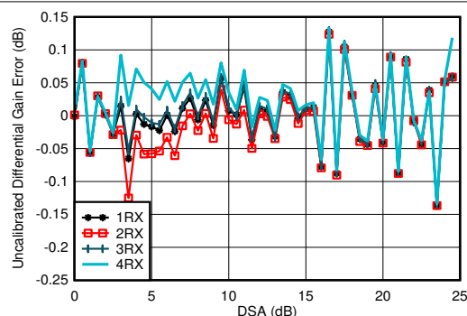
图 7-389. 4.9GHz 条件下 RX 未校准差分振幅误差与 DSA 设置间的关系
