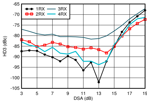
图 7-331. 1.9GHz 条件下 RX HD3 与 DSA 设置和通道间的关系
