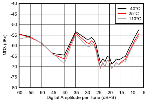
图 7-214. 8.1GHz 条件下 TX IMD3 与数字振幅间的关系
