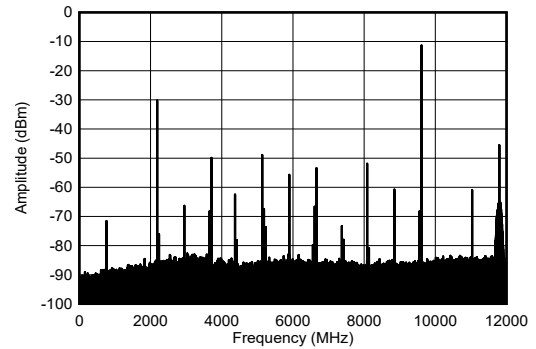
图 7-262. 9.61GHz 和 -1dBFS (宽带) 条件下 TX 单音频谱
