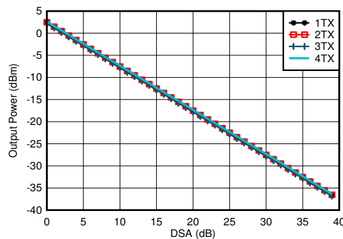
图 7-79. 2.6GHz 条件下 TX 输出功率与 DSA 设置和通道间的关系
