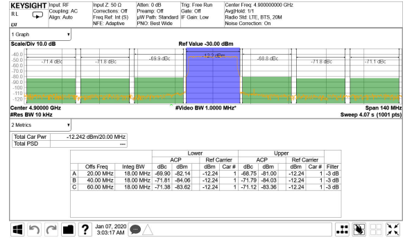
图 7-174. 4.9GHz 条件下的 TX 20MHz LTE 输出频谱
