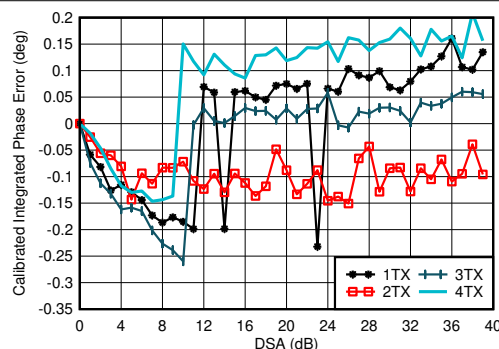
图 7-89. 2.6GHz 条件下 TX 校准差分相位误差与 DSA 设置和通道间的关系
