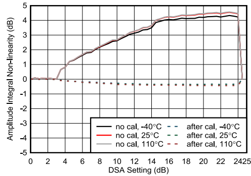
图 7-419. 8.11GHz 条件下 RX 振幅积分非线性
