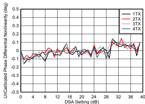
图 7-195. 8.1GHz 条件下 TX DSA 未校准相位微分非线性
