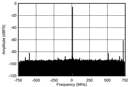
图 7-462. 9.61GHz 条件下 RX 单音输出 FFT
