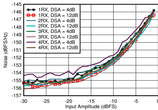
图 7-400. 4.9GHz 条件下 RX 噪声频谱密度与输入振幅和通道间的关系
