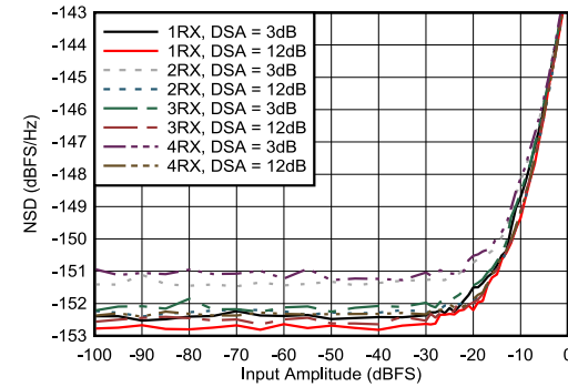
图 7-455. 9.6GHz 条件下 RX NSD 与数字振幅间的关系
