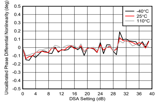
图 7-197. 8.1GHz 条件下 TX DSA 未校准相位微分非线性
