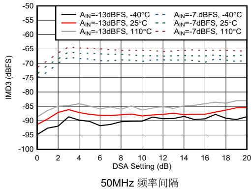
图 7-423. 8.11 GHz 条件下 RX IMD3 与 DSA 设置间的关系
