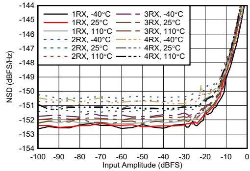
图 7-454. 9.6GHz 条件下 RX NSD 与数字振幅间的关系
