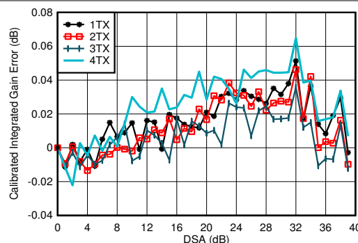
图 7-81. 2.6GHz 条件下 TX 校准差分增益误差与 DSA 设置和通道间的关系
