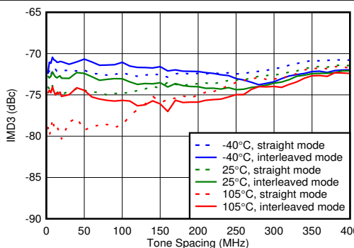
图 7-99. 2.6GHz 条件下 TX IMD3 与频率间隔和温度间的关系
