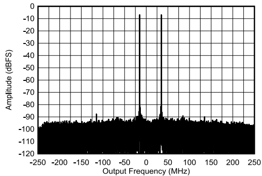
图 7-466. 9.61GHz 条件下 RX 单音输出 FFT
