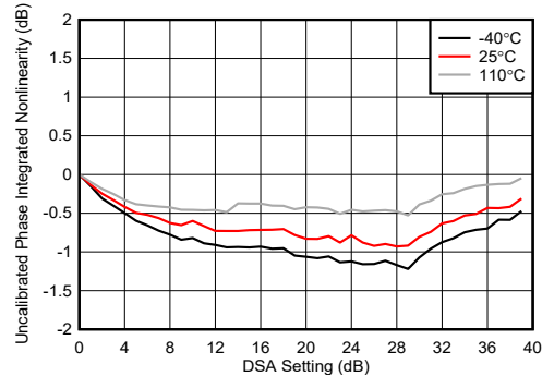
图 7-201. 8.1GHz 条件下 TX DSA 未校准相位积分非线性
