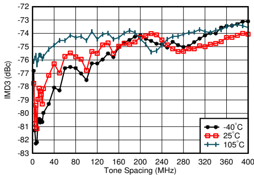
图 7-25. 0.85GHz 条件下 TX IMD3 与频率间隔和温度间的关系
