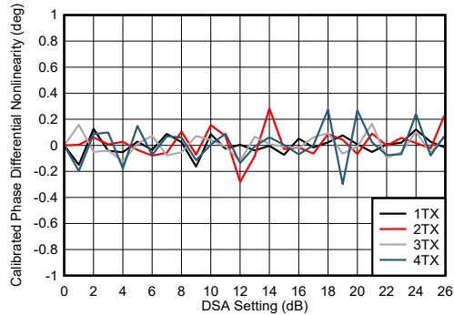
图 7-241. TX DSA 校准相位微分非线性
