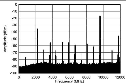
图 7-270. 9.61GHz 和 -12dBFS (宽带) 条件下 TX 双音频谱
