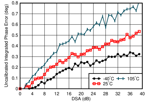
图 7-164. 4.9GHz 条件下 TX 未校准差分相位误差与 DSA 设置和温度间的关系
