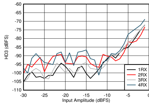
图 7-378. 3.6GHz 条件下 RX HD3 与输入电平和通道间的关系
