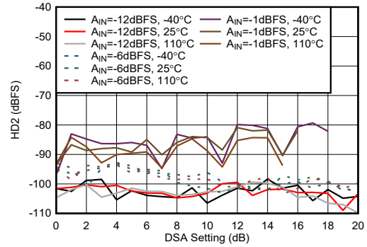
图 7-430. 8.1 GHz 条件下 RX HD2 与 DSA 设置间的关系
