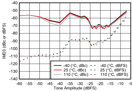
图 7-249. 9.61GHz 条件下 TX IMD3 与数字振幅间的关系
