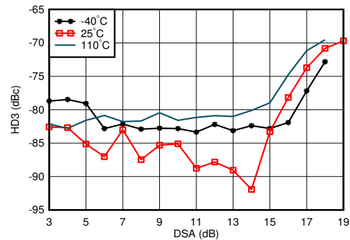
图 7-332. 1.9GHz 条件下 RX HD3 与 DSA 设置和温度间的关系
