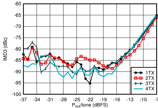
图 7-29. 0.85GHz 条件下 TX IMD3 与数字电平间的关系
