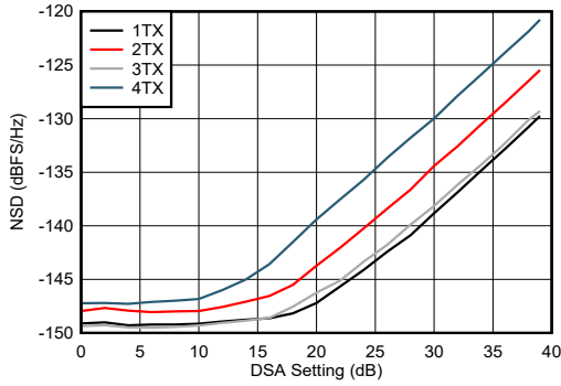
图 7-259. 9.61 GHz 条件下 TX NSD 与 DSA 设置间的关系
