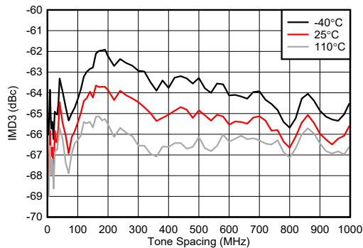
图 7-255. 9.61GHz 条件下 TX IMD3 与频率间隔间的关系
