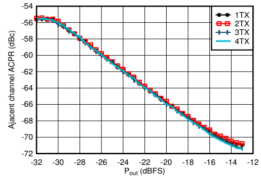
图 7-69. 1.8425GHz 条件下 TX 20MHz LTE ACPR 与数字电平间的关系
