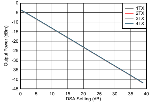
图 7-185. 8.11 GHz 条件下 TX 输出功率与 DSA 设置间的关系
