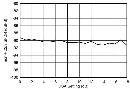
图 7-356. 2.6GHz 条件下 Rx 非 HD2/3 与 DSA 设置间的关系
