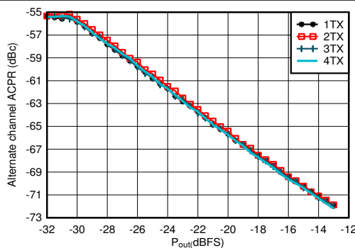
图 7-70. 1.8425GHz 条件下 TX 20MHz LTE alt-ACPR 与数字电平间的关系
