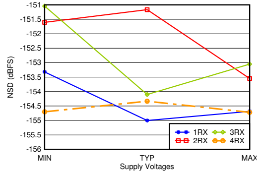
图 7-338. 1.75GHz 条件下 RX 噪声频谱密度与电源和通道间的关系
