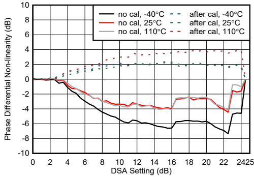
图 7-421. 8.11GHz 条件下 RX 相位积分非线性
