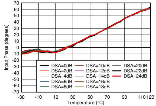
图 7-360. 3.6GHz 条件下 RX 输入相位与温度间的关系
