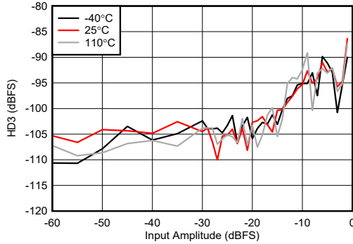
图 7-431. 8.1GHz 条件下 RX HD3 与数字振幅间的关系
