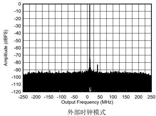
图 7-434. 8.1GHz 条件下 RX 单音输出 FFT, -1dBFS
