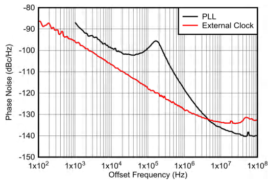
图 7-472. 12GHz 条件下 PLL 和外部时钟的相位噪声与偏移频率间的关系
