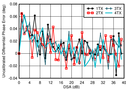
图 7-124. 3.5GHz 条件下 TX 未校准差分相位误差与 DSA 设置和通道间的关系
