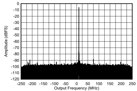
图 7-436. 8.11GHz 条件下 RX 单音输出 FFT，-6dBFS
