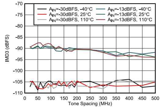
图 7-424. 8.11 GHz 条件下 RX IMD3 与频率间隔间的关系
