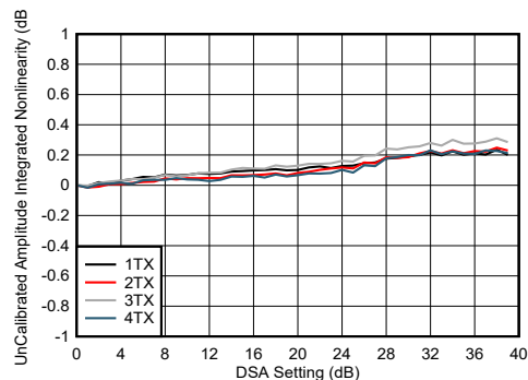
图 7-191. 8.1GHz 条件下 TX DSA 未校准振幅积分非线性
