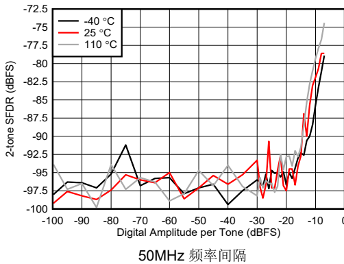
图 7-433. 8.1GHz 条件下 RX 双音 SFDR 与数字振幅间的关系
