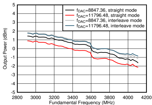
图 7-118. TX 输出功率与频率间的关系
