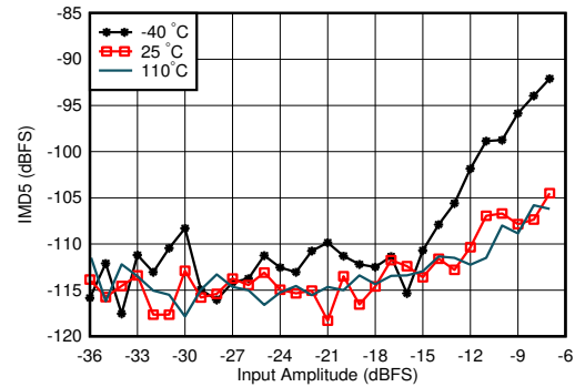
图 7-297. 0.8GHz 条件下 Rx IMD5 与输入电平和温度间的关系
