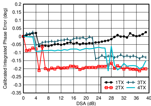
图 7-13. 0.85GHz 条件下 TX 校准差分相位误差与 DSA 设置和通道间的关系
