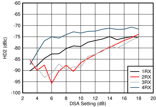
图 7-349. 2.6GHz 条件下 RX HD2 与 DSA 设置和通道间的关系
