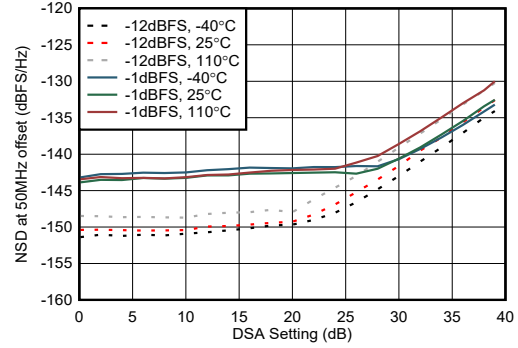
图 7-221. 8.11 GHz 条件下 TX NSD 与 DSA 设置间的关系
