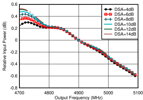
图 7-386. RX 带内增益平坦度， f_{\text{IN}} = 4900\text{MHz}
