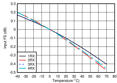
图 7-310. 1.75GHz 条件下 RX 输入满量程与温度和通道间的关系
