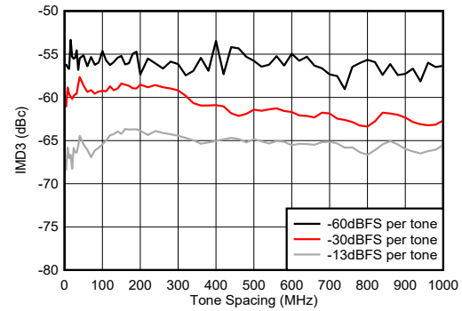
图 7-254. 9.61GHz 条件下 TX IMD3 与频率间隔间的关系
