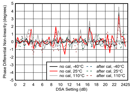
图 7-448. 9.6GHz 条件下 RX 相位微分非线性
