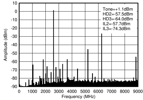
图 7-114. 2.6GHz (0 - f_{\text{DAC}} ) 条件下的 TX 单频 (-12dBFS) 输出频谱
