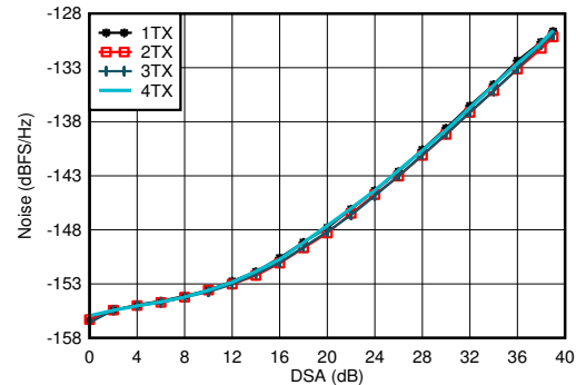
图 7-168. 2.6GHz 条件下 TX 输出噪声与通道和衰减间的关系
