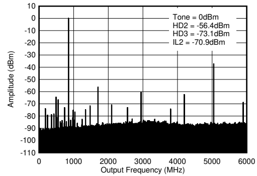
图 7-42. 0.85GHz (0- f_{\text{DAC}} ) 条件下的 TX 单频 (-6dBFS) 输出频谱
