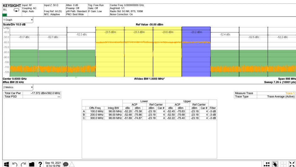
图 7-276. 9.61GHz 条件下 TX NR100MHz 输出频谱
