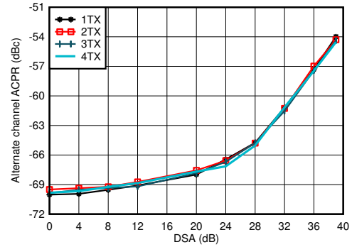
图 7-36. 0.85GHz 条件下 TX 20MHz LTE alt-ACPR 与 DSA 间的关系
