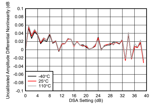
图 7-189. 8.11GHz 条件下 TX DSA 未校准振幅微分非线性
