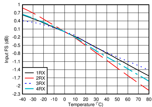
图 7-387. 4.9GHz 条件下 RX 输入满量程与温度和通道间的关系
