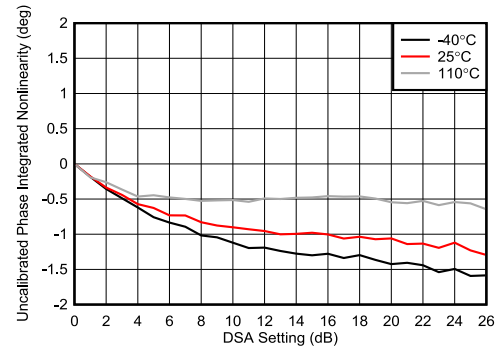
图 7-246. TX DSA 未校准相位积分非线性
