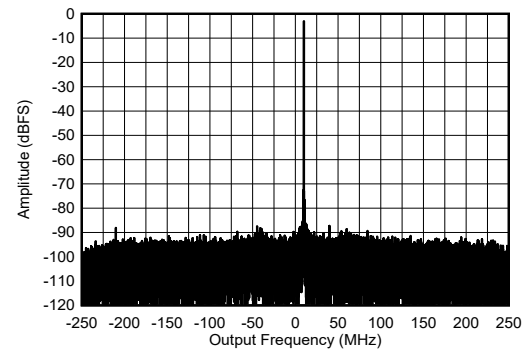
图 7-461. 9.61GHz 条件下 RX 单音输出 FFT
