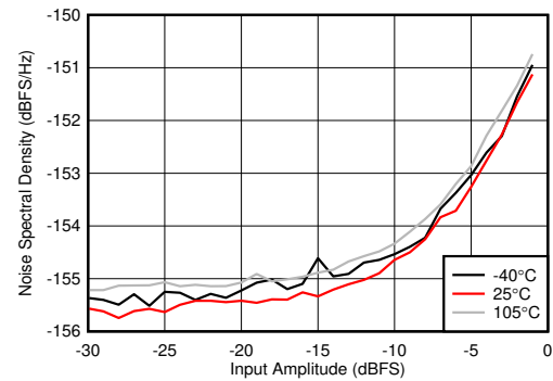
图 7-344. 2.6GHz 条件下 RX 噪声频谱密度与输入振幅和温度间的关系
