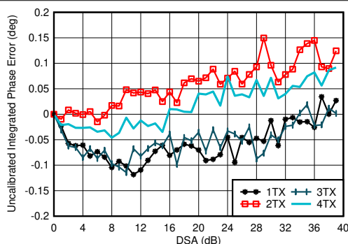
图 7-88. 2.6GHz 条件下 TX 未校准差分相位误差与 DSA 设置和通道间的关系
