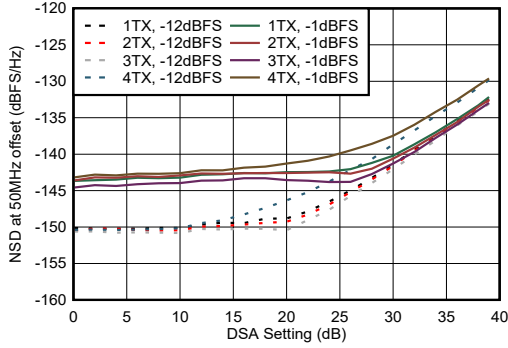
图 7-220. 8.11 GHz 条件下 TX NSD 与 DSA 设置间的关系
