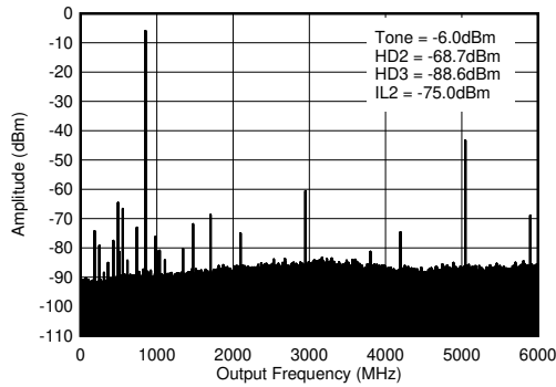
图 7-41. 0.85GHz (0- f_{\text{DAC}} ) 条件下的 TX 单频 (-12dBFS) 输出频谱
