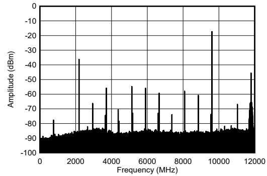
图 7-266. 9.61GHz 和 -12dBFS (宽带) 条件下 TX 单音频谱
