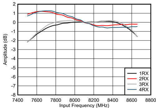
图 7-415. RX 振幅与频率和通道间的关系
