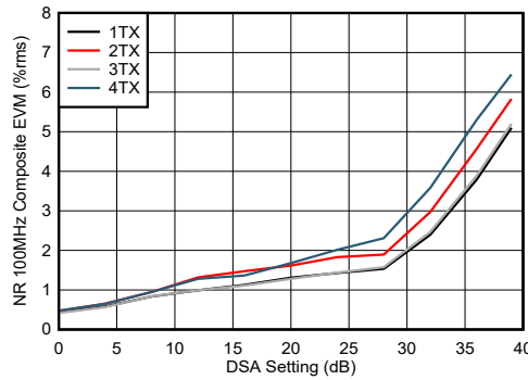
图 7-224. 8.11GHz 条件下 TX NR100MHz EVM 与 DSA 设置间的关系
