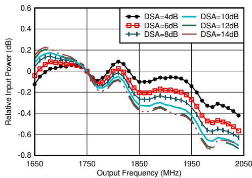
图 7-309. RX 带内增益平坦度， f_{\text{IN}} = 1750\text{MHz}
