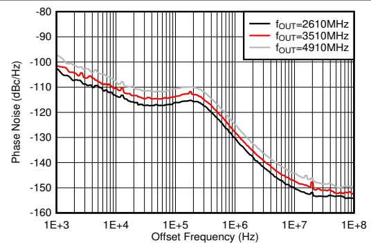
图 7-487. 25°C 条件下的 10GHz VCO 相位噪声与偏移频率和 f_{OUT} 间的关系
