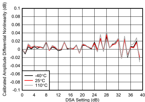
图 7-190. 8.1GHz 条件下 TX DSA 校准振幅微分非线性
