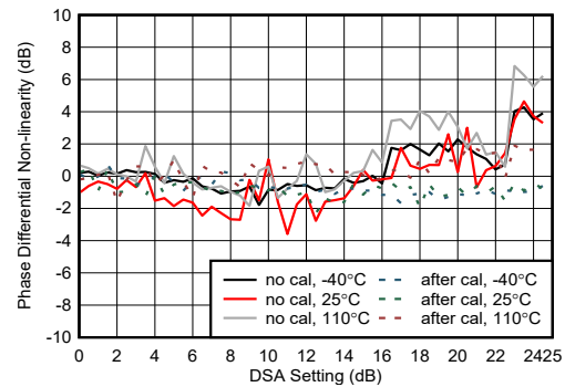
图 7-449. 9.6GHz 条件下 RX 相位积分非线性
