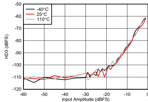
图 7-459. 9.6GHz 条件下 RX HD3 与数字电平间的关系
