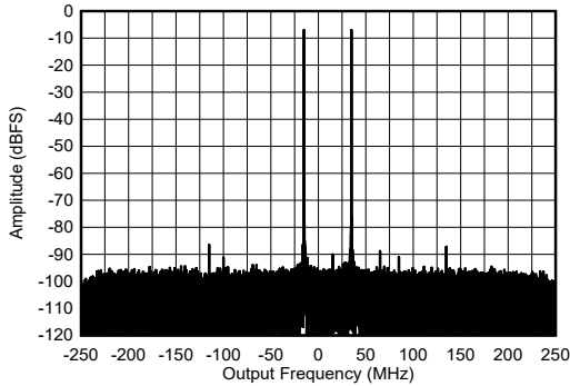
外部时钟模式，单音幅度为 -12dBFS 图 7-441. 8.11GHz 条件下 RX 双音输出 FFT
