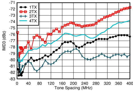
图 7-23. 0.85GHz 条件下 TX IMD3 与频率间隔和通道间的关系
