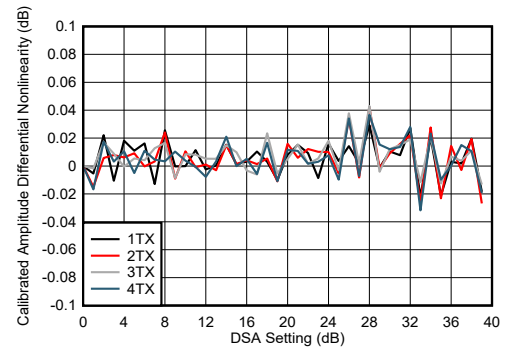
图 7-188. 8.11GHz 条件下 TX DSA 校准振幅微分非线性
