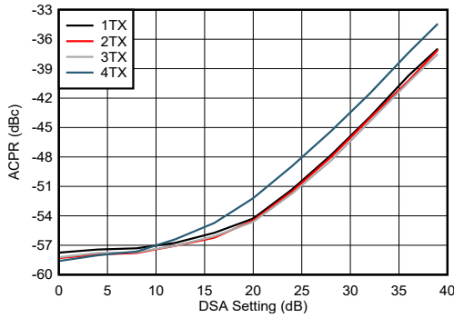
图 7-222. 8.11GHz 条件下 TX NR100MHz ACPR 与 DSA 设置间的关系
