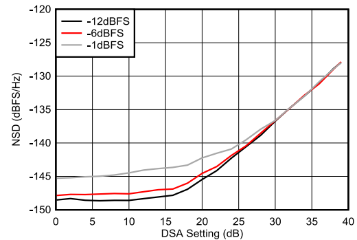
图 7-258. 9.61 GHz 条件下 TX NSD 与 DSA 设置间的关系
