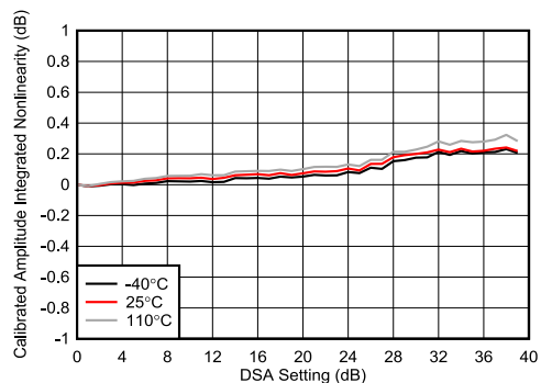
图 7-194. 8.1GHz 条件下 TX DSA 校准振幅积分非线性
