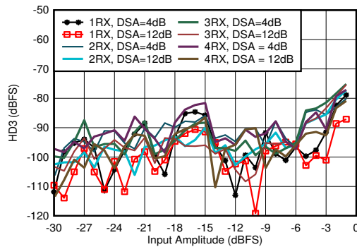
图 7-331. 1.9GHz 条件下 RX HD3 与 DSA 设置和通道间的关系
