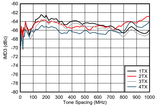
图 7-253. 9.61GHz 条件下 TX IMD3 与频率间隔间的关系
