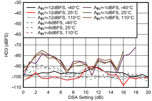
图 7-432. 8.1 GHz 条件下 RX HD3 与 DSA 设置间的关系
