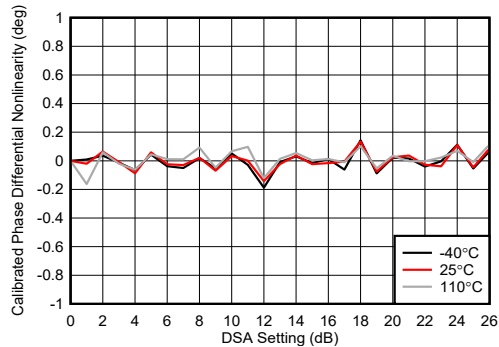
图 7-245. TX DSA 校准相位积分非线性
