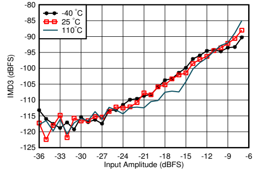
图 7-326. 1.75GHz 条件下 RX IMD3 与输入电平和温度间的关系
