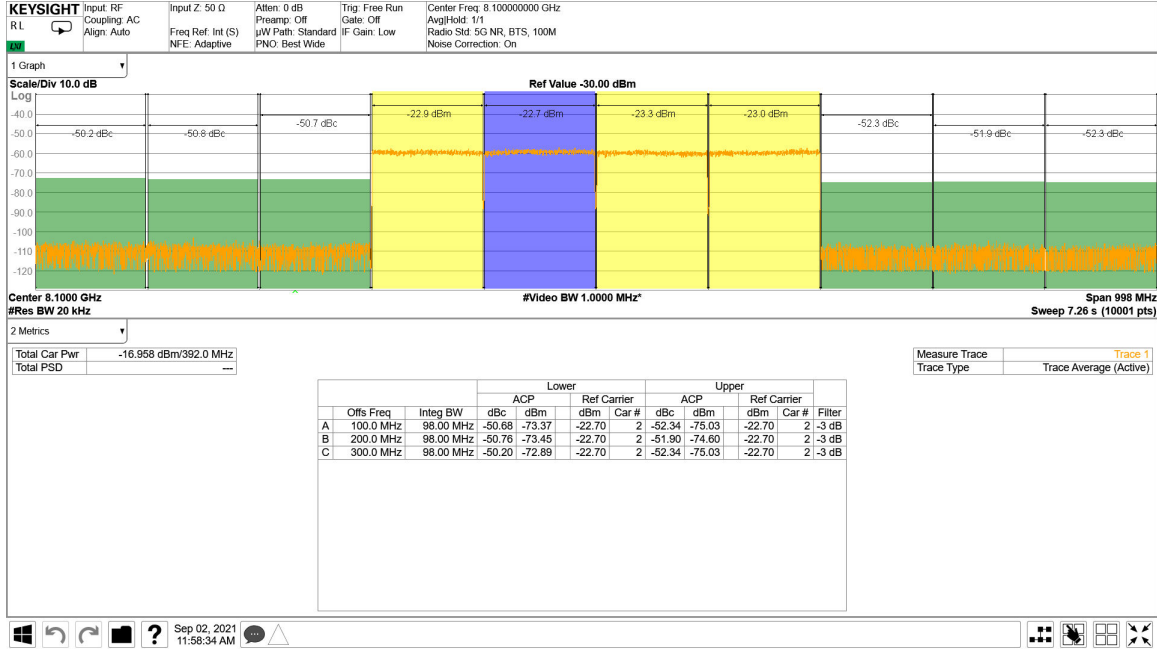
图 7-227. 8.11GHz 条件下 TX 4x100MHz NR 输出频谱
