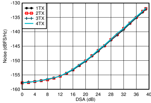
图 7-136. 3.5GHz 条件下 TX NSD 与 DSA 设置间的关系
