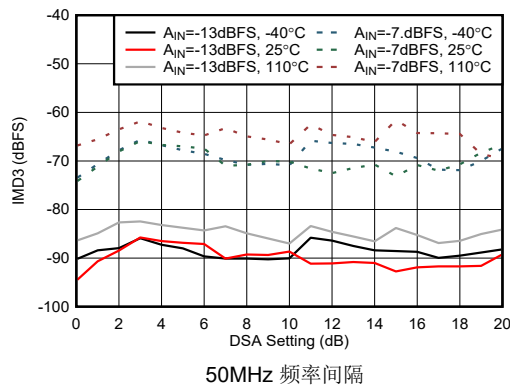
图 7-451. 9.6 GHz 条件下 RX IMD3 与 DSA 设置间的关系
