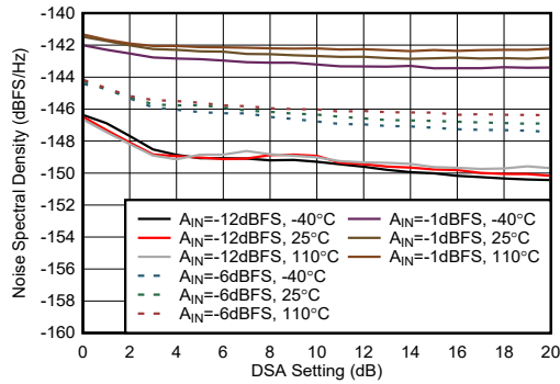
图 7-456. 9.6 GHz 条件下 RX NSD 与 DSA 设置间的关系
