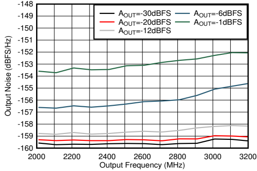
图 7-102. 2.6GHz 条件下 TX 单频输出噪声与频率和振幅间的关系
