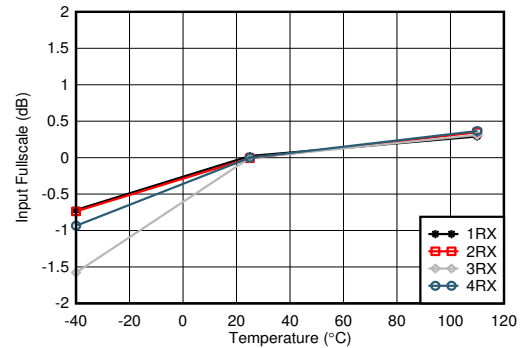
图 7-340. 2.6GHz 条件下 RX 输入满量程与温度和通道间的关系
