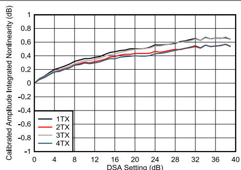
图 7-192. 8.1GHz 条件下 TX DSA 校准振幅积分非线性
