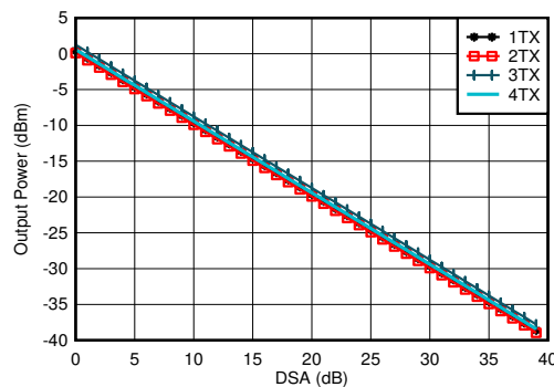
图 7-119. 3.5GHz 条件下 TX 输出功率与 DSA 设置间的关系
