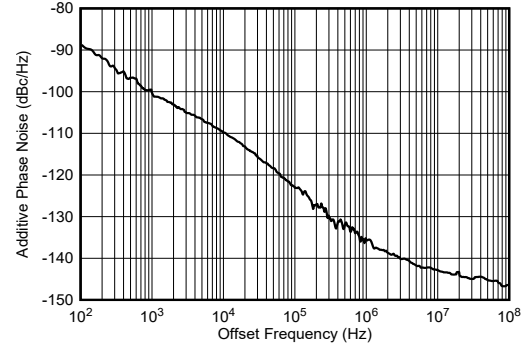
图 7-272. 9.61GHz 条件下 TX 附加相位噪声与偏移频率间的关系
