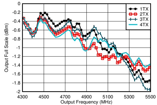
图 7-150. 5898.24MSPS、直接模式、第二奈奎斯特区域条件下的 TX 满量程与射频频率和通道间的关系
