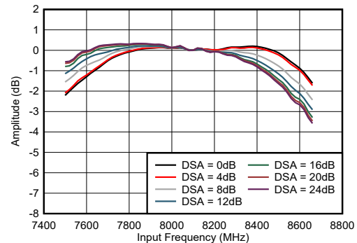
图 7-416. RX 振幅与频率和 DSA 设置间的关系
