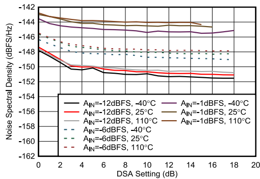
图 7-427. 8.11 GHz 条件下 RX NSD 与 DSA 设置间的关系
