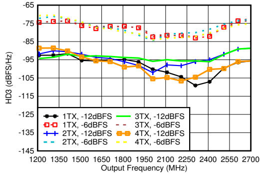
图 7-74. 1.8GHz 条件下 TX HD3 与数字振幅和输出频率间的关系
