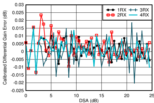
图 7-282. 0.8GHz 条件下 RX 校准差分振幅误差与 DSA 设置间的关系
