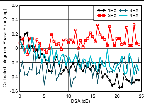
图 7-286. 0.8GHz 条件下 RX 校准差分相位误差与 DSA 设置间的关系
