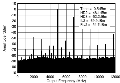
图 7-181. 4.9GHz (0 - f_{\text{DAC}} ) 条件下的 TX 单频 (-12dBFS) 输出频谱
