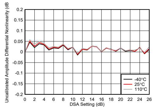
图 7-234. TX DSA 未校准振幅微分非线性
