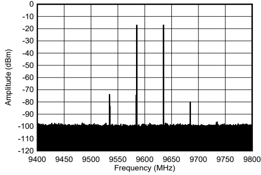
图 7-271. 9.61GHz 和 -12dBFS (400MHz 带宽) 条件下 TX 双音频谱
