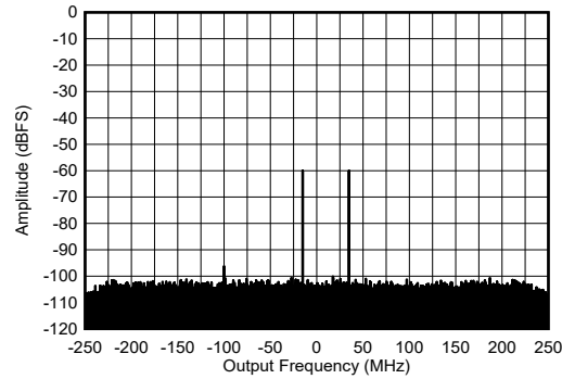
外部时钟模式，单音幅度为 -60dBFS 图 7-443. 8.11GHz 条件下 RX 双音输出 FFT
