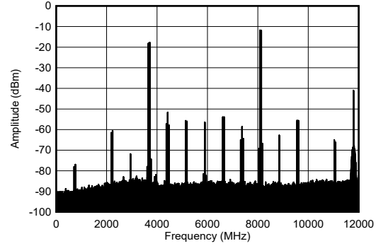
图 7-209. 8.11GHz 条件下 TX 双音输出频谱
