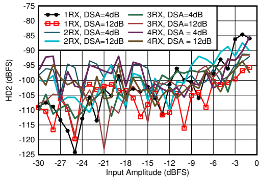
图 7-327. 1.9GHz 条件下 RX HD2 与 DSA 设置和通道间的关系
