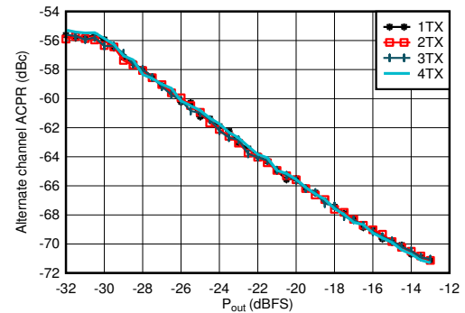
图 7-176. 4.9GHz 条件下 TX 20MHz LTE alt-ACPR 与数字电平间的关系
