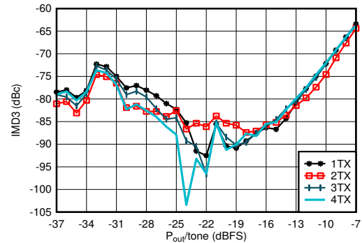
图 7-30. 0.85GHz 条件下 TX IMD3 与数字电平间的关系
