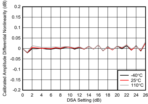
图 7-235. TX DSA 校准振幅微分非线性
