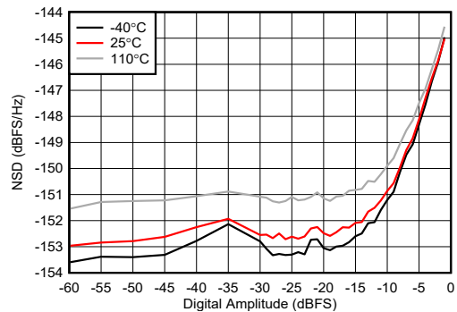
图 7-257. 9.61GHz 条件下 TX NSD 与数字振幅间的关系
