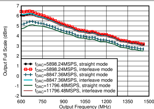
图 7-1. TX 输出满量程与输出频率间的关系
