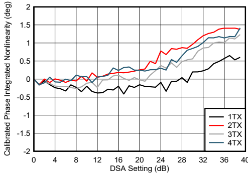
图 7-200. 8.1GHz 条件下 TX DSA 校准相位积分非线性
