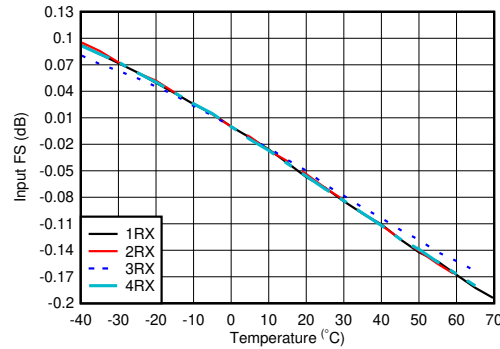
图 7-279. 800MHz 条件下 RX 输入满量程与温度和通道间的关系
