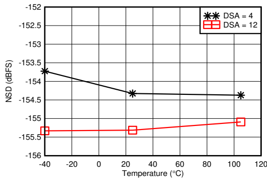
图 7-343. 2.6GHz 条件下 RX 噪声频谱密度与温度间的关系
