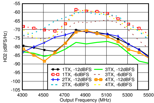
图 7-179. 4.9GHz 条件下 TX HD2 与数字振幅和输出频率间的关系
