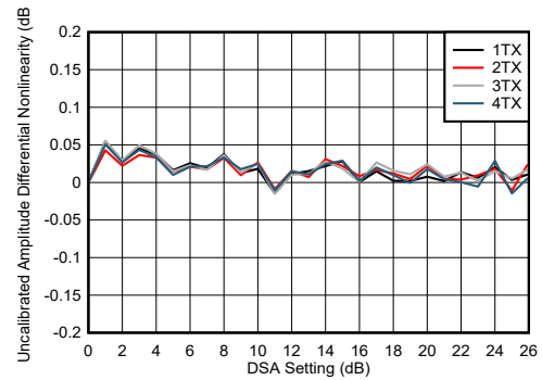
图 7-232. TX DSA 未校准振幅微分非线性
