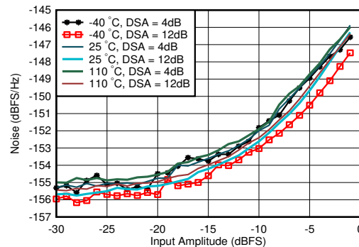
图 7-399. 4.9GHz 条件下 RX 噪声频谱密度与输入振幅和温度间的关系
