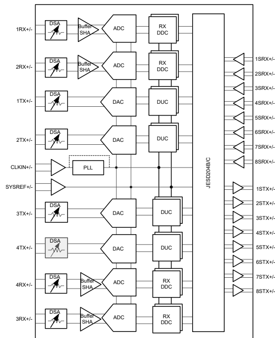
功能模块图
