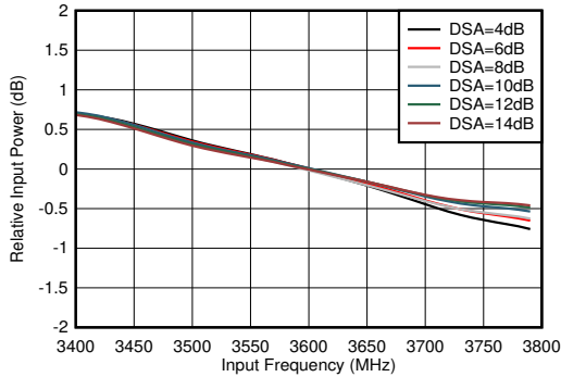
图 7-359. RX 带内增益平坦度， f_{\text{IN}} = 3600\text{MHz}
