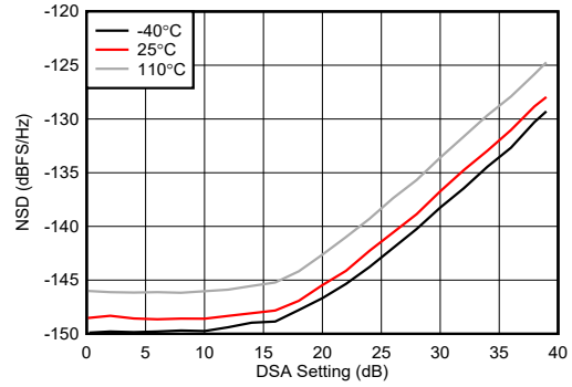
图 7-260. 9.61 GHz 条件下 TX NSD 与 DSA 设置间的关系
