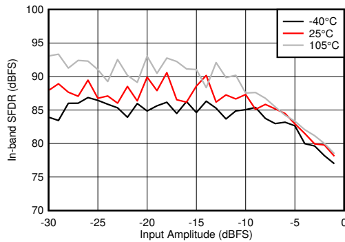
图 7-355. 2.6GHz 条件下 RX 带内 SFDR ( \pm 300\text{MHz} ) 与输入振幅和温度间的关系
