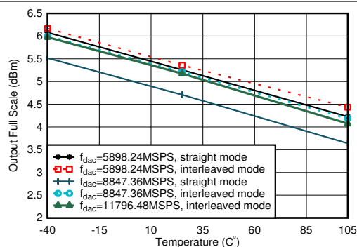
图 7-2. TX 输出满量程与温度间的关系
