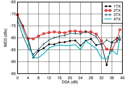
图 7-63. 1.8 GHz 条件下 TX IMD3 与 DSA 设置间的关系
