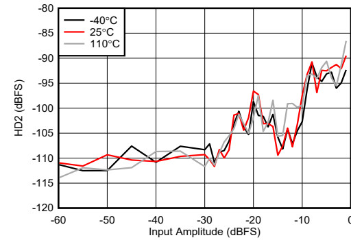
图 7-457. 9.6GHz 条件下 RX HD2 与数字电平间的关系
