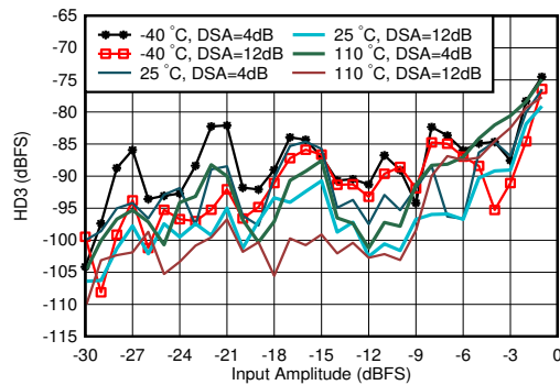
图 7-332. 1.9GHz 条件下 RX HD3 与 DSA 设置和温度间的关系
