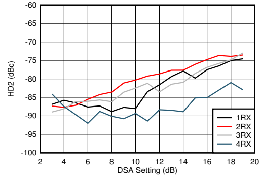
图 7-372. 3.6GHz 条件下 RX HD2 与 DSA 设置和通道间的关系
