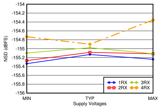
图 7-308. 0.8GHz 条件下 RX 噪声频谱密度与电源和通道间的关系
