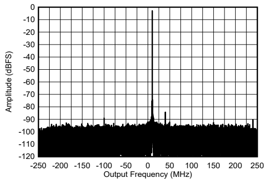
图 7-435. 8.11GHz 条件下 RX 单音输出 FFT，-3dBFS
