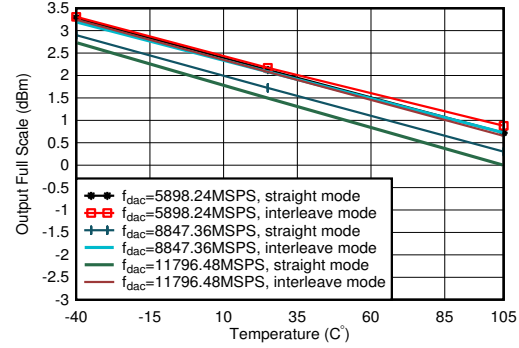
图 7-45. 1.8GHz 条件下 TX 输出功率与温度间的关系
