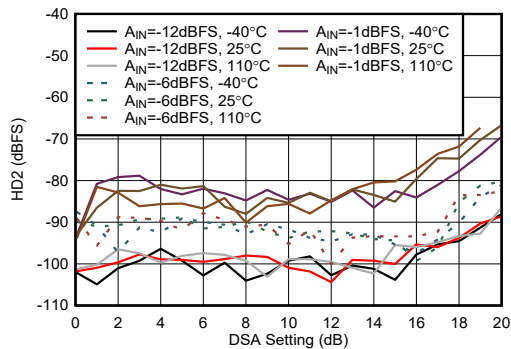
图 7-458. 9.6 GHz 条件下 RX HD2 与 DSA 设置间的关系
