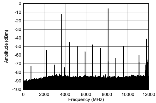
图 7-203. 8.1GHz 条件下 TX 单音输出频谱
