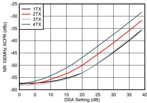
图 7-273. 9.61GHz 条件下 TX NR100MHz ACPR 与 DSA 设置间的关系
