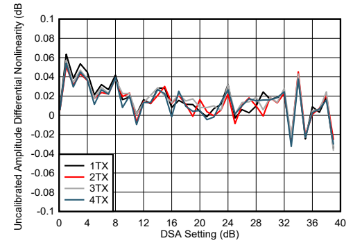
图 7-187. 8.11GHz 条件下 TX DSA 未校准振幅微分非线性
