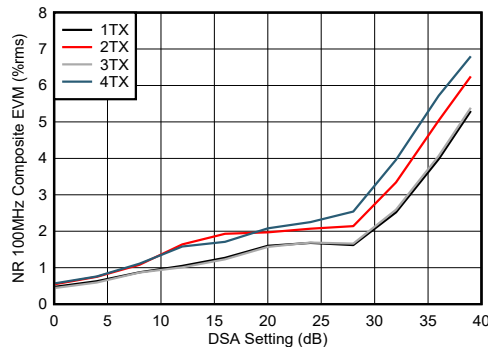
图 7-275. 9.61GHz 条件下 TX NR100MHz EVM 与 DSA 设置间的关系
