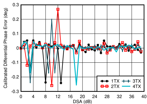
图 7-125. 3.5GHz 条件下 TX 校准差分相位误差与 DSA 设置和通道间的关系
