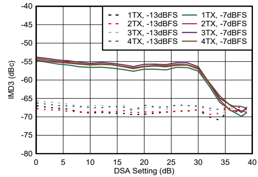
图 7-215. 8.1 GHz 条件下 TX IMD3 与 DSA 设置间的关系
