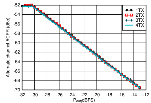
图 7-34. 0.85GHz 条件下 TX 20MHz LTE alt-ACPR 与数字电平间的关系
