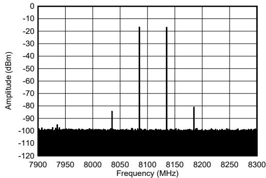
图 7-210. 8.11GHz 条件下 TX 双音输出频谱
