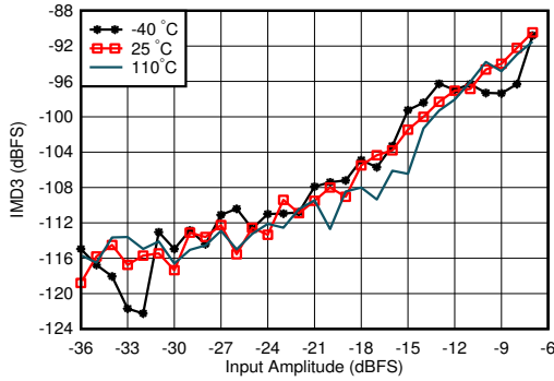
图 7-325. 1.75GHz 条件下 RX IMD3 与输入电平和温度间的关系
