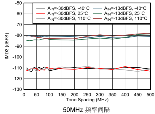
图 7-453. 9.6 GHz 条件下 RX IMD3 与频率间隔间的关系
