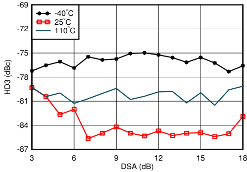
图 7-302. 0.8GHz 条件下 RX HD3 与 DSA 设置和温度间的关系
