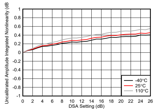
图 7-238. TX DSA 未校准振幅积分非线性
