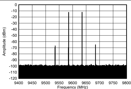
图 7-267. 9.61GHz 和 -12dBFS (400MHz 带宽) 条件下 TX 单音频谱
