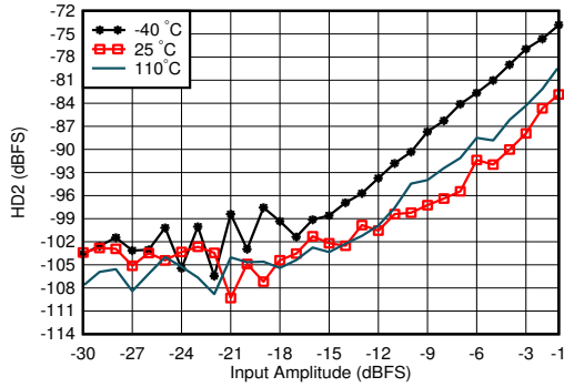
图 7-406. 4.9GHz 条件下 RX HD2 与输入电平和温度间的关系
