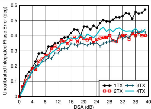
图 7-126. 3.5GHz 条件下 TX 未校准积分相位误差与 DSA 设置和通道间的关系
