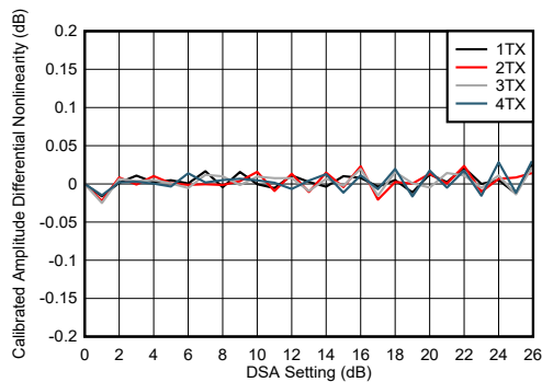
图 7-233. TX DSA 校准振幅微分非线性
