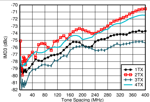
图 7-22. 0.85GHz 条件下 TX IMD3 与频率间隔和通道间的关系
