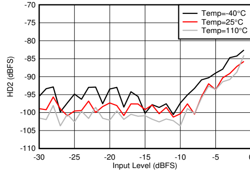
图 7-350. 2.6GHz 条件下 RX HD2 与输入电平和温度间的关系
