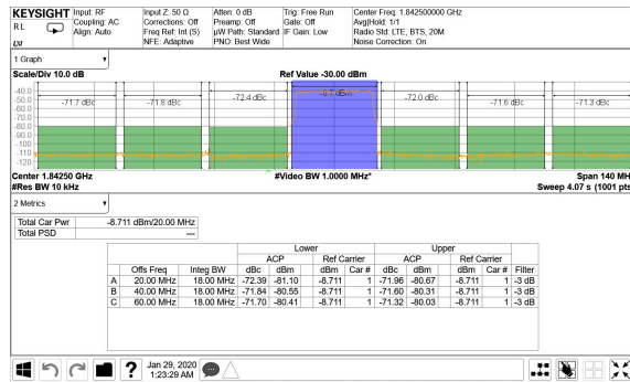
图 7-68. 1.8425GHz 条件下的 TX 20MHz LTE 输出频谱
