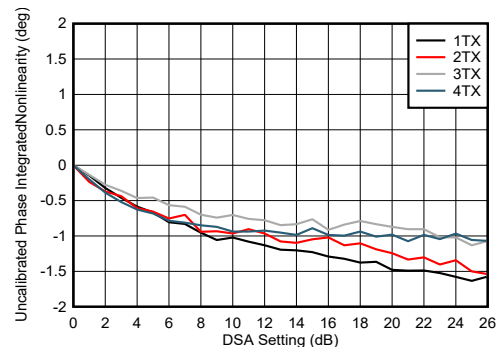
图 7-244. TX DSA 未校准相位积分非线性
