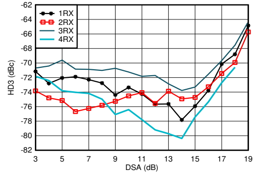
图 7-407. 4.9GHz 条件下 RX HD3 与 DSA 设置和通道间的关系
