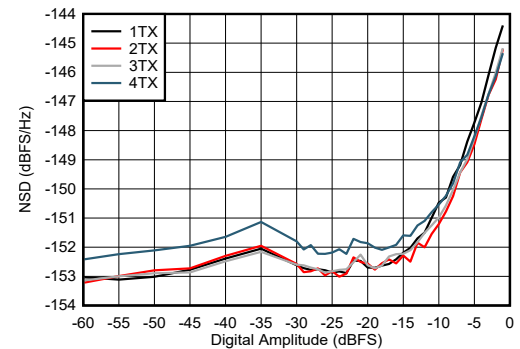
图 7-256. 9.61GHz 条件下 TX NSD 与数字振幅间的关系
