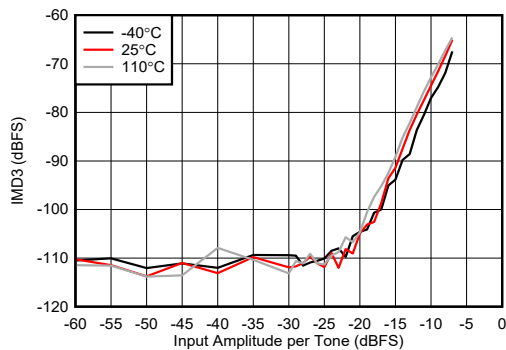
图 7-450. 9.6GHz 条件下 RX IMD3 与数字振幅间的关系
