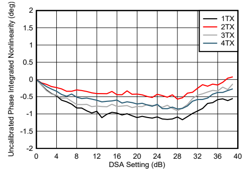
图 7-199. 8.1GHz 条件下 TX DSA 未校准相位积分非线性
