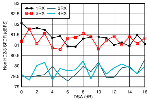
图 7-412. 4.9GHz 条件下 RX 非 HD2/3 与 DSA 设置间的关系
