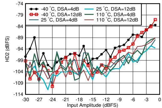
图 7-328. 1.9GHz 条件下 RX HD2 与 DSA 设置和温度间的关系
