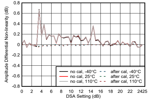
图 7-418. 8.11GHz 条件下 RX 振幅微分非线性
