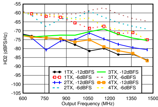
图 7-37. 0.85GHz 条件下 TX HD2 与数字振幅和输出频率间的关系
