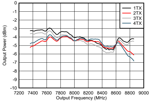
图 7-184. 8.11GHz 条件下 TX 输出功率与频率间的关系
