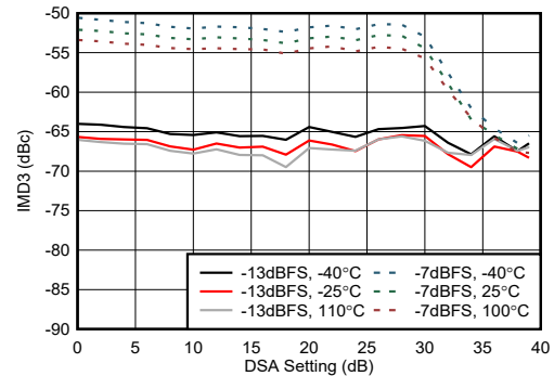
图 7-250. 9.61 GHz 条件下 TX IMD3 与 DSA 设置间的关系
