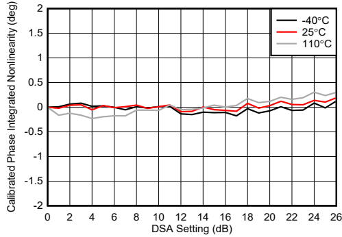
图 7-247. TX DSA 校准振幅积分非线性
