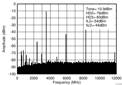
图 7-148. 3.5GHz (0 - f_{\text{DAC}} ) 条件下的 TX 单频 (-12dBFS) 输出频谱
