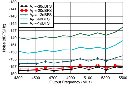
图 7-173. 4.9 GHz 条件下 TX 单频输出噪声与频率和振幅间的关系
