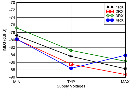
图 7-383. 3.6GHz 条件下 RX IMD3 与电源电压和通道间的关系
