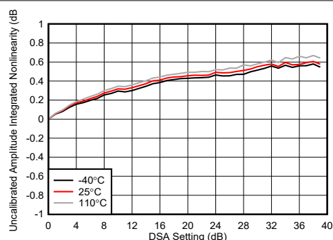
图 7-193. 8.1GHz 条件下 TX DSA 未校准振幅积分非线性
