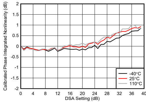
图 7-202. 8.1GHz 条件下 TX DSA 校准相位积分非线性
