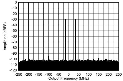
外部时钟模式，单音幅度为 -30dBFS 图 7-442. 8.11GHz 条件下 RX 双音输出 FFT
