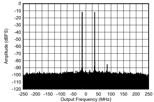
图 7-467. 9.61GHz 条件下 RX 单音输出 FFT
