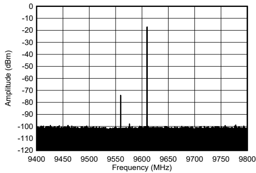
图 7-265. 9.61GHz 和 -6dBFS (400MHz 带宽) 条件下 TX 单音频谱
