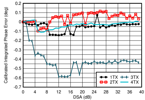
图 7-55. 1.8 GHz 条件下 TX 校准差分相位误差与 DSA 设置和通道间的关系
