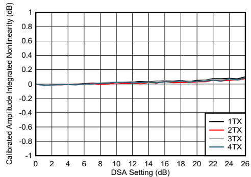
图 7-237. TX DSA 校准振幅积分非线性
