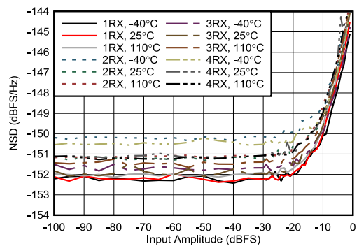
图 7-425. 8.11GHz 条件下 RX NSD 与数字振幅间的关系
