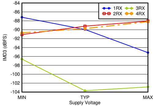
图 7-337. 1.75GHz 条件下 RX IMD3 与电源和通道间的关系
