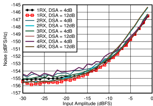
图 7-323. 1.75GHz 条件下 RX 噪声频谱密度与输入振幅和通道间的关系
