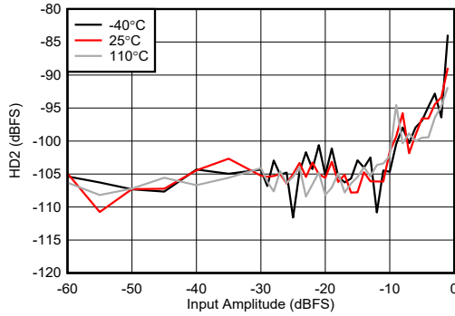
图 7-429. 8.1GHz 条件下 RX HD2 与数字振幅间的关系
