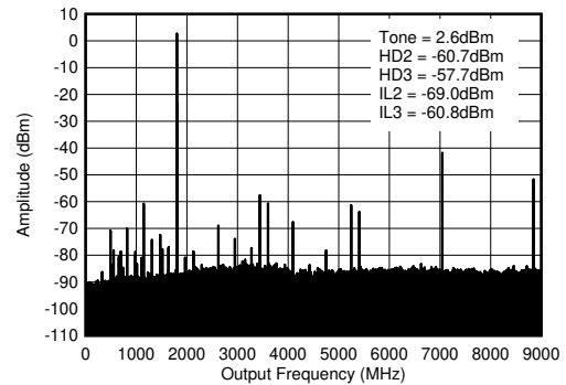
图 7-75. 1.8GHz (0 - f_{\text{DAC}} ) 条件下的 TX 单频 (-12dBFS) 输出频谱
