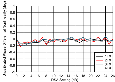
图 7-240. TX DSA 未校准相位微分非线性
