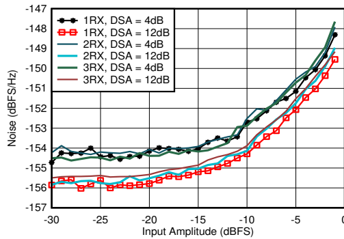
图 7-292. 0.8GHz 条件下 RX 噪声频谱密度与输入振幅和通道间的关系
