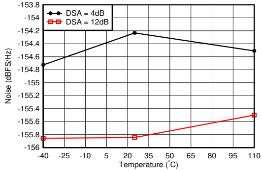
图 7-290. 0.8GHz 条件下 RX 噪声频谱密度与温度间的关系
