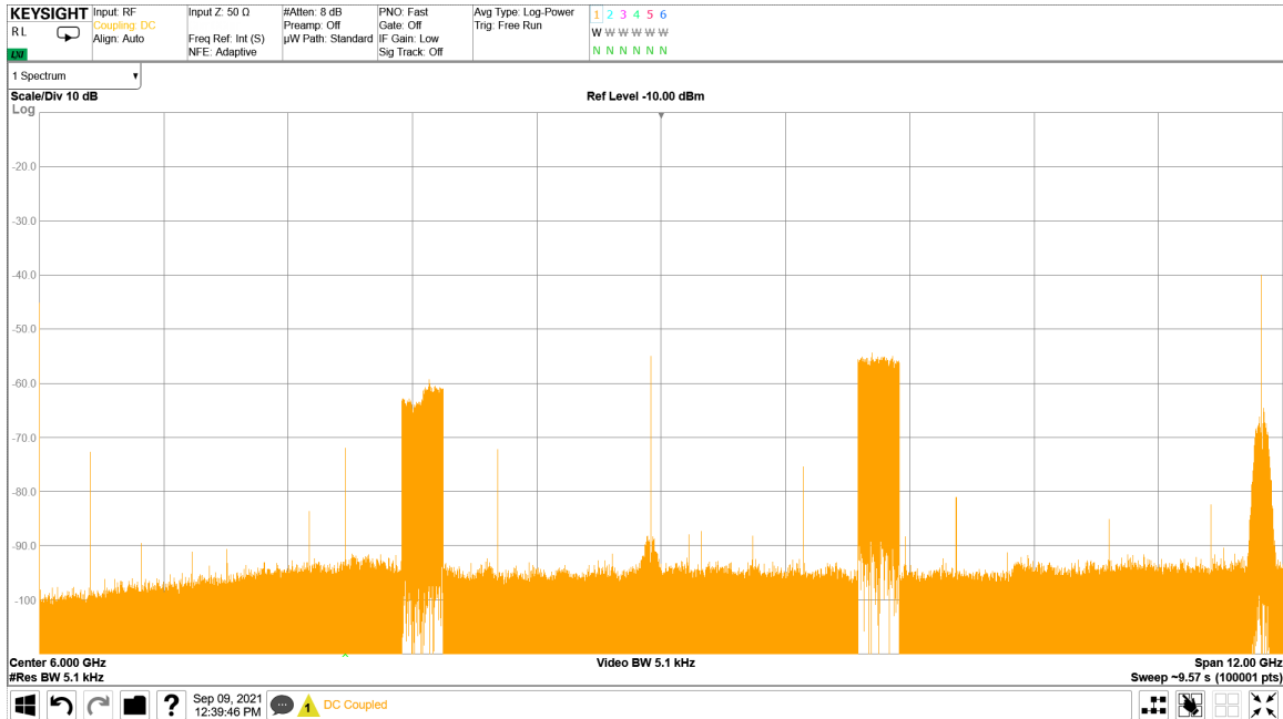
图 7-228. 8.11GHz 条件下 TX 4x100MHz NR 输出频谱
