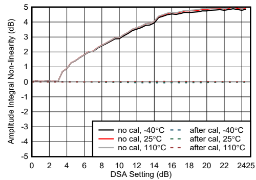
图 7-447. 9.6GHz 条件下 RX 振幅积分非线性
