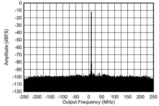
图 7-465. 9.61GHz 条件下 RX 单音输出 FFT
