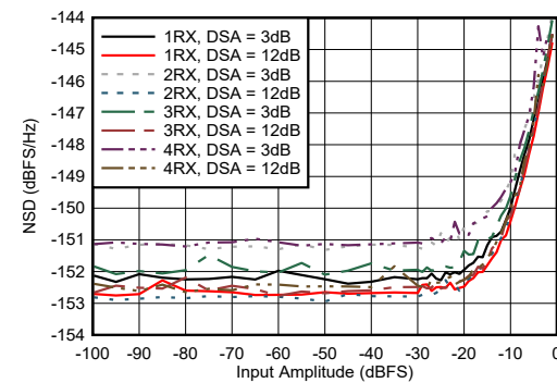
图 7-426. 8.11GHz 条件下 RX NSD 与数字振幅间的关系
