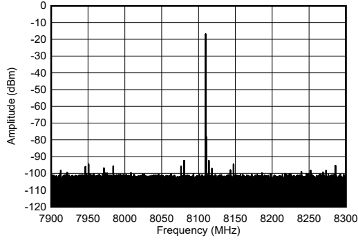
图 7-208. 8.11GHz 条件下 TX 单音输出频谱
