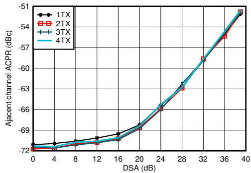
图 7-104. 2.6GHz 条件下 TX 20MHz LTE ACPR 与数字电平间的关系
