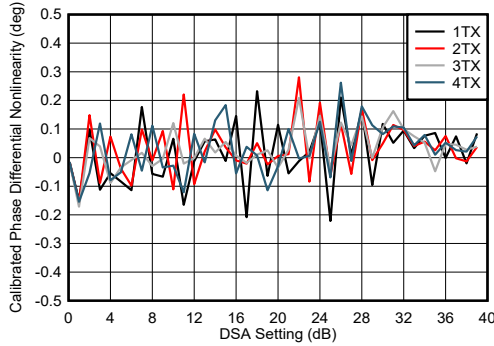
图 7-196. 8.1GHz 条件下 TX DSA 校准相位微分非线性
