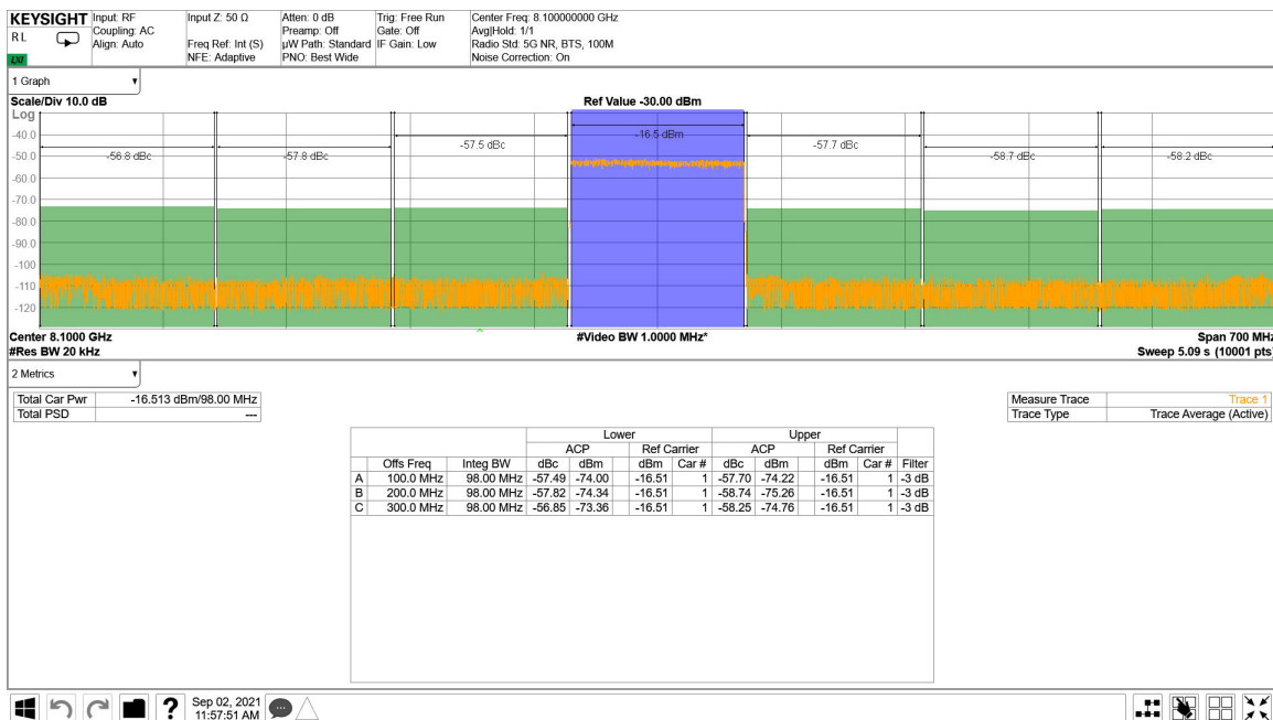
图 7-225. 8.1GHz 条件下 TX 100MHz NR 输出频谱
