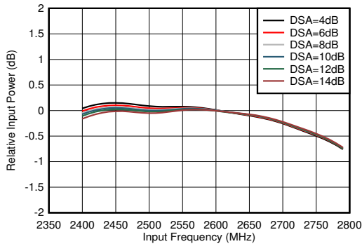
图 7-339. RX 带内增益平坦度， f_{\text{IN}} = 2600\text{MHz}
