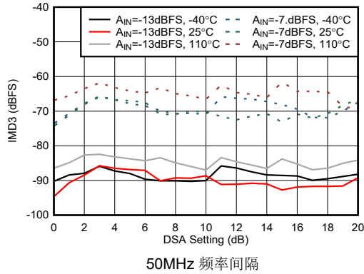
图 7-452. 9.6 GHz 条件下 RX IMD3 与 DSA 设置间的关系
