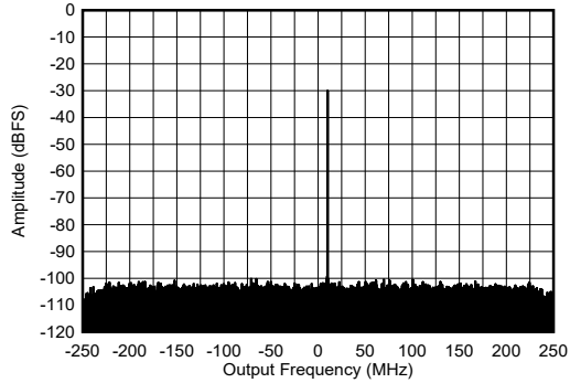
图 7-464. 9.61GHz 条件下 RX 单音输出 FFT
