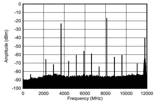
图 7-205. 8.1GHz 条件下 TX 单音输出频谱
