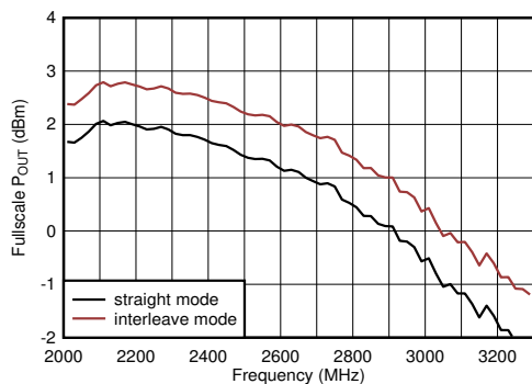
图 7-78. 11796.48MSPS 条件下 TX 满量程与射频频率间的关系
