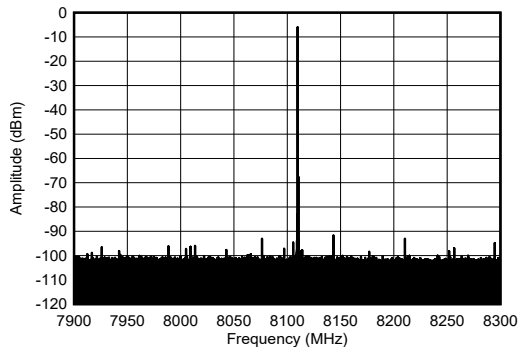
图 7-204. 8.1GHz 条件下 TX 单音输出频谱
