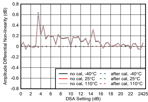
图 7-446. 9.6GHz 条件下 RX 振幅微分非线性
