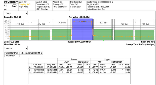
图 7-103. 2.6GHz (频带 41) 条件下的 TX 20MHz LTE 输出频谱
