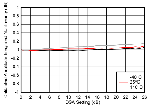
图 7-239. TX DSA 校准振幅积分非线性
