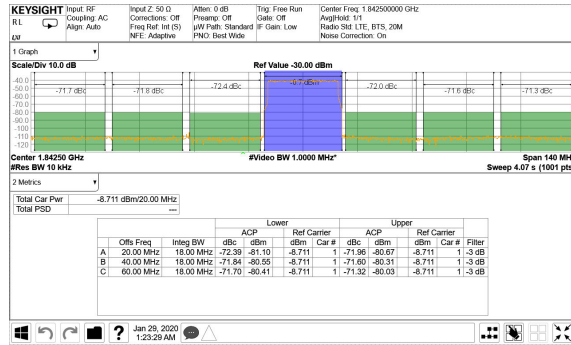
图 4-68. TX 20-MHz LTE Output Spectrum at 1.8425GHz
