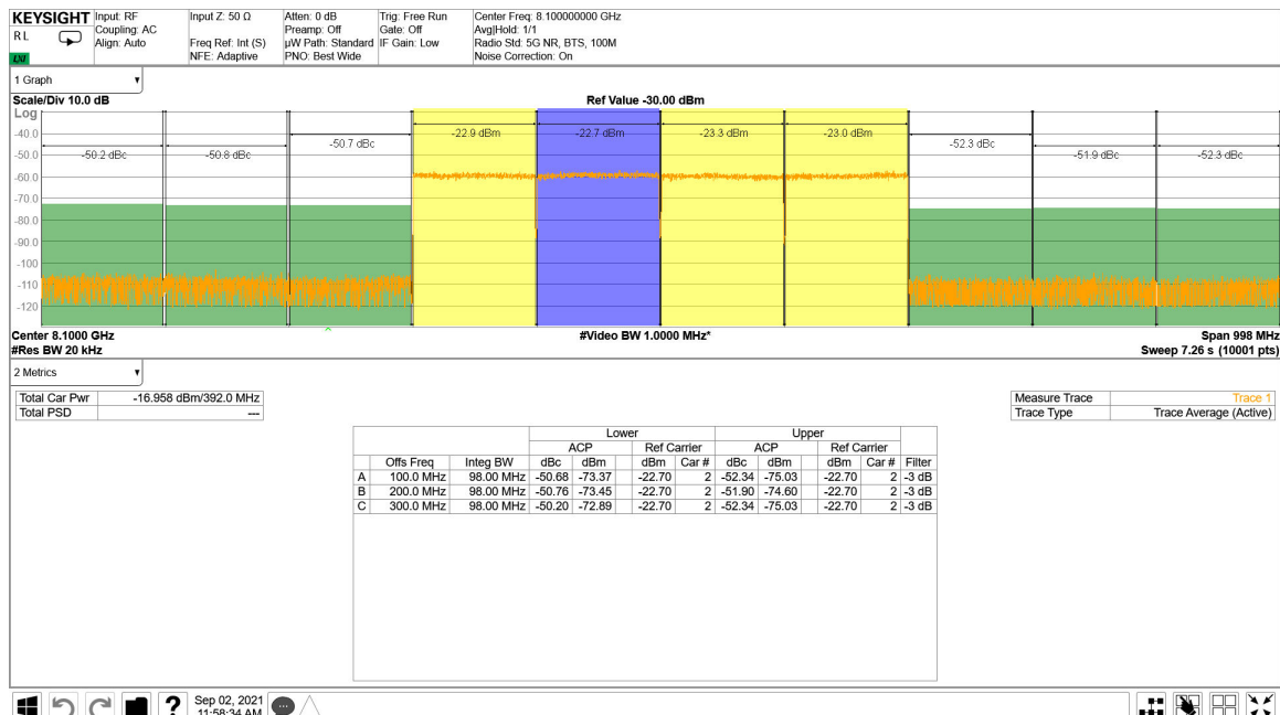
图 4-231. TX 4x100MHz NR Output Spectrum 8.1GHz
