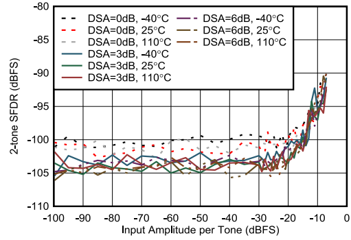
图 5-231. 6.85GHz 条件下 RX 2 子载波 SFDR 与输入振幅间的关系 100MHz 子载波间隔，不包括三阶失真
