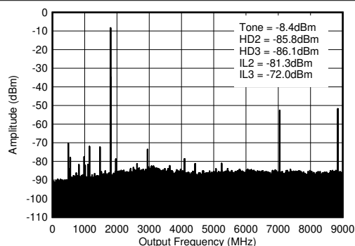
图 5-376. 1.8GHz ( 0 - f_{\text{DAC}} ) 条件下的 TX 单音 ( -1\text{dBFS} ) 输出频谱
