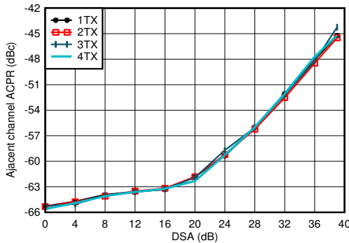
图 5-420. 2.6GHz 条件下 TX 100MHz NR ACPR 与 DSA 间的关系
