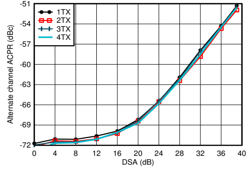
图 5-419. 2.6GHz 条件下 TX 20MHz LTE alt-ACPR 与 DSA 间的关系
