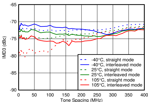
图 5-408. 2.6GHz 条件下 TX IMD3 与频率间隔和温度间的关系
