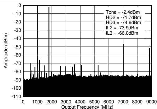
图 5-378. 1.8GHz ( 0 - f_{\text{DAC}} ) 条件下的 TX 单音 ( -12\text{dBFS} ) 输出频谱
