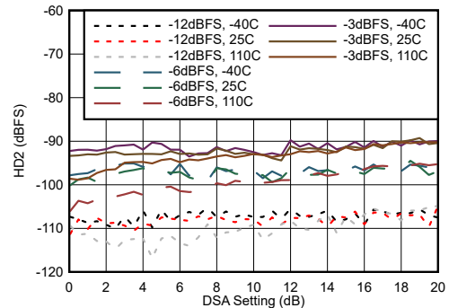
图 5-26. 30MHz 条件下 HD2 与 DSA 设置间的关系
