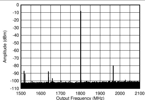
图 5-377. 1.8GHz ( \pm 300\text{MHz} ) 条件下的 TX 单音 ( -1\text{dBFS} ) 输出频谱
