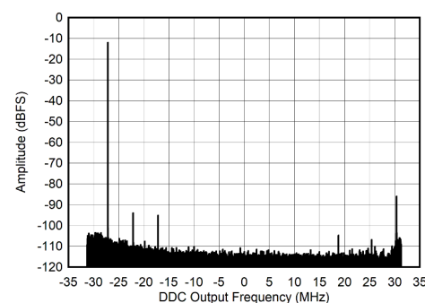
图 5-10. 5MHz 条件下的 RX 输出 FFT
