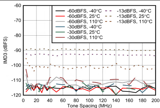
图 5-123. 2.6GHz (外部时钟) 条件下 RX IMD3 与子载波间隔间的关系
