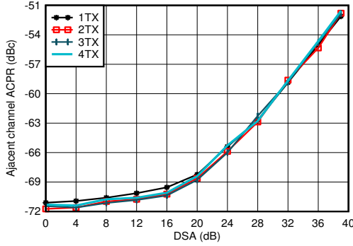
图 5-418. 2.6GHz 条件下 TX 20MHz LTE ACPR 与 DSA 间的关系
