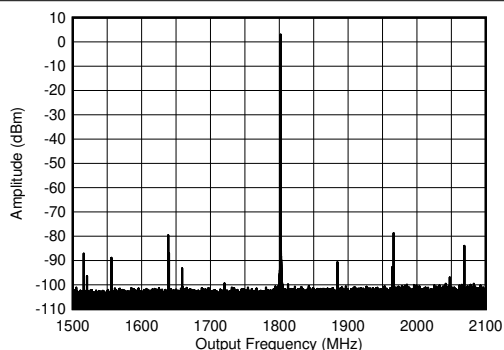
图 5-375. 1.8GHz ( \pm 300\text{MHz} ) 条件下的 TX 单音 ( -6\text{dBFS} ) 输出频谱
