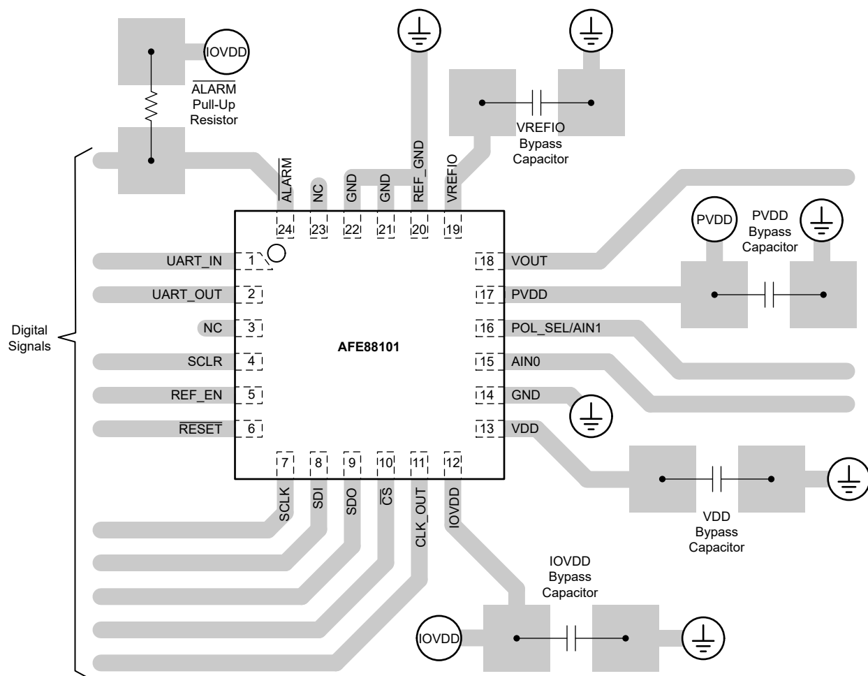
图 8-8. Layout Example
