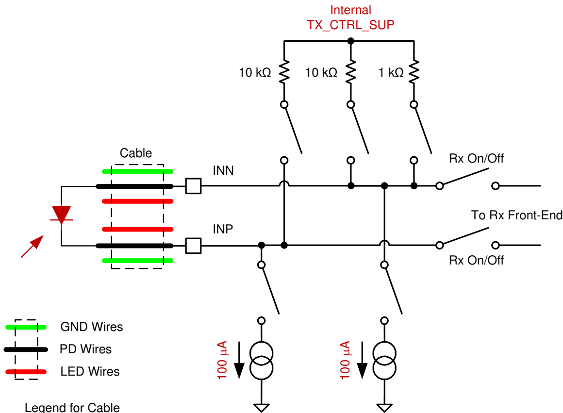
图 8-31. Photodiode Diagnostic
