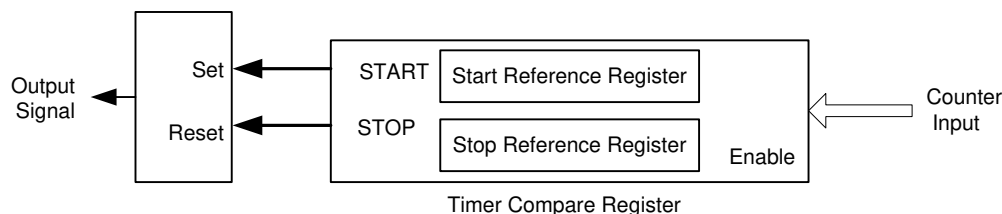
图 8-11. Compare Register
