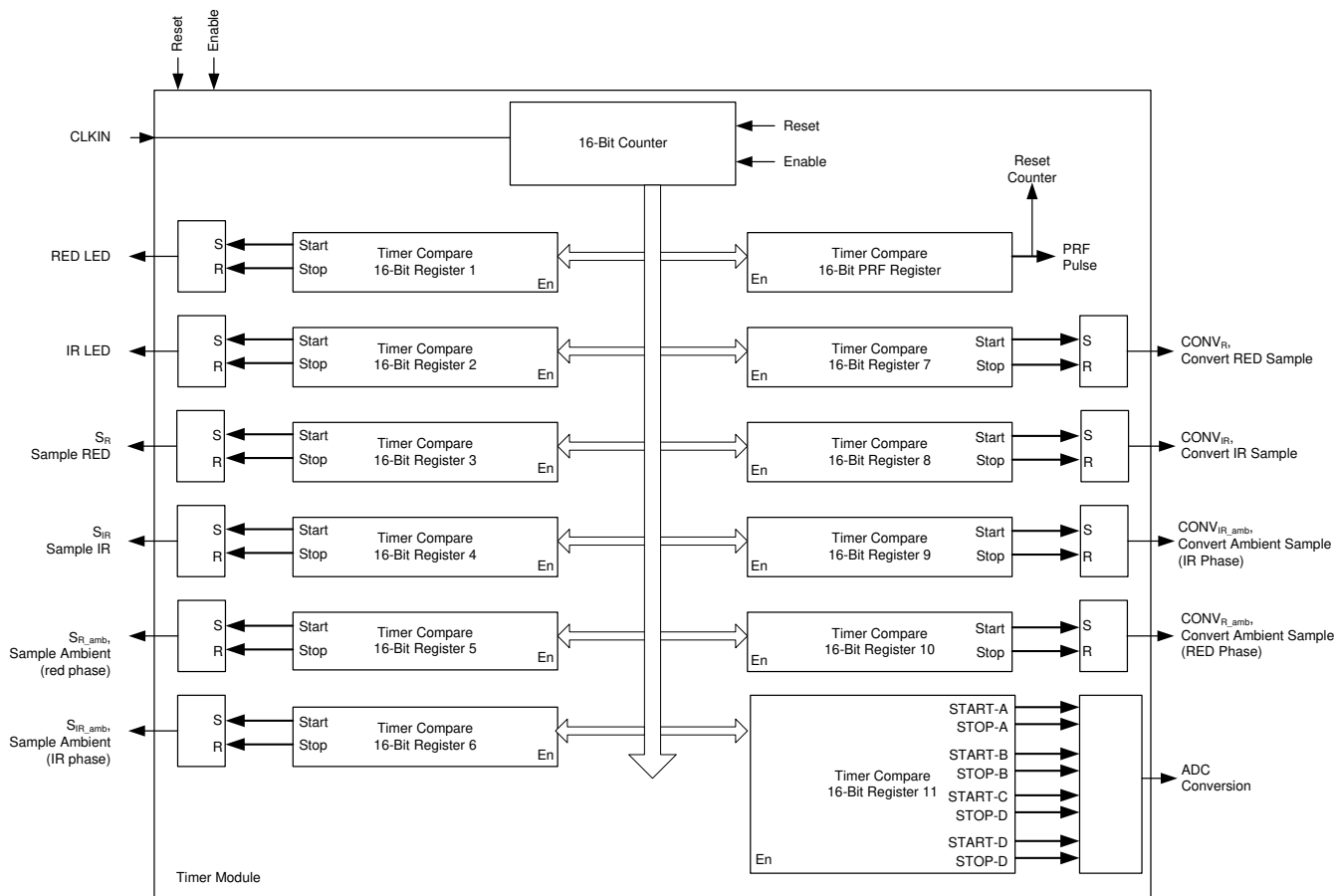
图 8-12. Timer Module
