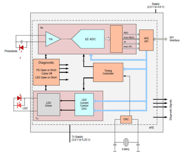
方框图
