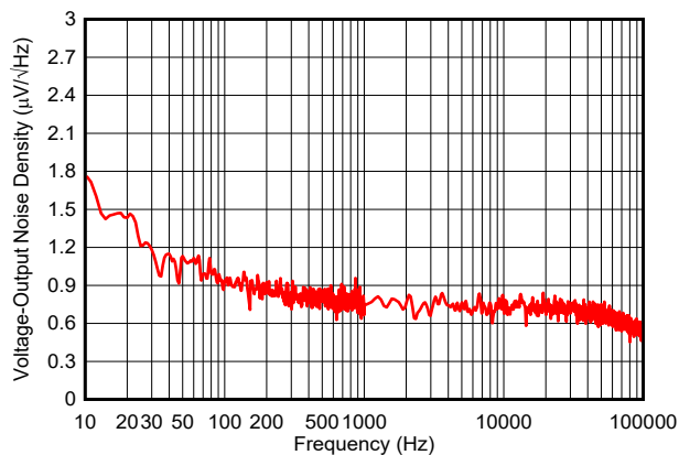
图 5-25. 电压输出噪声密度
