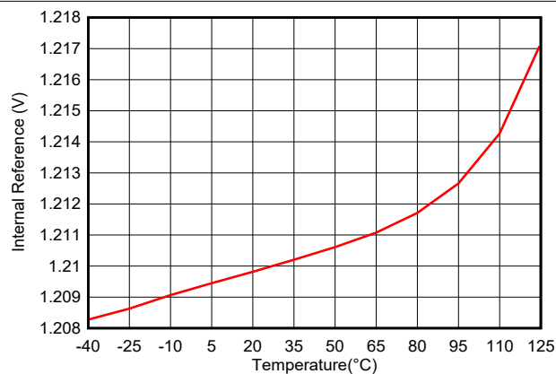
图 5-59. 内部基准与温度间的关系
