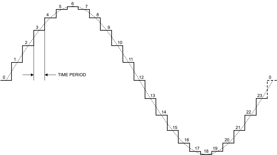
图 6-13. 正弦波生成
