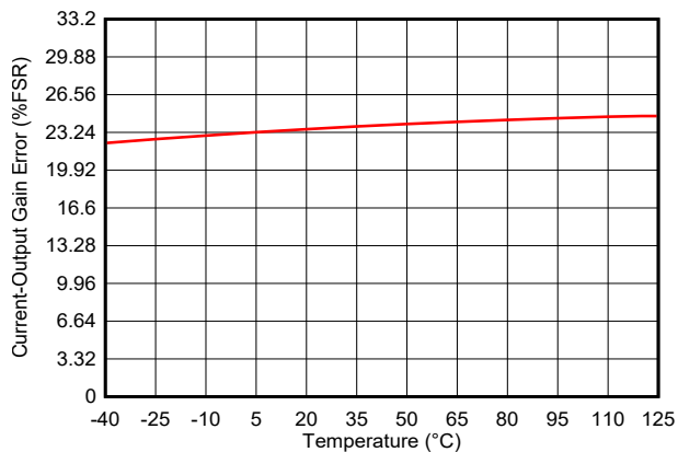
图 5-36. 电流输出增益误差与温度间的关系
