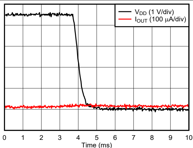
图 5-43. 电流输出断电干扰
