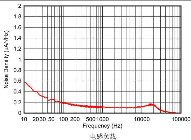
图 5-45. 电流输出噪声密度
