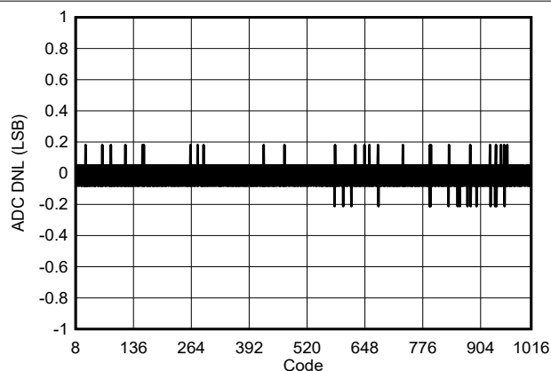
图 5-55. ADC DNL 与数字输出代码间的关系
