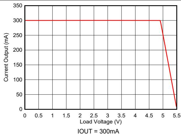
图 5-37. 电流输出与负载电压间的关系
