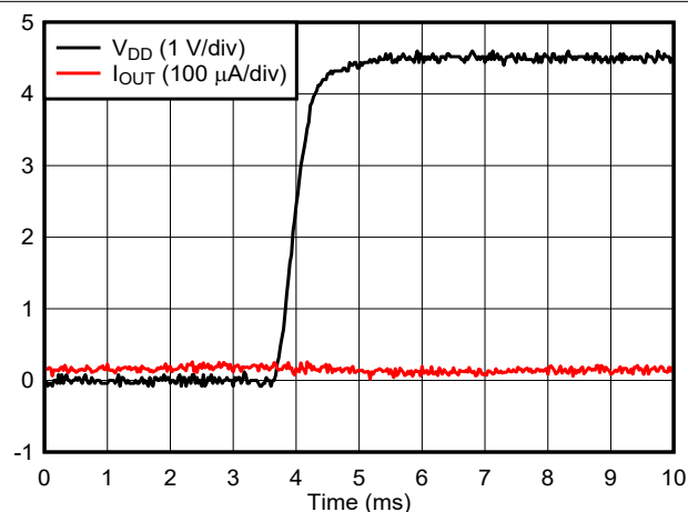
图 5-42. 电流输出上电干扰
