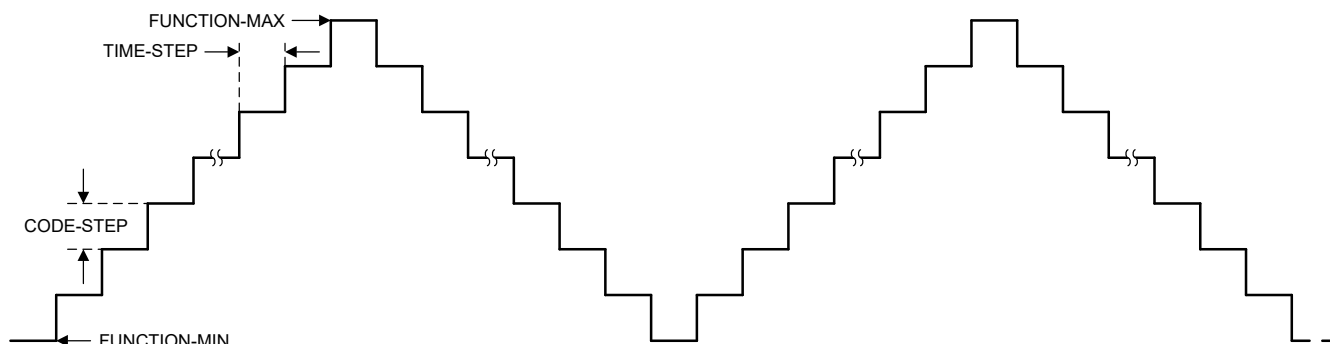
图 6-11. 三角波形
