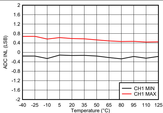
图 5-54. ADC INL 与温度间的关系
