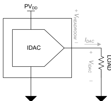
图 8-2. IDAC 功率耗散
