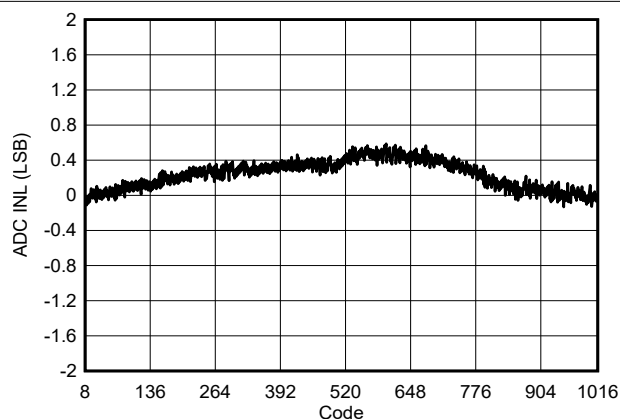
图 5-53. ADC INL 与数字输出代码间的关系
