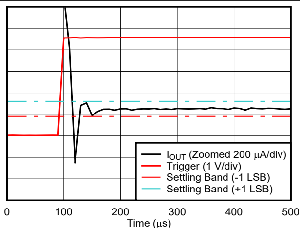
图 5-41. 电流输出建立时间（下降沿）
