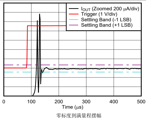
图 5-40. 电流输出建立时间（上升沿）
