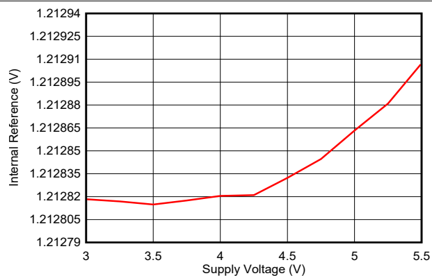
图 5-60. 内部基准与电源电压间的关系
