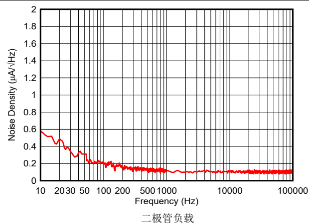
图 5-44. 电流输出噪声密度
