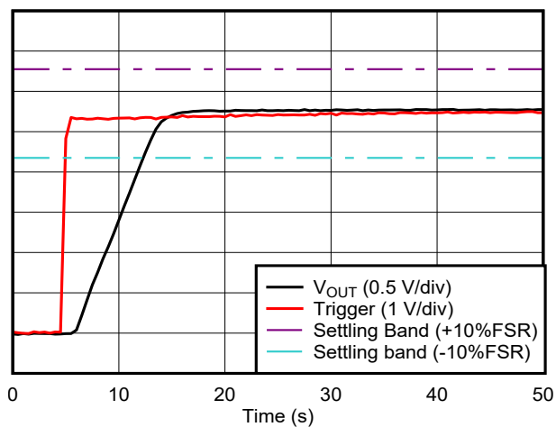
图 5-21. 电压输出建立时间 - 上升沿
