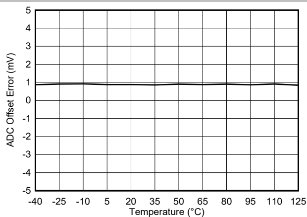
图 5-57. ADC 偏移误差与温度间的关系
