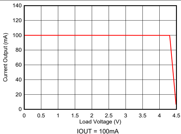
图 5-38. 电流输出与负载电压间的关系
