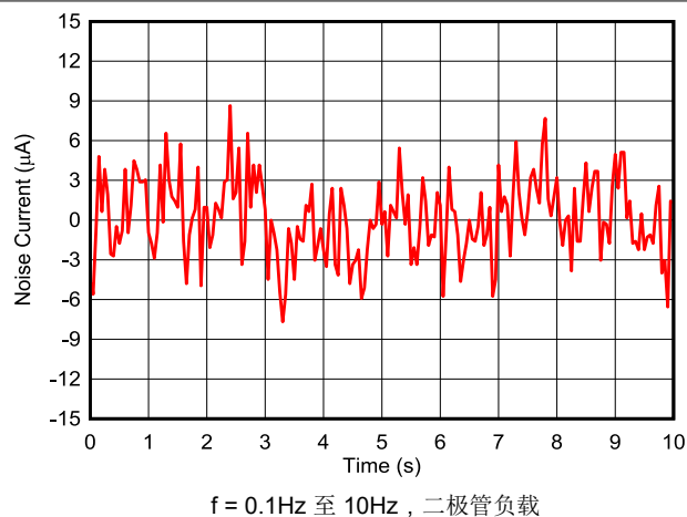
图 5-46. 电流输出闪烁噪声
