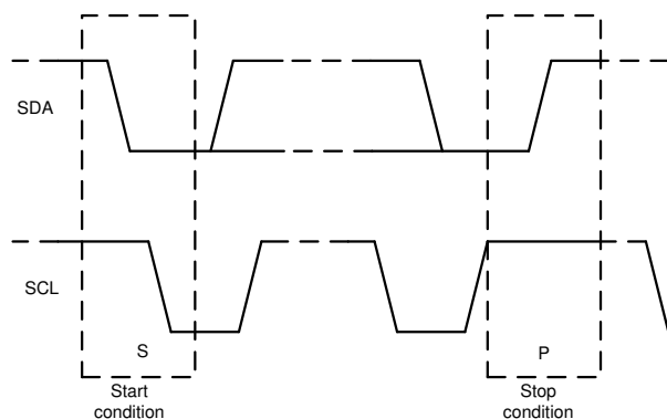
图 6-20. 启动和停止条件
