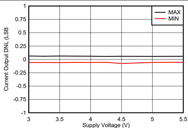
图 5-34. 电流输出 DNL 与电源电压间的关系
