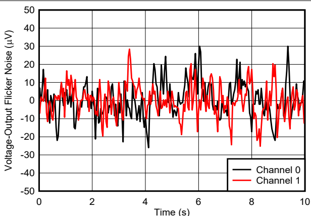
图 5-27. 电压输出闪烁噪声
