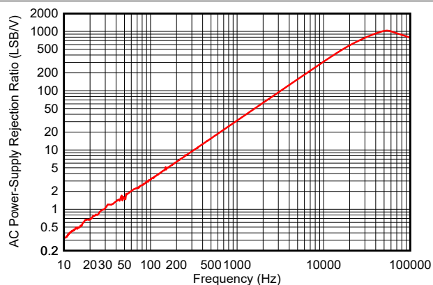
图 5-48. 电流输出交流 PSRR 与频率间的关系
