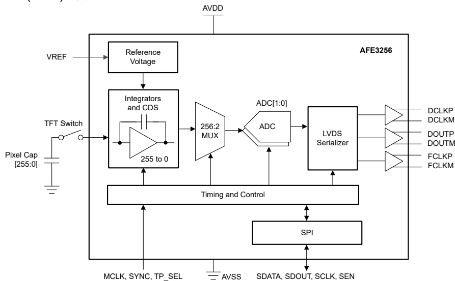
AFE3256 方框图
