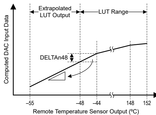
图 6-12. 远程温度传感器输出
