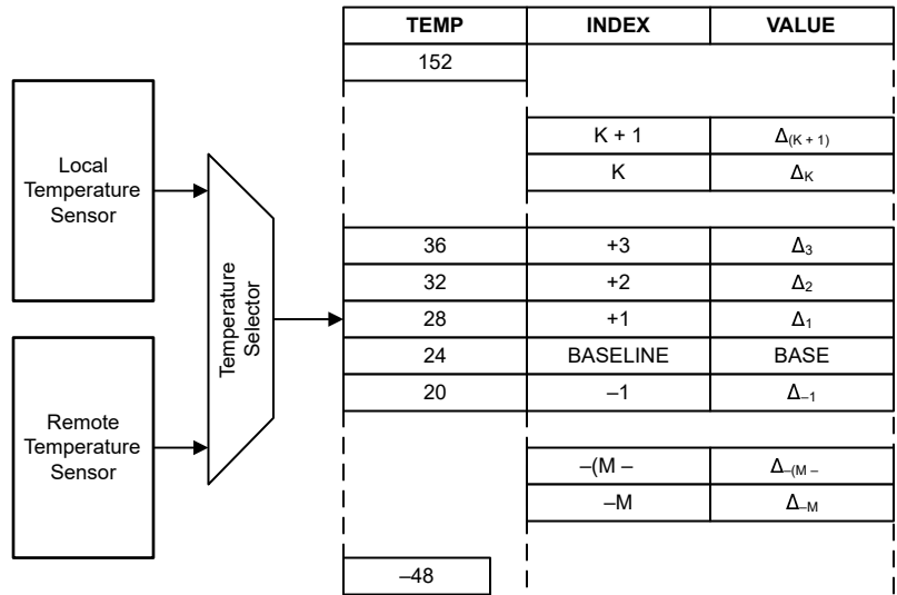
图 6-9. LUT 组织
