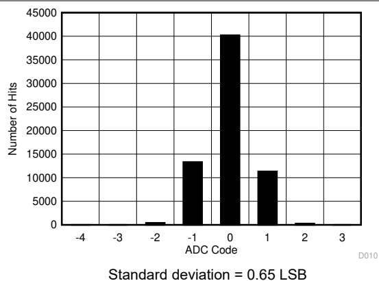
图 6-12. DC Input Histogram
