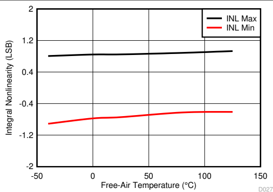
图 6-18. Typical INL ADC B
