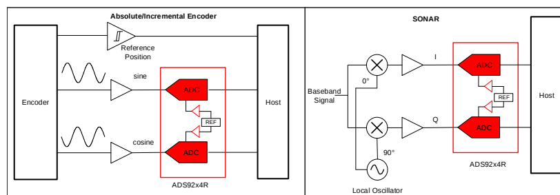
典型应用图
