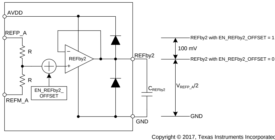
图 40. REFby2 Buffer
