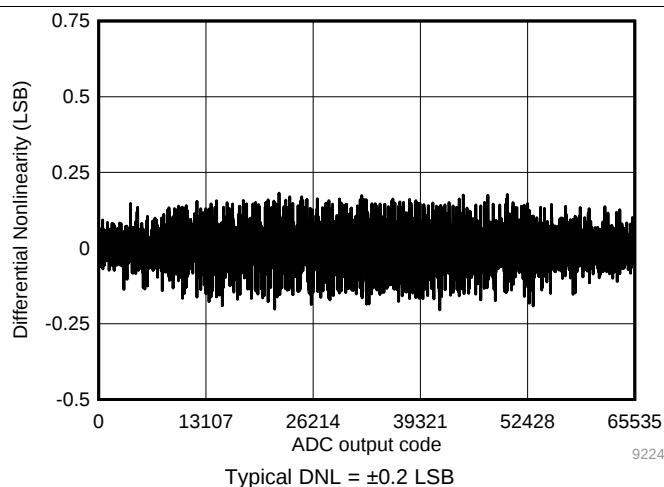
图 16. Typical DNL
