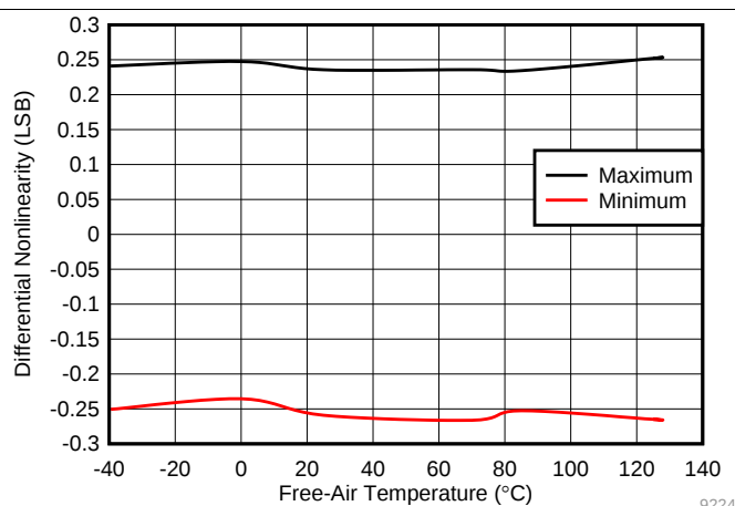
图 16. Typical DNL
