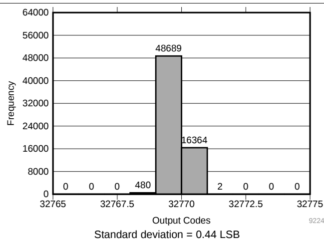
图 15. DC Input Histogram
