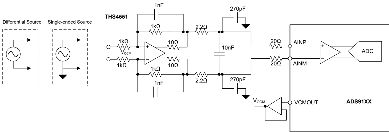
图 8-1. \leq 20\text{kHz} 的输入信号带宽的数据采集 (DAQ) 电路
