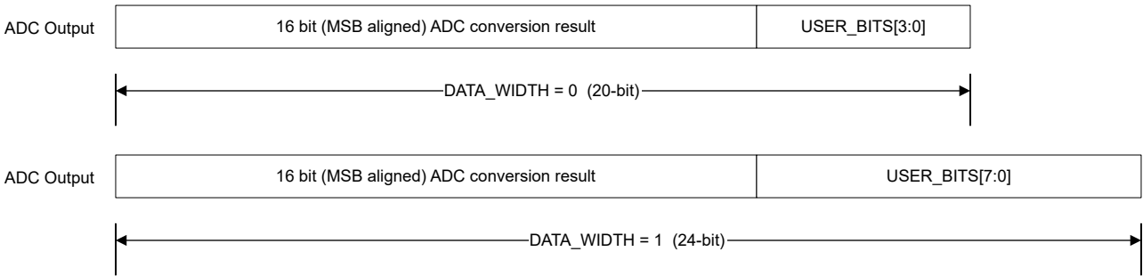
图 6-6. 数据帧宽度组成
