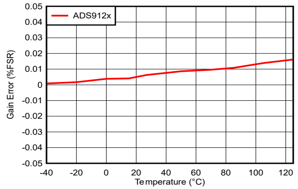
图 5-8. 增益误差与温度间的关系
