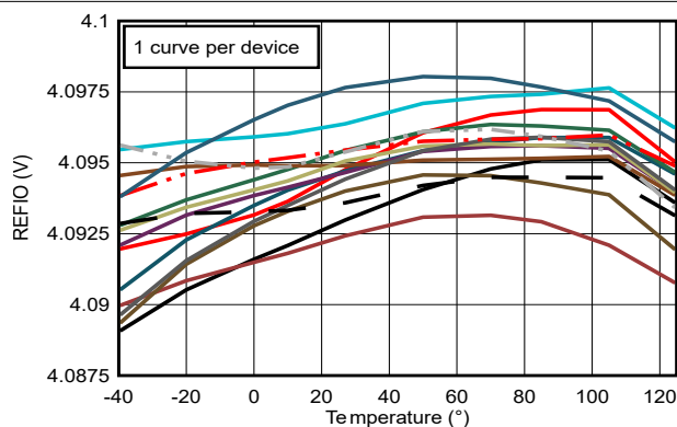
图 5-13. REFIO 电压与温度间的关系
