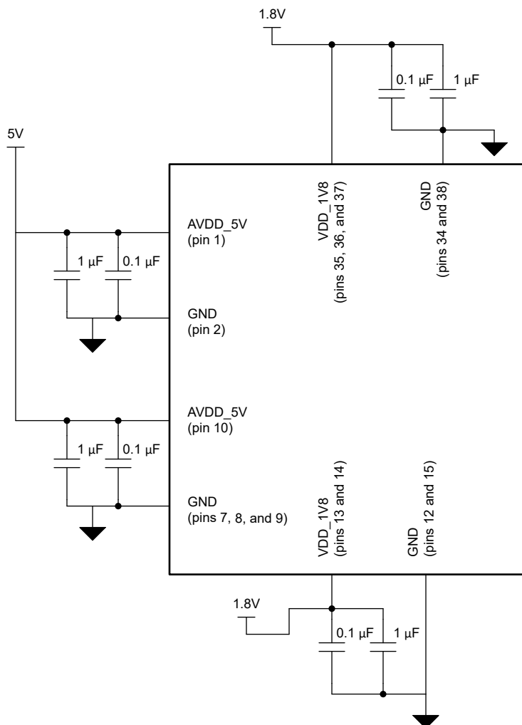
图 8-10. 电源去耦
