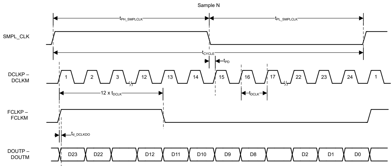
图 5-2. LVDS 数据接口：SDR
