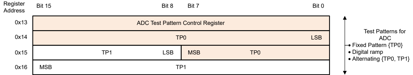
图 6-7. 用于测试图形的寄存器组
