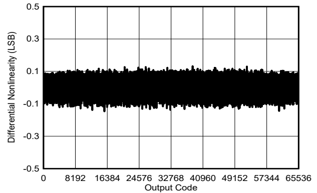
图 5-18. 典型 DNL：ADS9129
