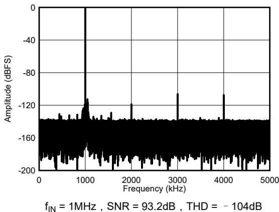
图 8-8. 10MSPS 时的典型 FFT : ADS9128
