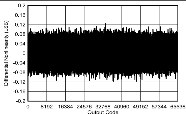
图 5-23. 典型 DNL
