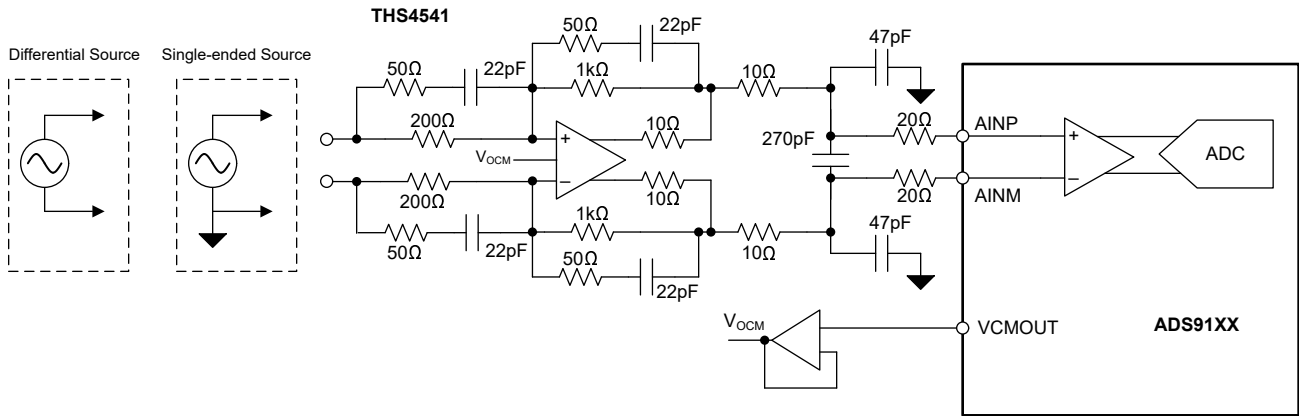
图 8-7. \leq 1\text{MHz} 的输入信号带宽的数据采集 (DAQ) 电路
