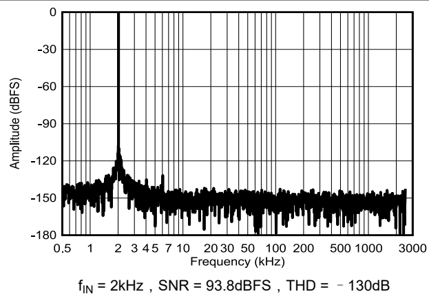
图 8-2. 5MSPS 时的典型 FFT : ADS9127
