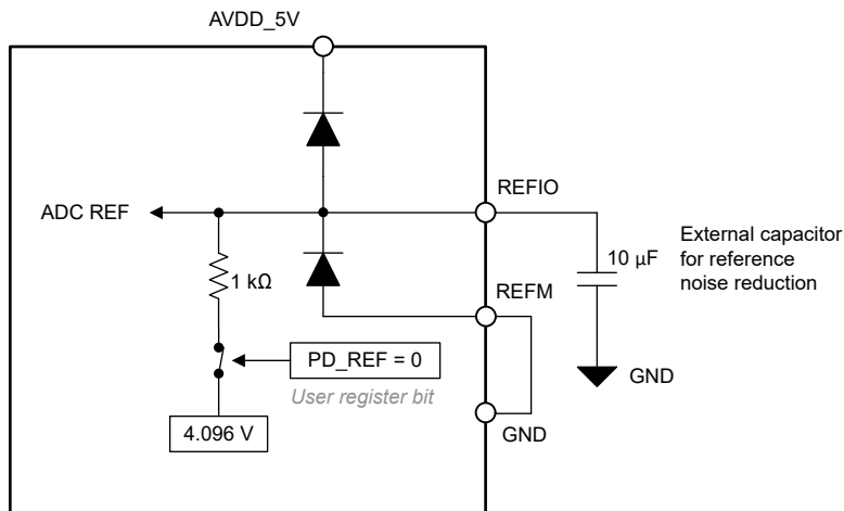
图 6-2. 内部基准电压
