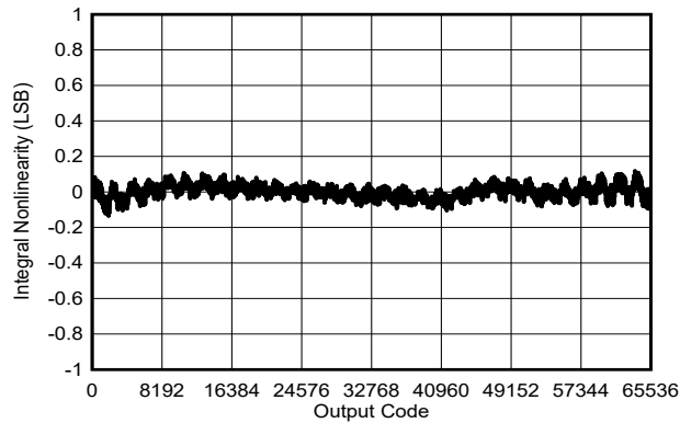
图 5-17. 典型 INL
