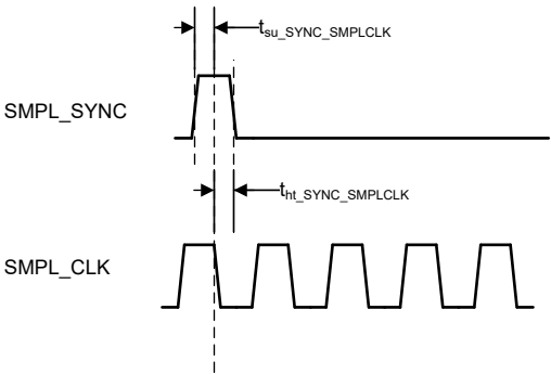
图 5-5. SMPL_SYNC 时序
