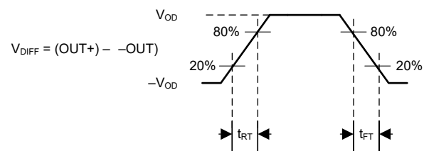
图 5-3. LVDS 输出转换次数
