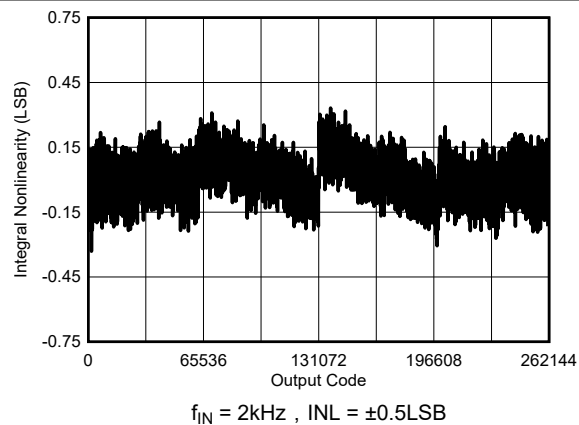
图 8-3. 5MSPS 时的典型 INL : ADS9127
