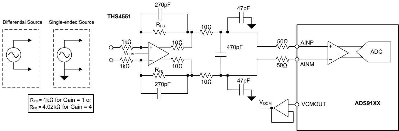
图 8-4. \leq 100\text{kHz} 的输入信号带宽的数据采集 (DAQ) 电路
