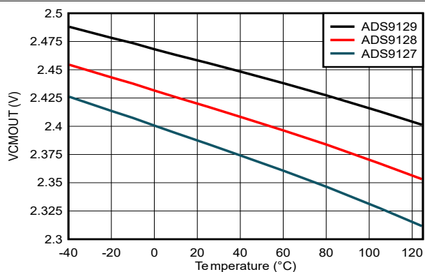
图 5-14. V_{CMOUT} 电压与温度间的关系
