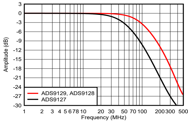
图 5-7. 典型模拟输入带宽
