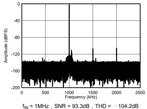
图 8-9. 5MSPS 时的典型 FFT : ADS9127
