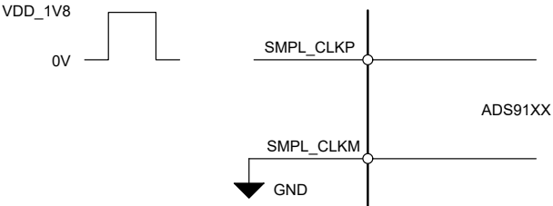
图 6-9. 单端采样时钟
