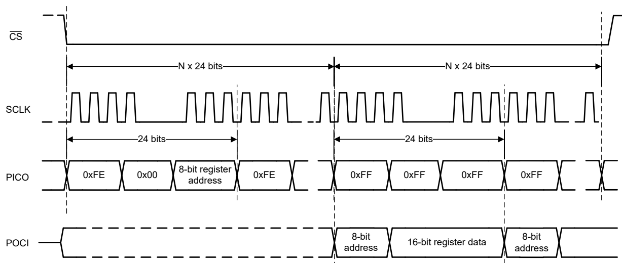
图 6-15. 菊花链配置中的寄存器读取
