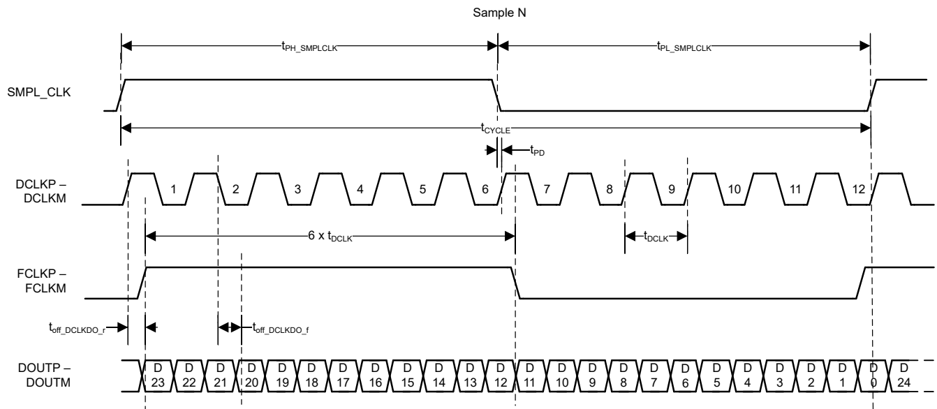
图 5-1. LVDS 数据接口：DDR
