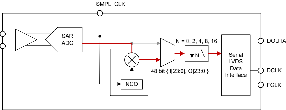
图 6-5. 使用数字下变频器时的数据路径
