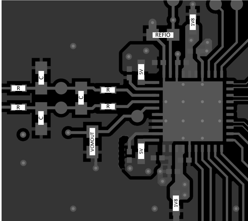
图 8-11. 示例布局
