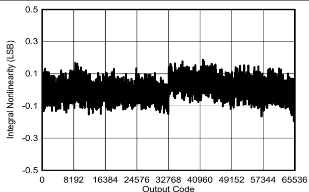
图 5-22. 典型 INL
