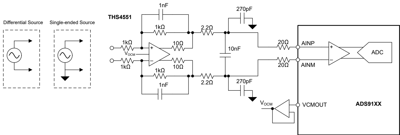
图 8-1. ≤20kHz 的输入信号带宽的数据采集 (DAQ) 电路
