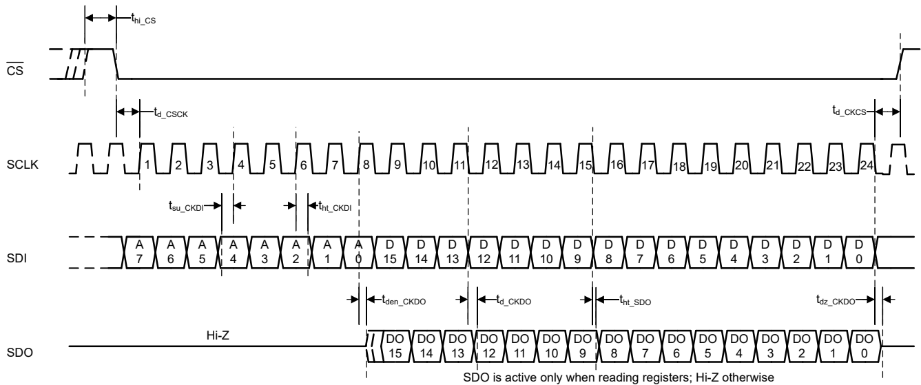
图 5-4. 配置 SPI
