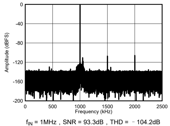
图 8-9. 5MSPS 时的典型 FFT : ADS9127
