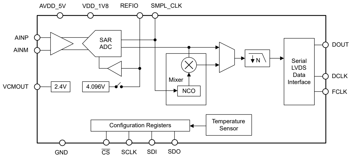
器件方框图
