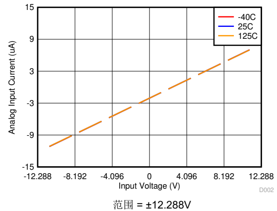
图 5-10. 整个温度范围内的输入 I-V 特性
