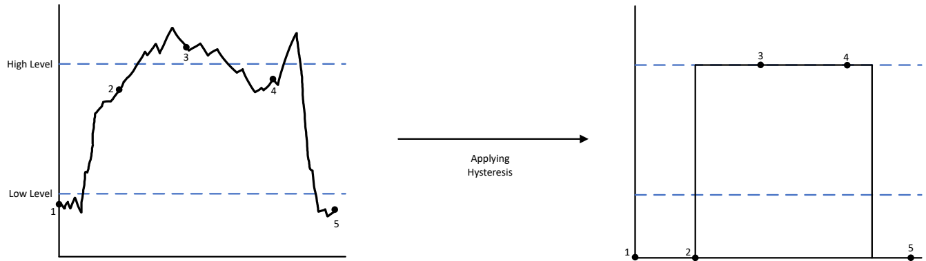
图 8-4. 带迟滞的警报功能
