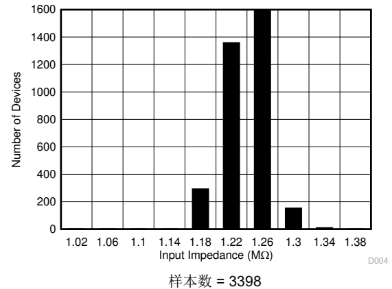
图 5-12. 输入阻抗的典型分布
