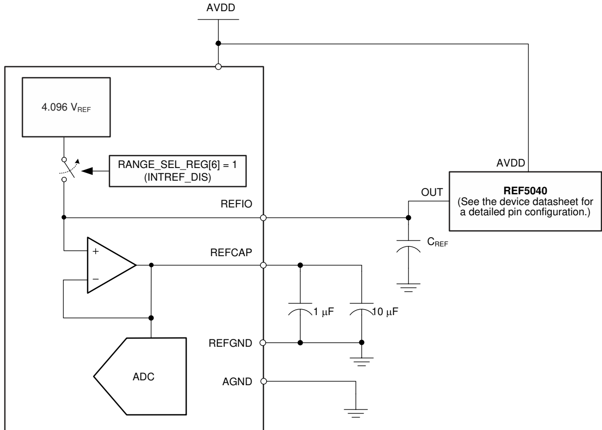
在 REFCAP 引脚上获取内部基准缓冲器的输出。在 REFCAP 引脚和 REFGND 引脚之间放置一个最小 10\ \mu\text{F} 的电容。在尽可能靠近 REFCAP 引脚的位置放置另一个 1\ \mu\text{F} 电容器，用于对高频信号去耦。请勿使用内部缓冲器来驱动外部交流或直流负载，因为此缓冲器的电流输出能力有限。
