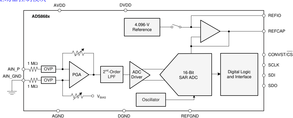
方框图
