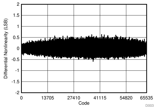
图 6-14. Typical DNL
