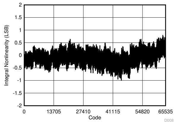
图 6-15. Typical INL
